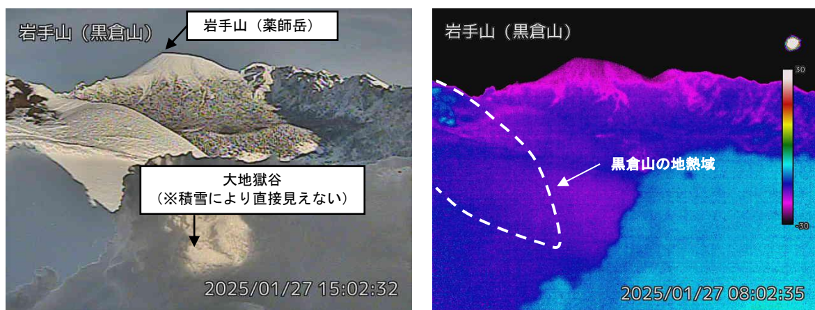
図1 岩手山 黒倉山監視カメラからの状況と地表面温度分布（1月27日）
