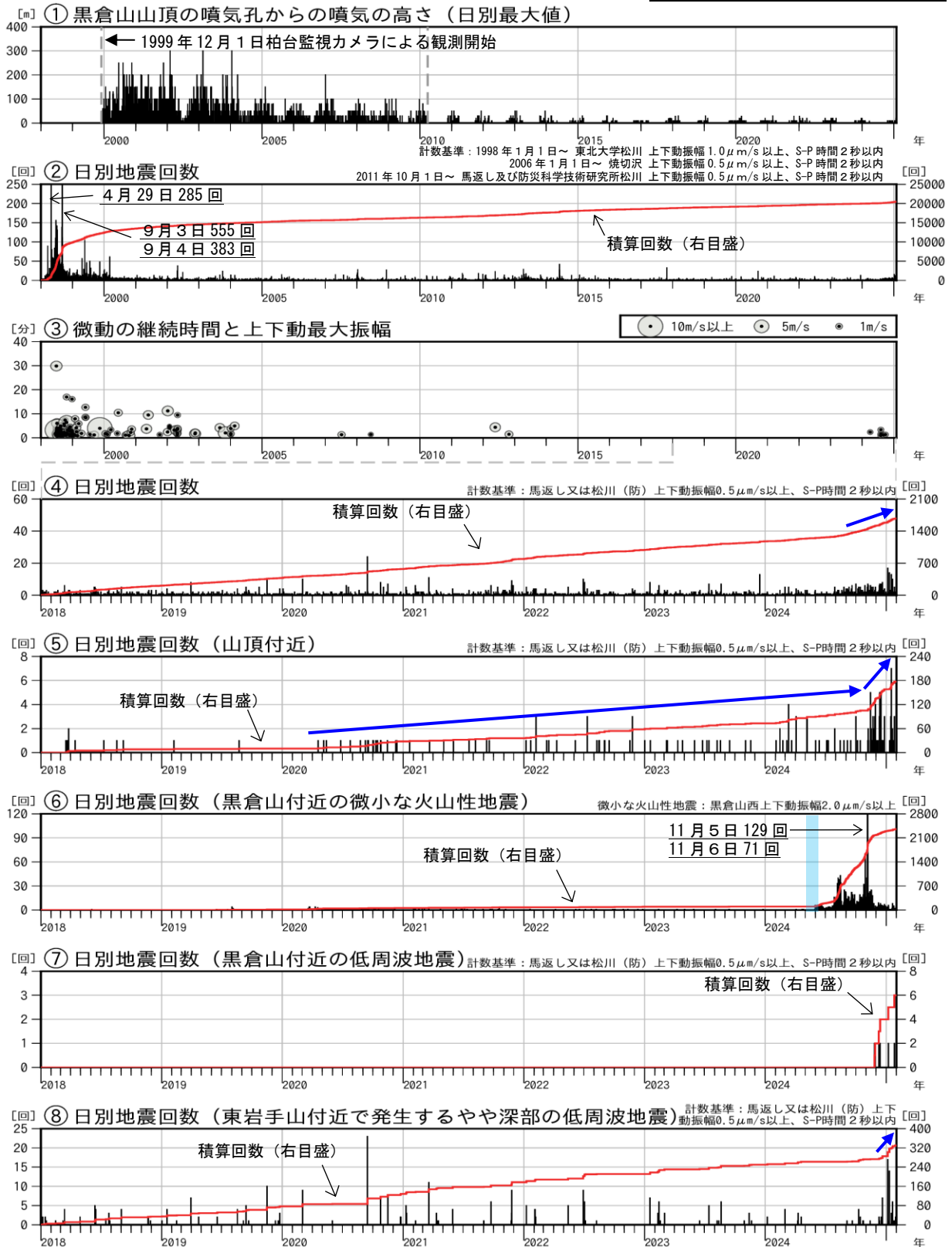
図3 岩手山 火山活動経過図（1998年1月～2025年1月）
