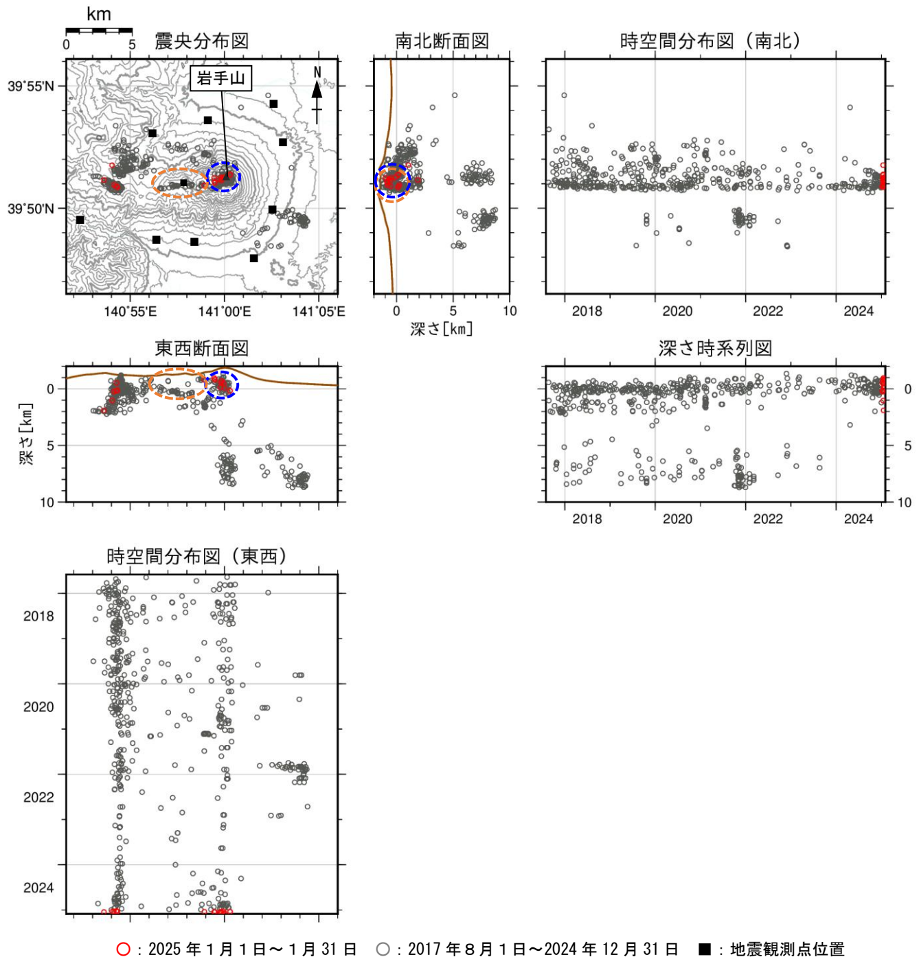
図4 岩手山 地震活動（2017年8月～2025年1月）
