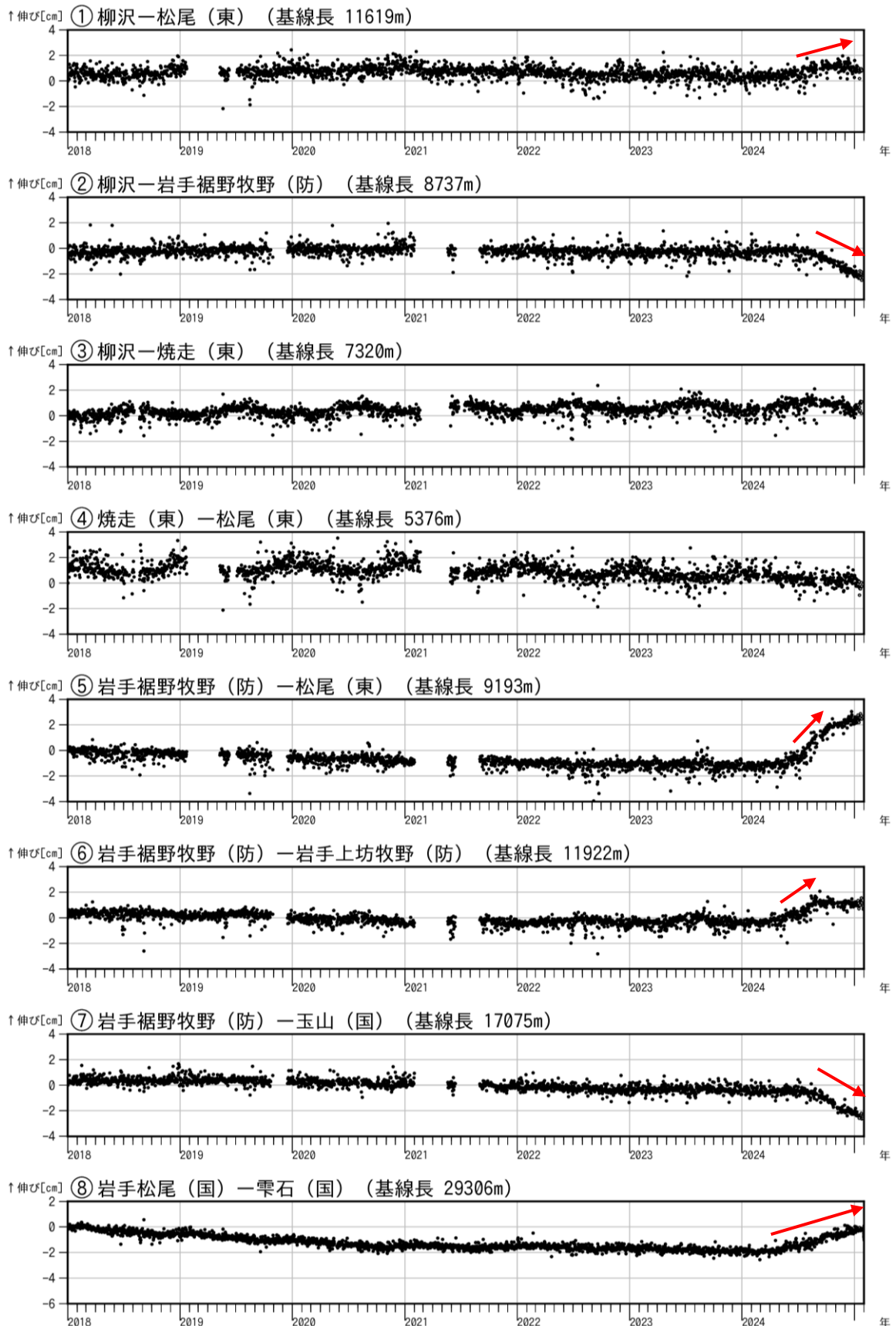
図5 岩手山 GNSS 基線長変化図（2018 年 1 月～2025 年 1 月）
