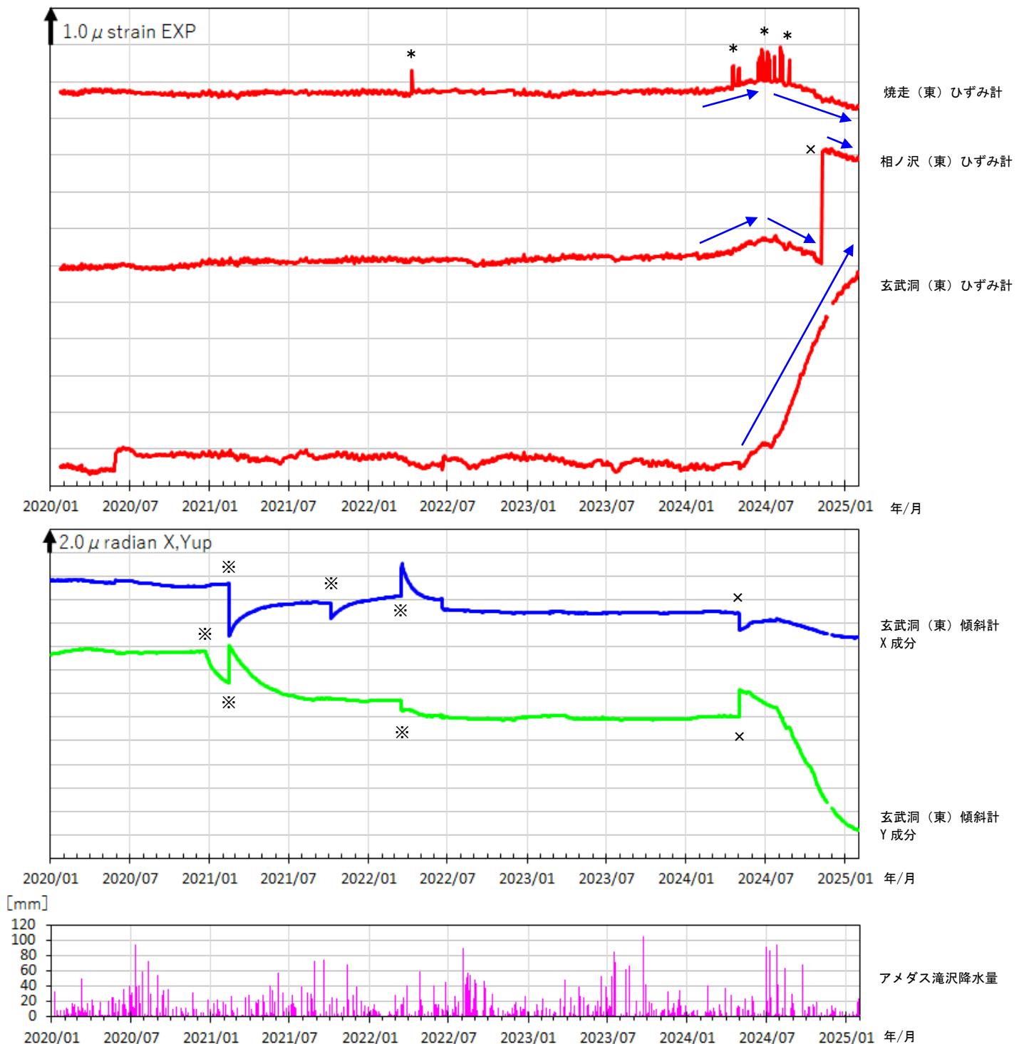
図6 岩手山 ひずみ計・傾斜計（日値・トレンド補正済み）による地殻変動の状況 （2020年1月～2025年1月）
