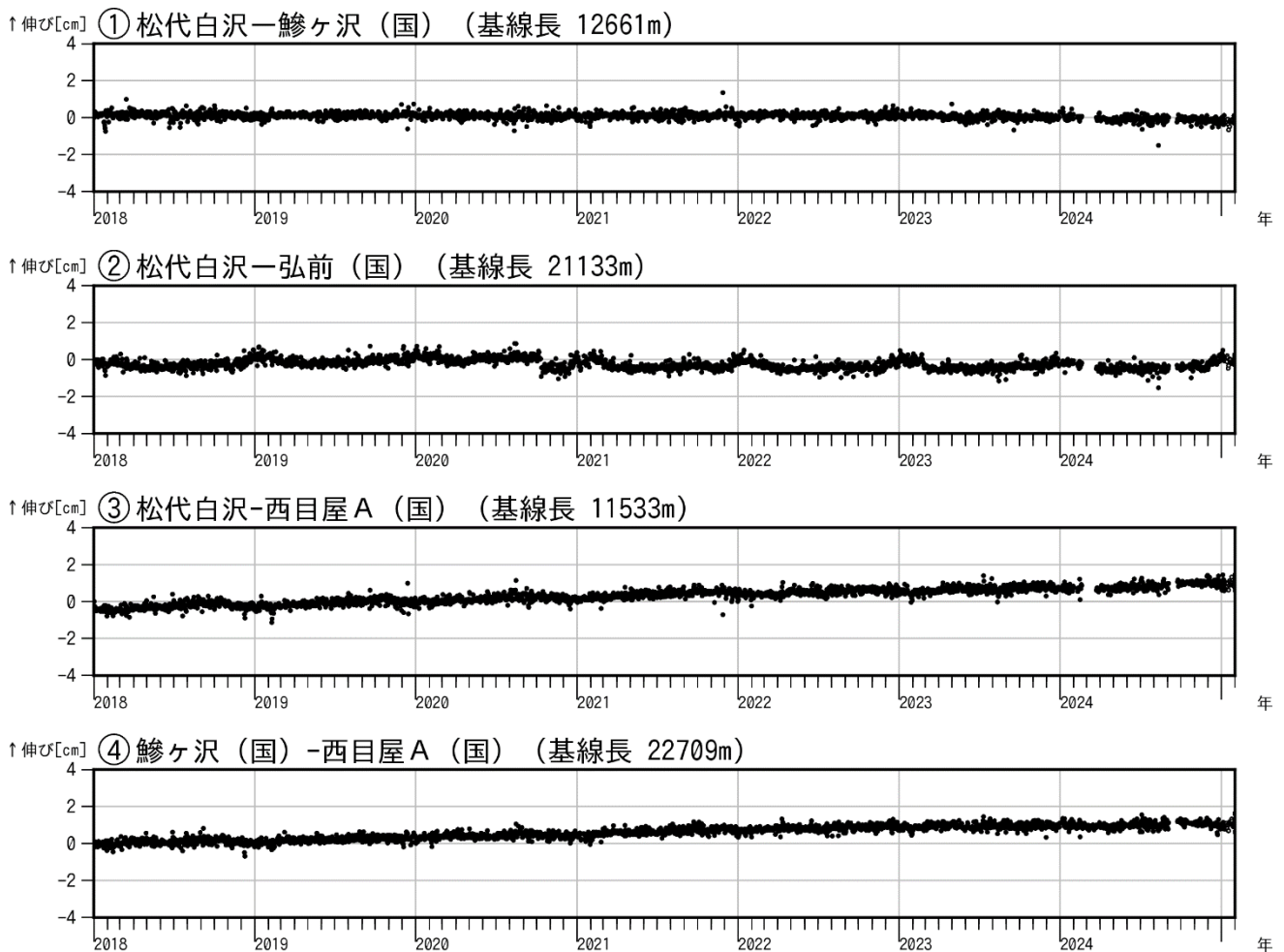
図3 岩木山 GNSS 基線長変化図（2018年1月～2025年1月）
