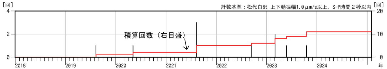
図2 岩木山 日別地震回数（2018年1月～2025年1月）
