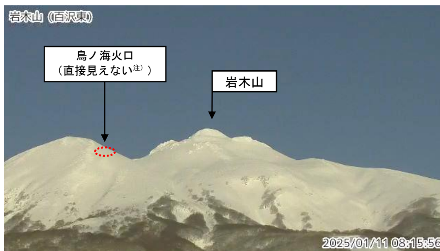
図1 岩木山 山頂部の状況（1月11日）
