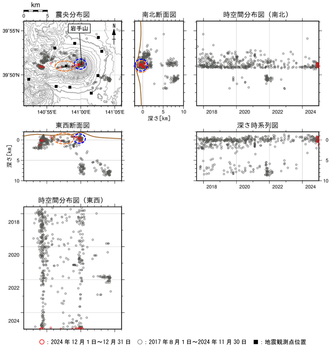
図4 岩手山 地震活動（2017年8月～2024年12月）
