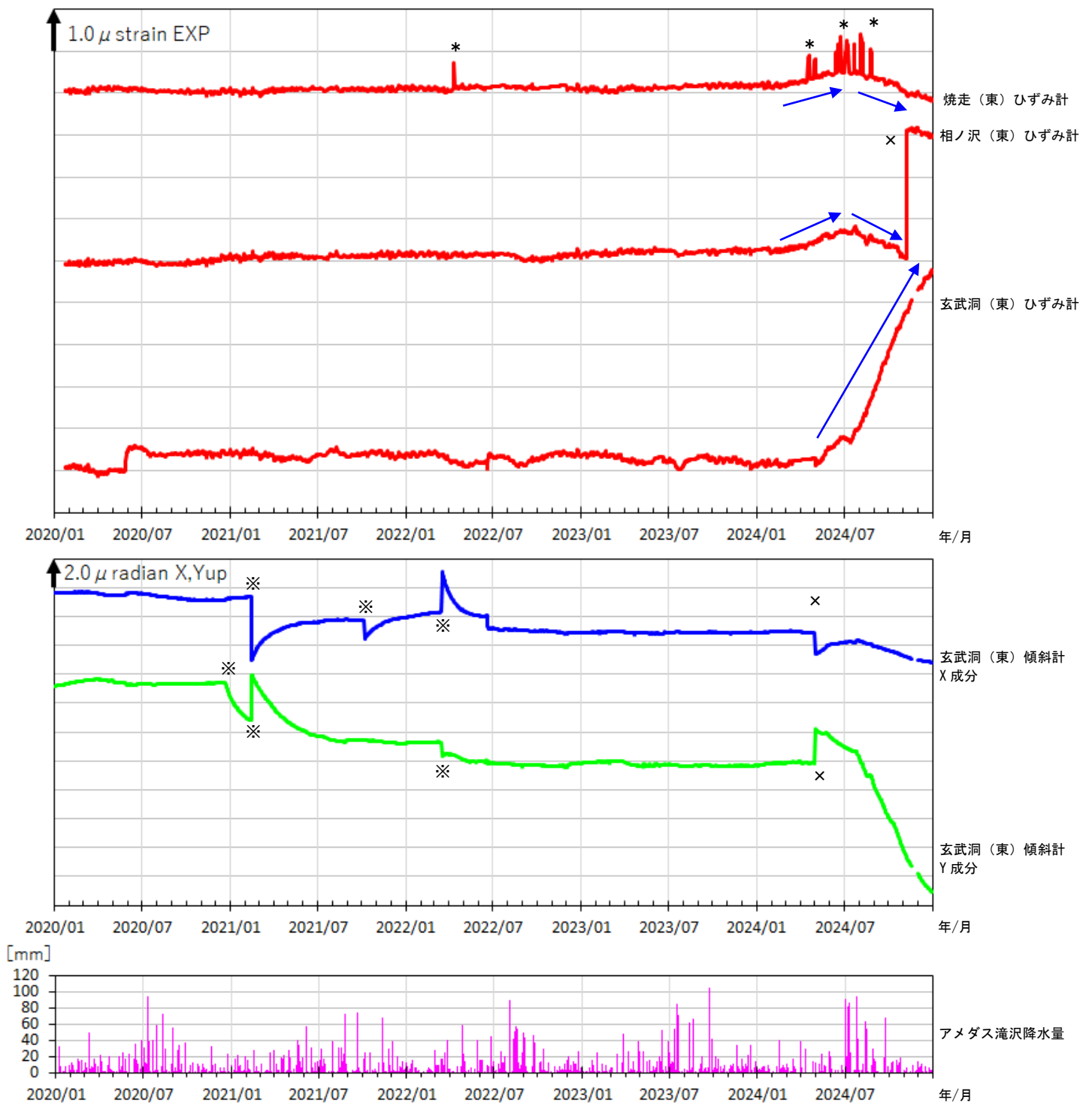
図6 岩手山 ひずみ計・傾斜計（日値・トレンド補正済み）による地殻変動の状況 （2020年1月～2024年12月）
