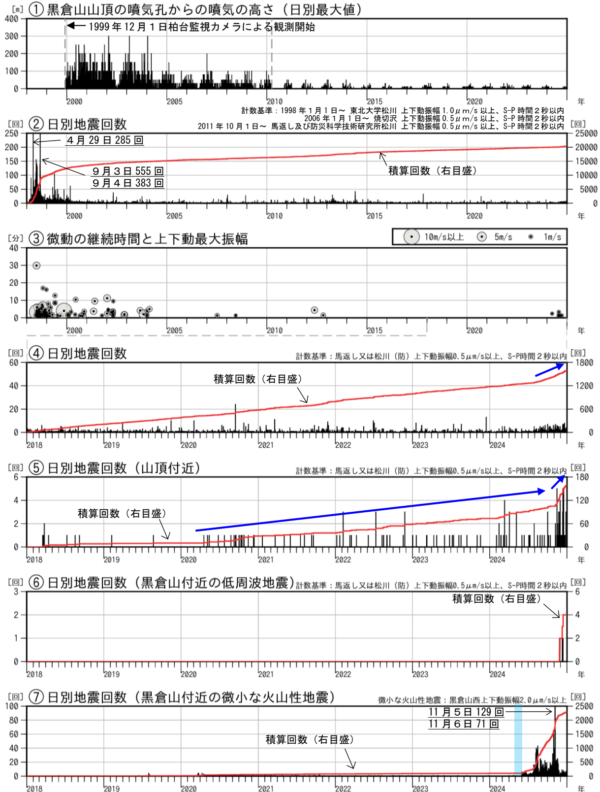
図3 岩手山 火山活動経過図（1998年1月～2024年12月）
