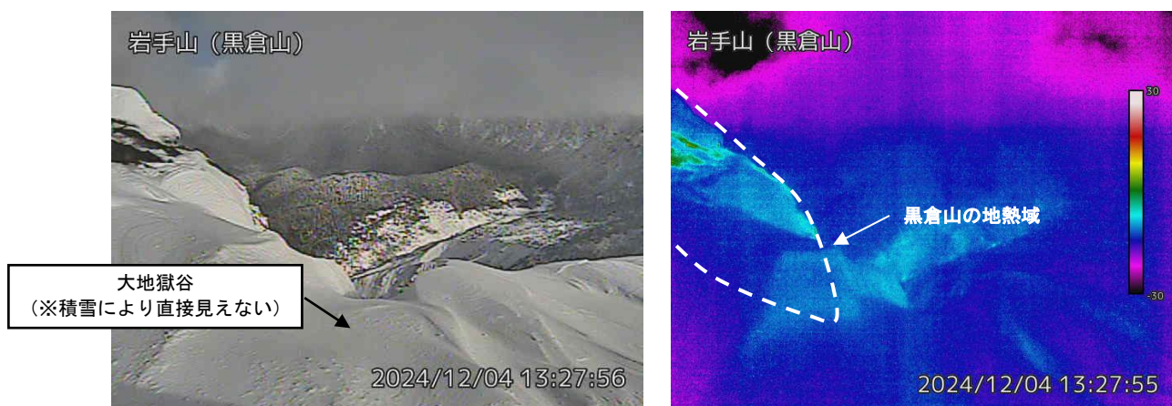
図1 岩手山 黒倉山監視カメラからの状況と地表面温度分布（12月4日）
