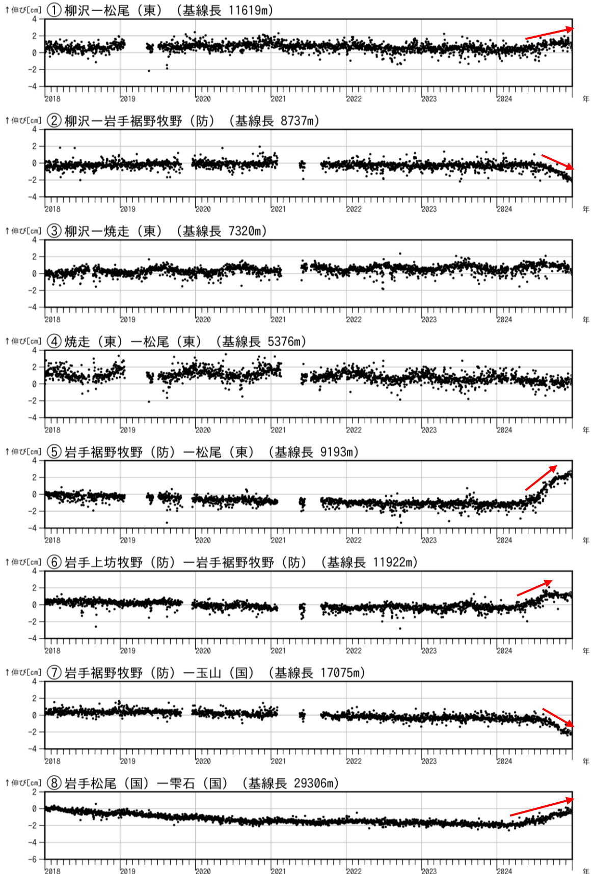
図5 岩手山 GNSS 基線長変化図（2018年1月～2024年12月）
