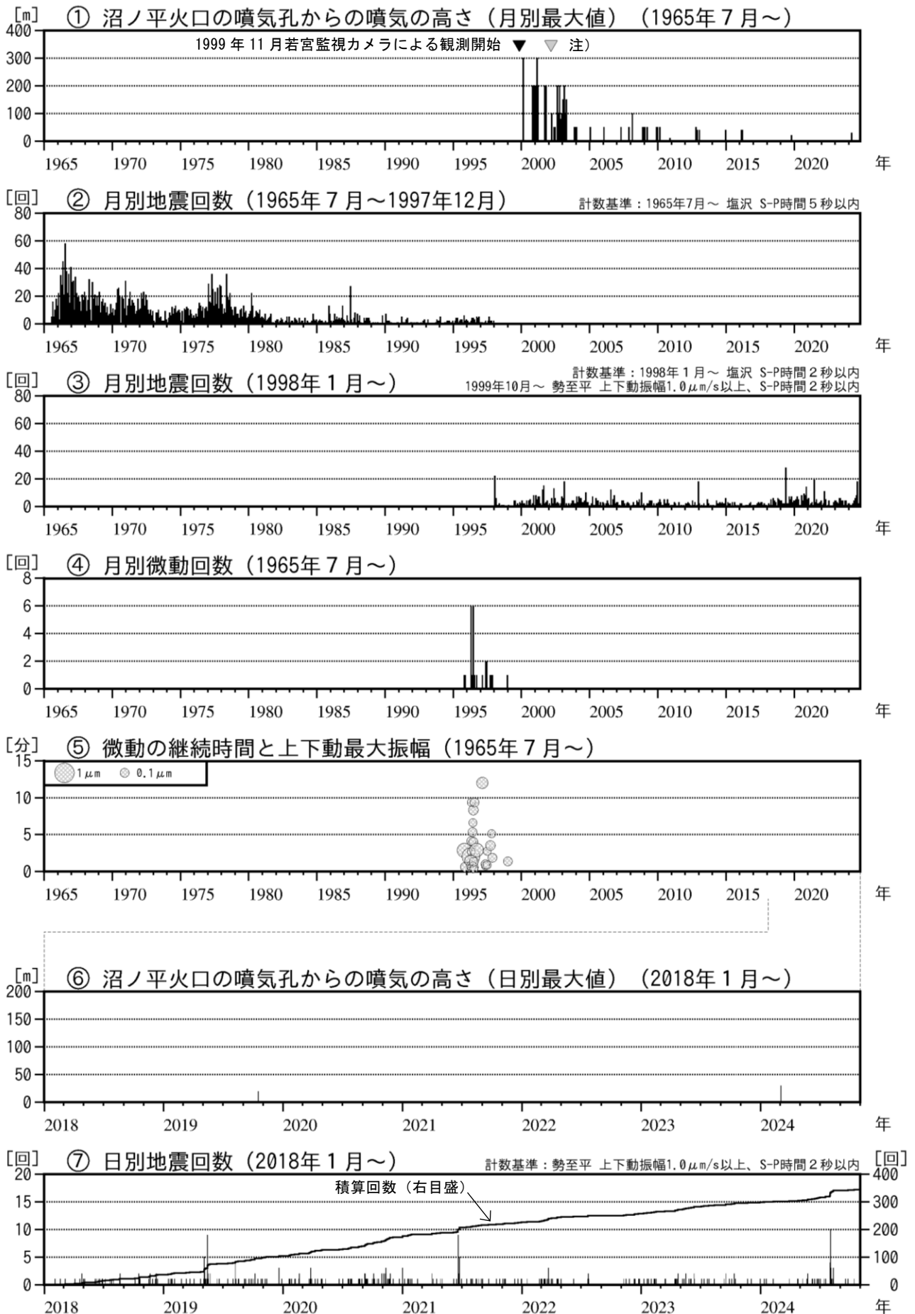
図3 安達太良山 火山活動経過図（1965年7月～2024年10月）
