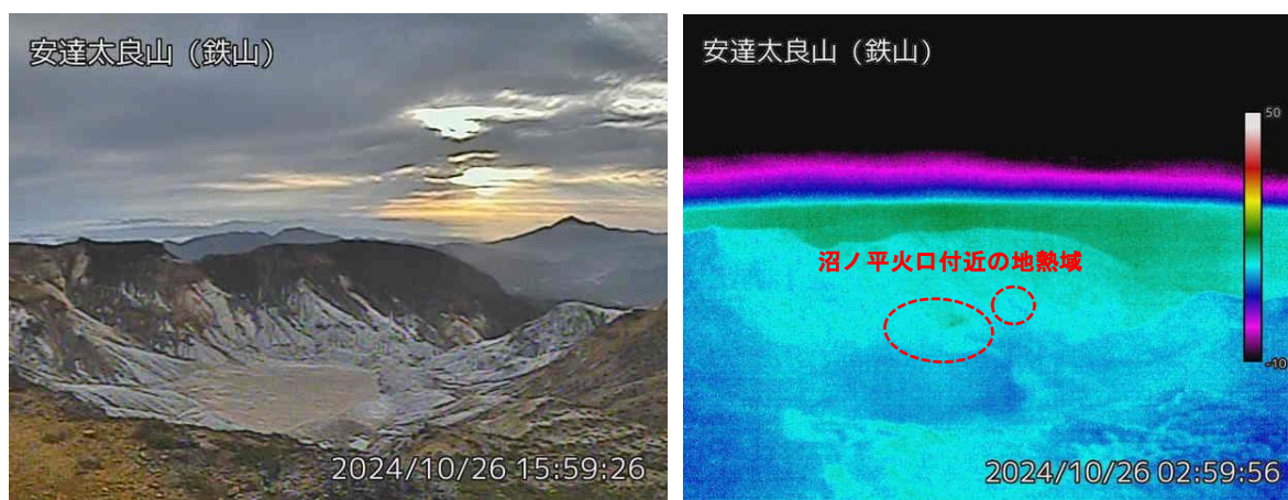
図2 安達太良山 沼ノ平火口周辺の状況と地表面温度分布の状況（10月26日） ・鉄山監視カメラ（沼ノ平火口の北東約700m）の映像です。
