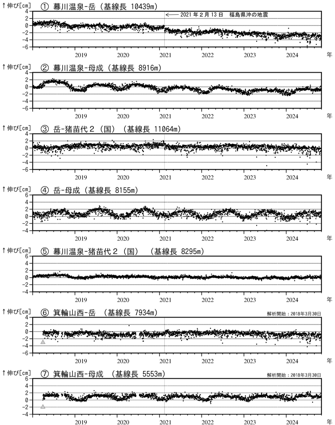
図4 安達太良山 GNSS 基線長変化図 (2018年1月～2024年10月)
