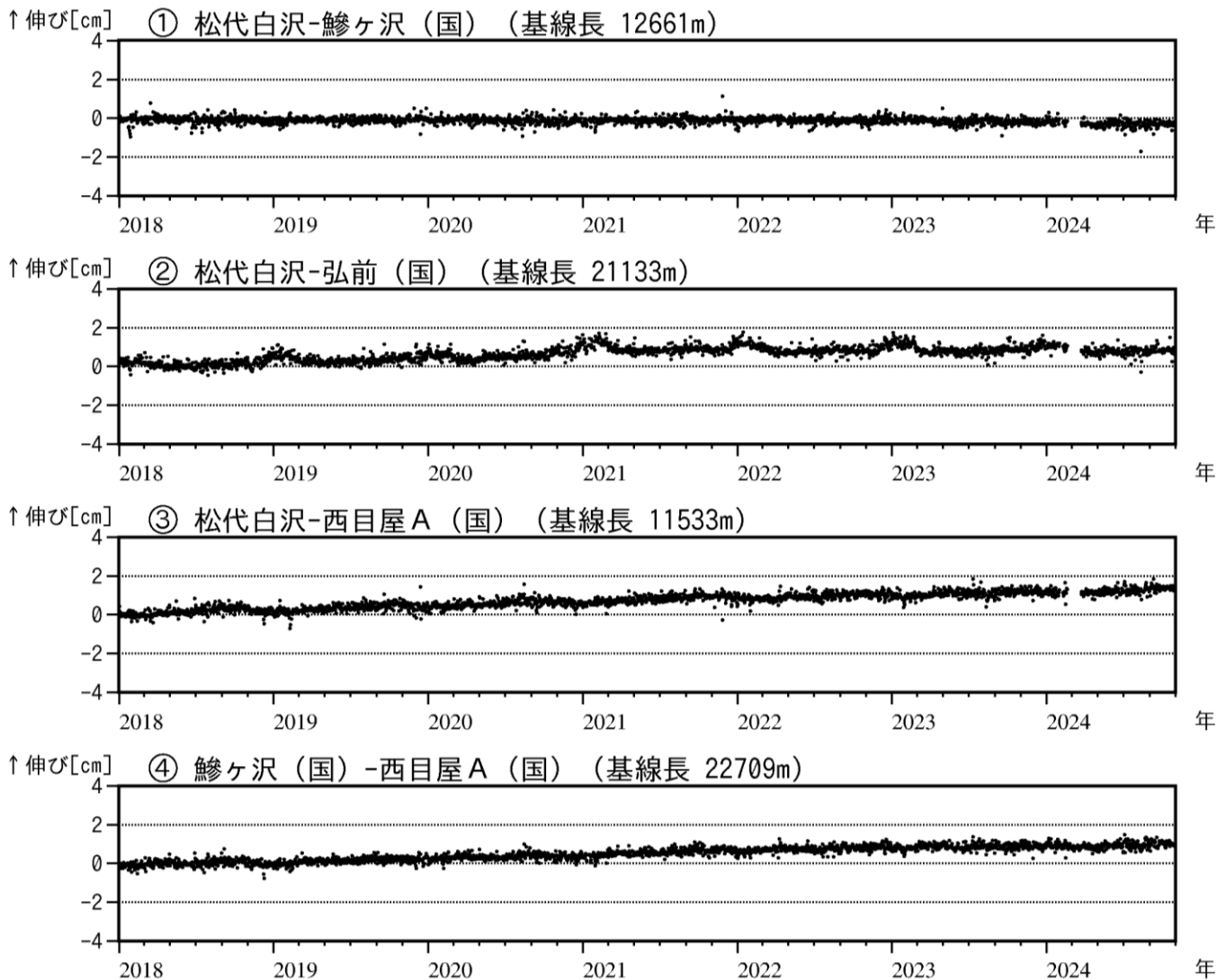
図3 岩木山 GNSS 基線長変化図（2018年1月～2024年10月）
