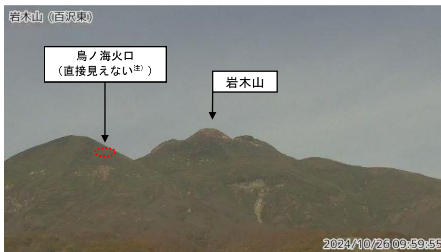
図1 岩木山 山頂部の状況（10月26日）
