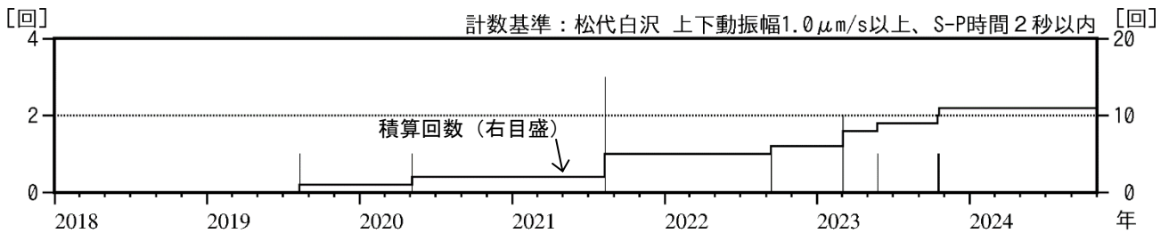
図2 岩木山 日別地震回数（2018年1月～2024年10月）
