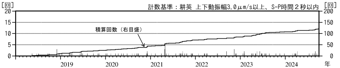
図2 栗駒山 日別地震回数（2018年1月～2024年9月）
