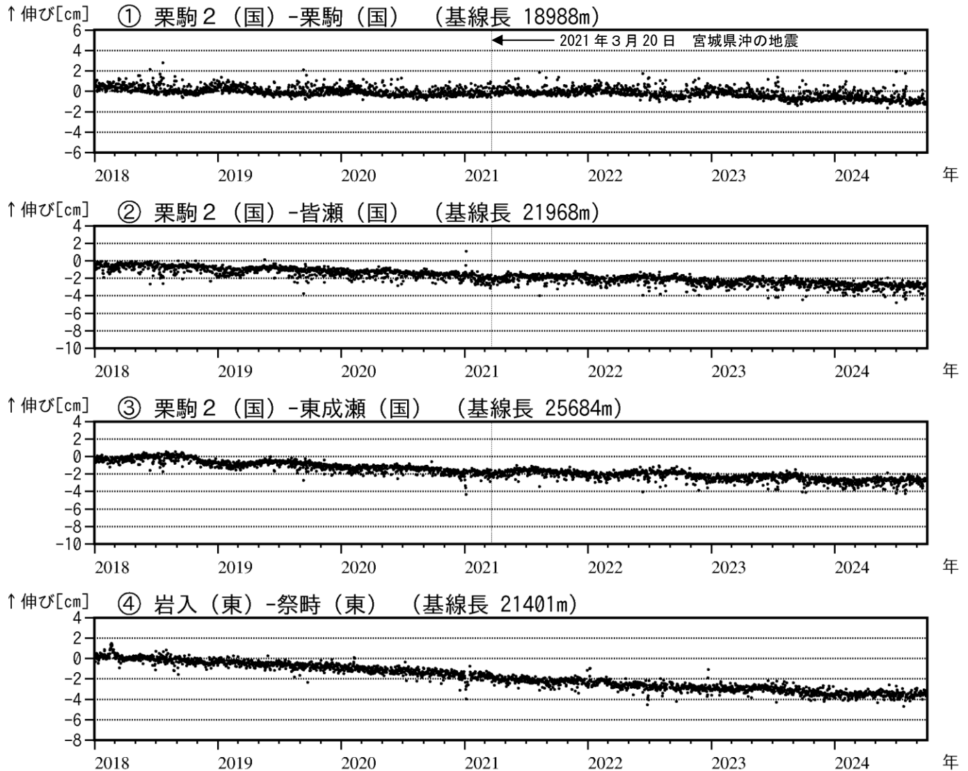
図3 栗駒山 GNSS 基線長変化図（2018年1月～2024年9月）
