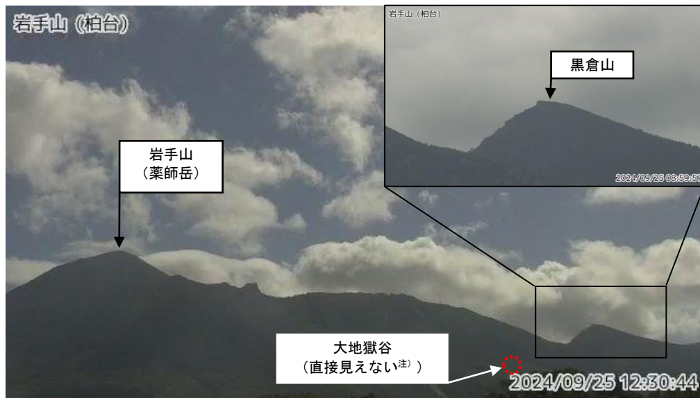
図4 岩手山 山頂部から黒倉山周辺の状況（9月25日）
