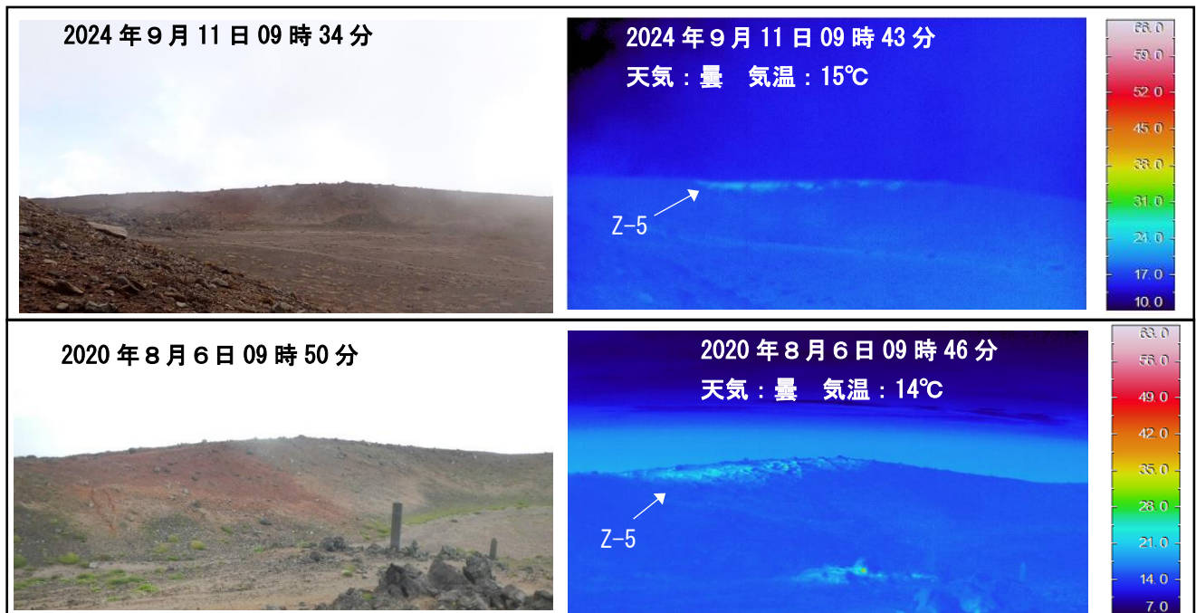
図9 岩手山 岩手山山頂付近の状況と地表面温度分布
