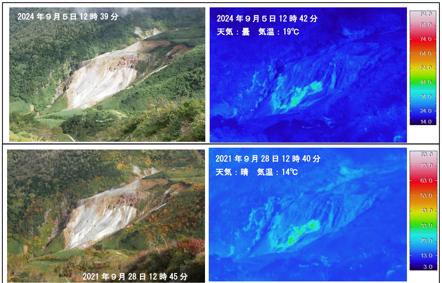
図7 岩手山 大地獄谷の状況と地表面温度分布
