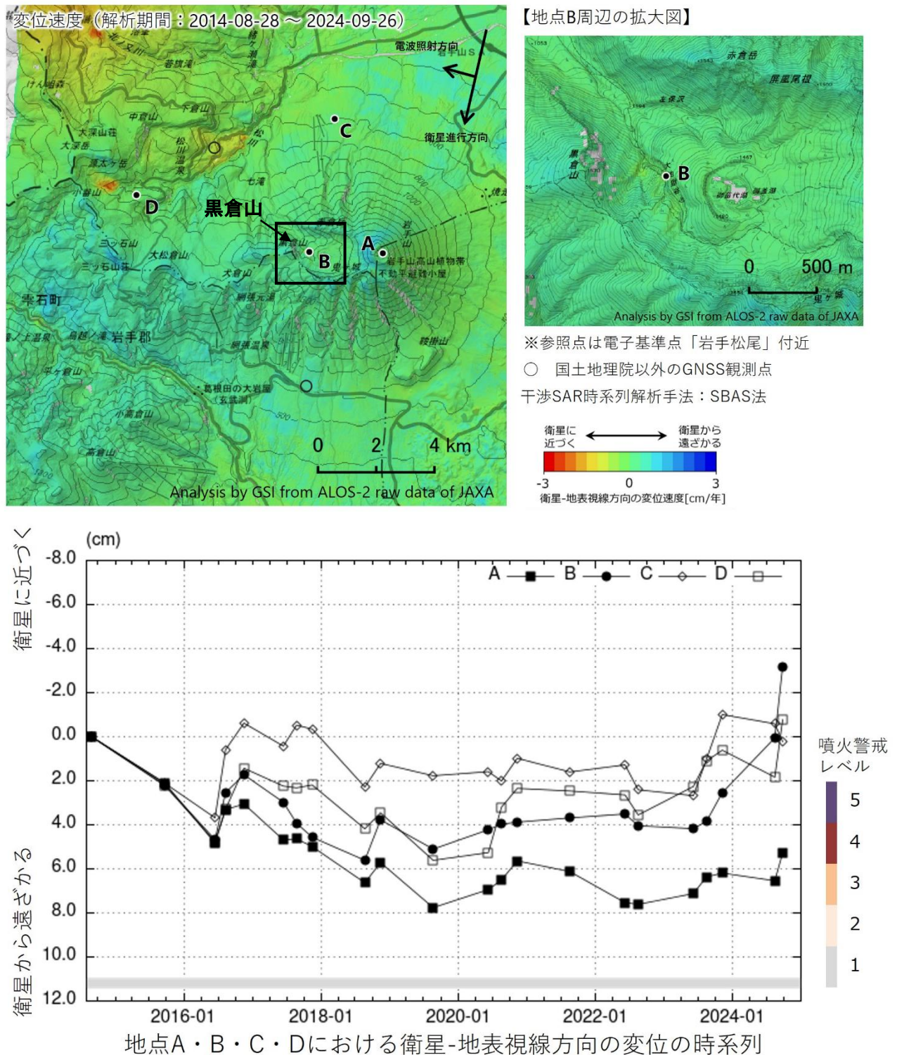
図3 岩手山 国土地理院の干渉 SAR 時系列解析結果（2014 年 8 月 28 日から 2024 年 9 月 26 日の変化） ・ 国土地理院が作成した図に地名等一部加筆をしています。
