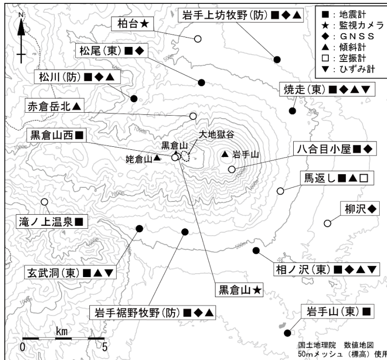
図 15 岩手山 観測点配置図
