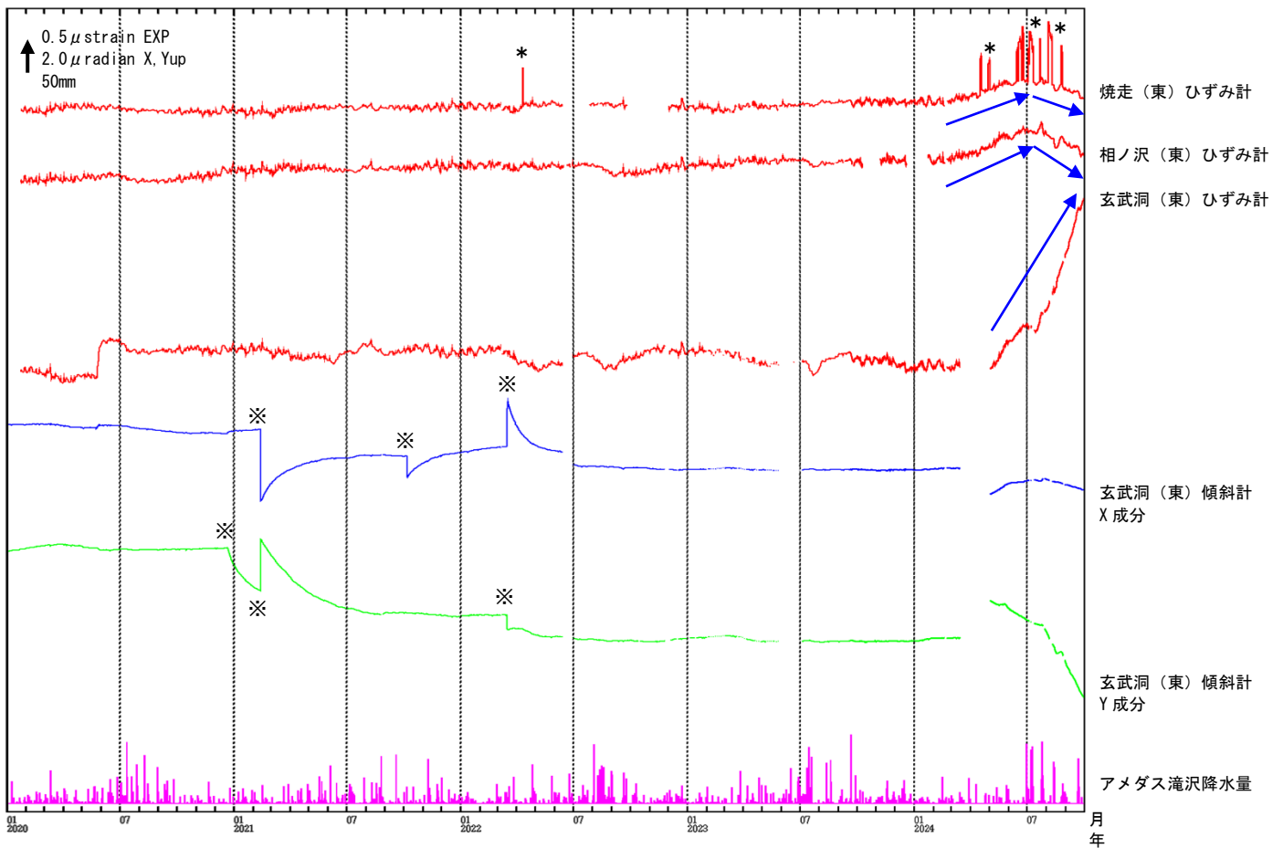
図 14 岩手山 ひずみ計・傾斜計（日値・トレンド補正済み）による地殻変動の状況 （2020 年 1 月～2024 年 9 月）
