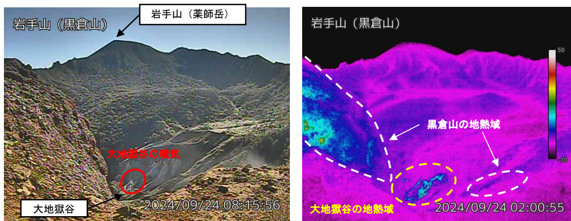
図5 岩手山 黒倉山監視カメラからの状況と地表面温度分布（9月24日）
