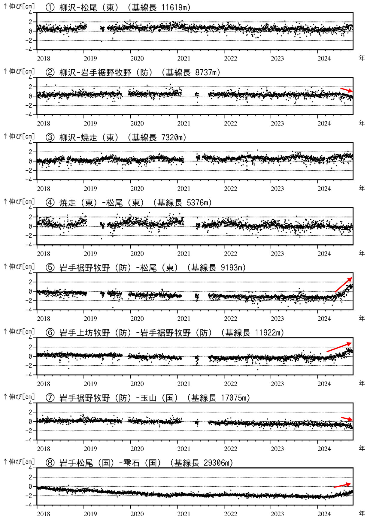
図 13 岩手山 GNSS 基線長変化図 (2018 年 1 月～2024 年 9 月)
