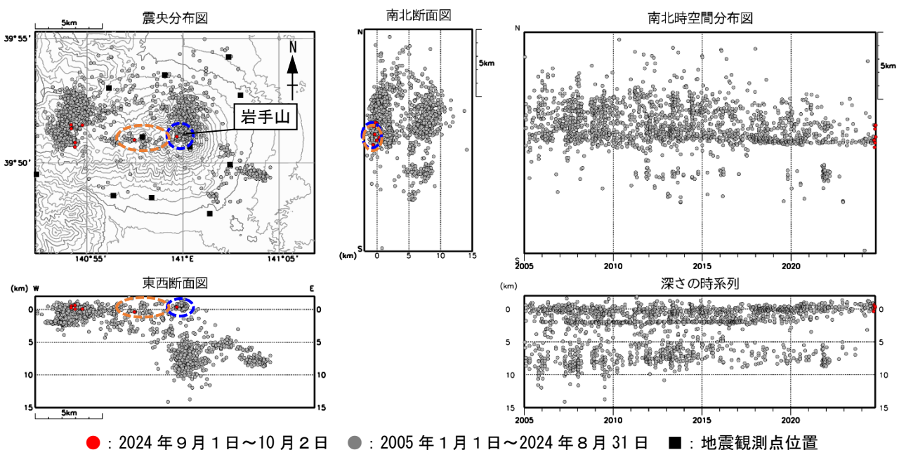
図12 岩手山 地震活動（2005年1月～2024年10月2日）
