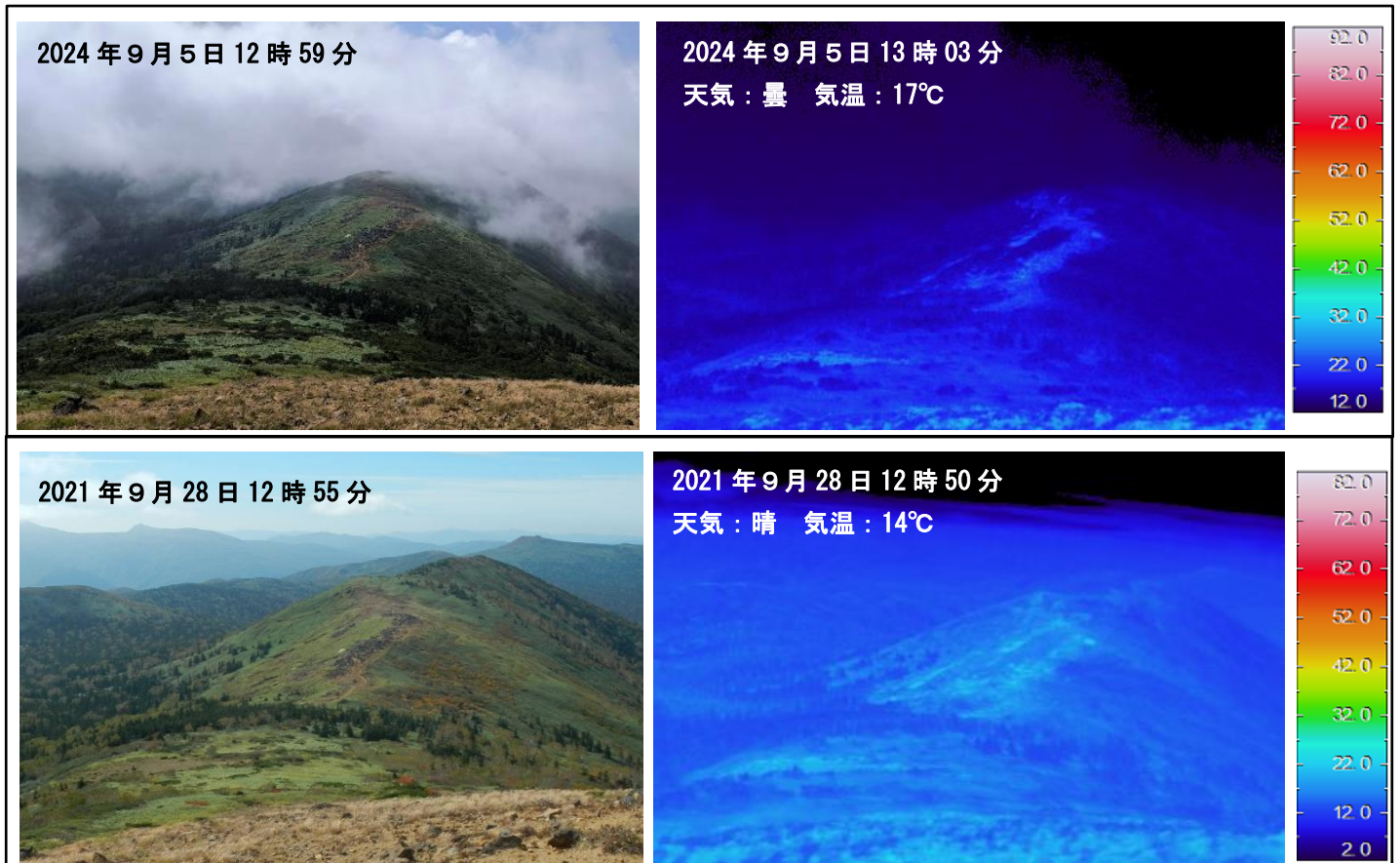
図8 岩手山 姥倉山東斜面の状況と地表面温度分布
