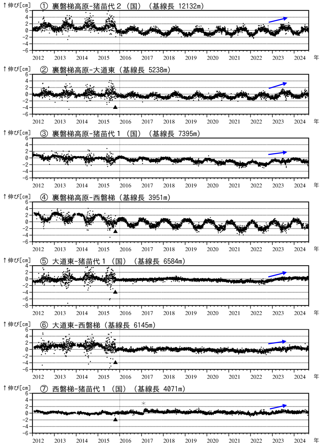
図6 磐梯山 GNSS基線長変化図（2012年1月～2024年8月）
