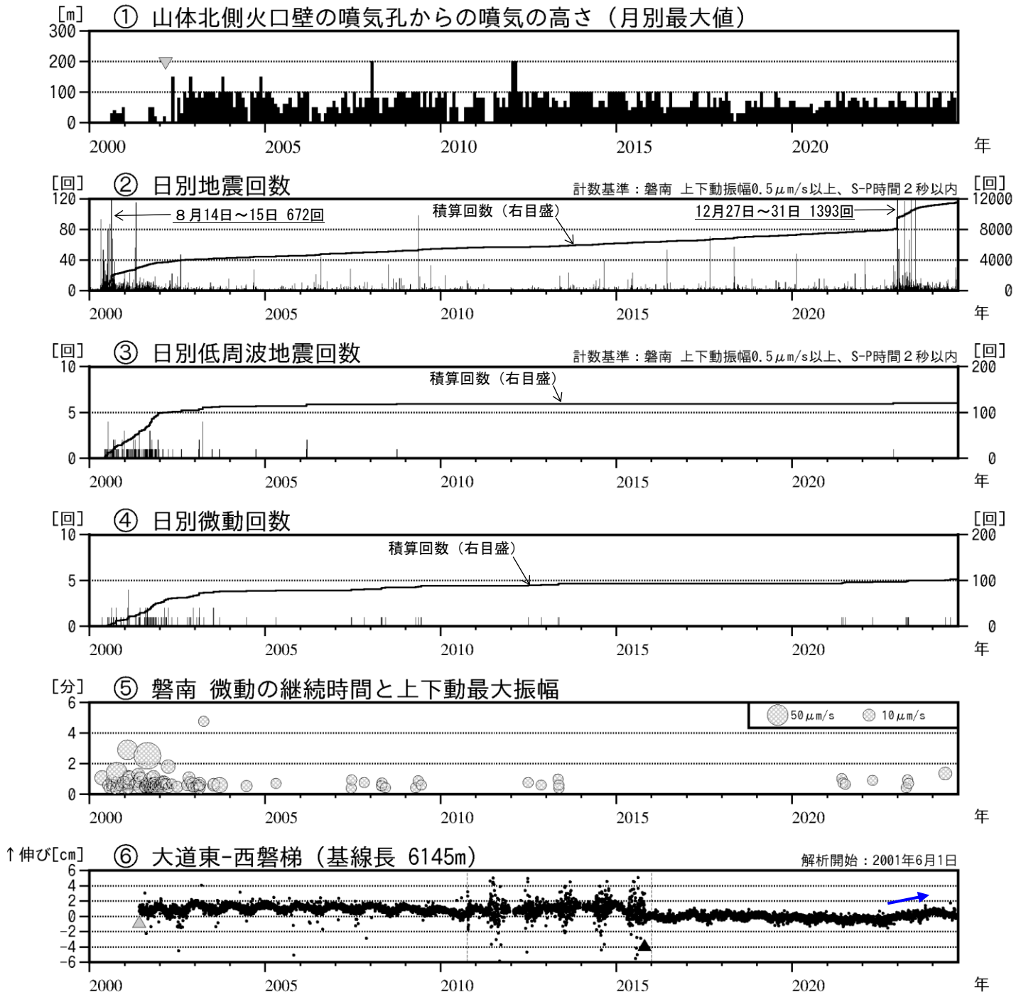
図3 磐梯山 火山活動経過図（2000年1月～2024年8月）
