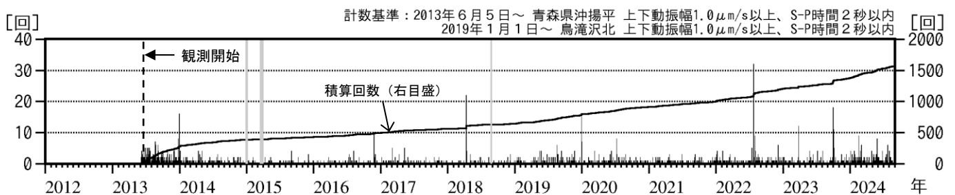
図2 八甲田山 日別地震回数（2013年6月～2024年8月）
