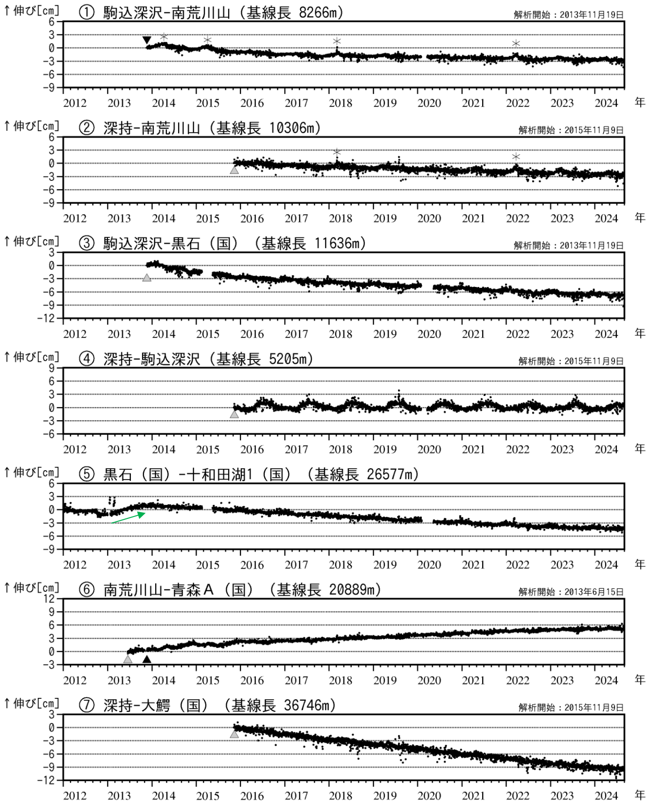
図3 八甲田山 GNSS 基線長変化図（2012年1月～2024年8月）
