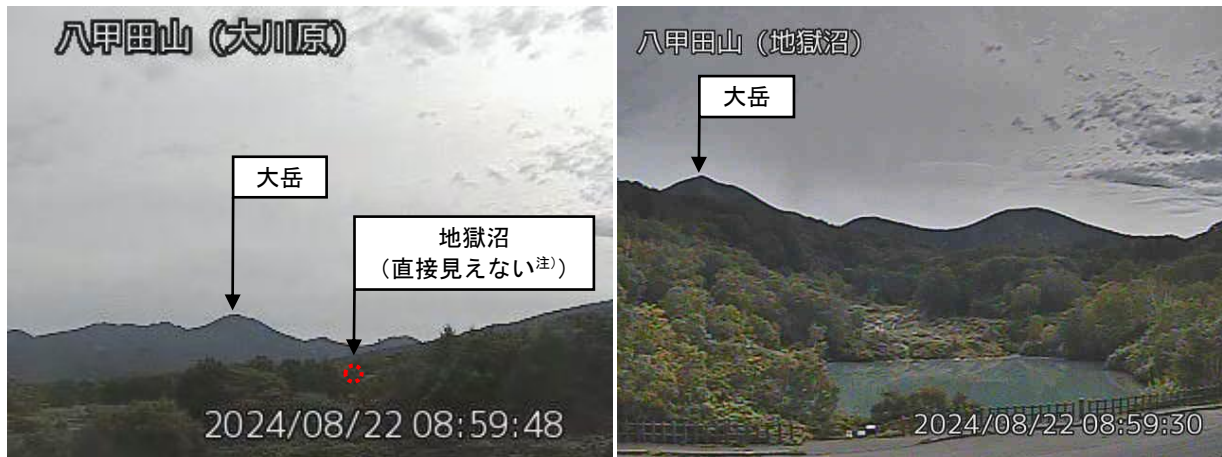
図1 八甲田山 山頂部及び地獄沼周辺（8月22日）の状況
