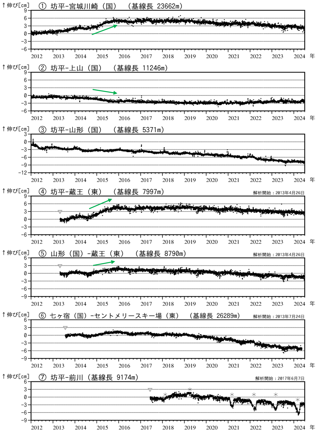
図3 蔵王山 GNSS 基線長変化図 (2012年1月～2024年6月)
