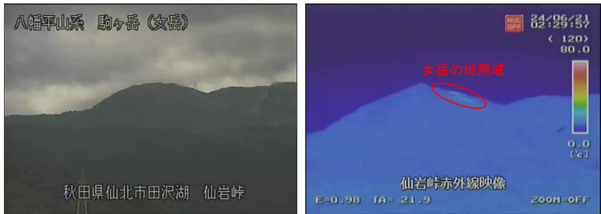
図1 秋田駒ヶ岳 女岳周辺の状況（6月27日）と地表面温度分布の状況（6月21日） ・東北地方整備局が設置している仙岩峠監視カメラ（女岳山頂の南約5km）の可視及び赤外映像です。
