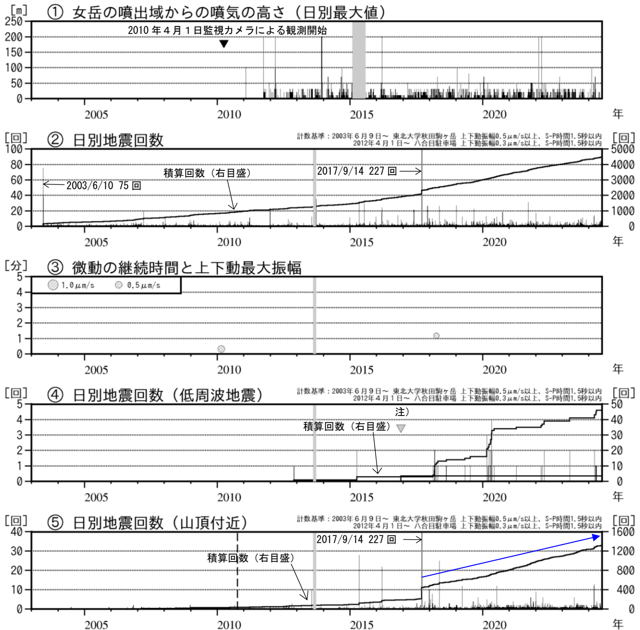
図2 秋田駒ヶ岳 火山活動経過図（2003年6月～2024年6月）
