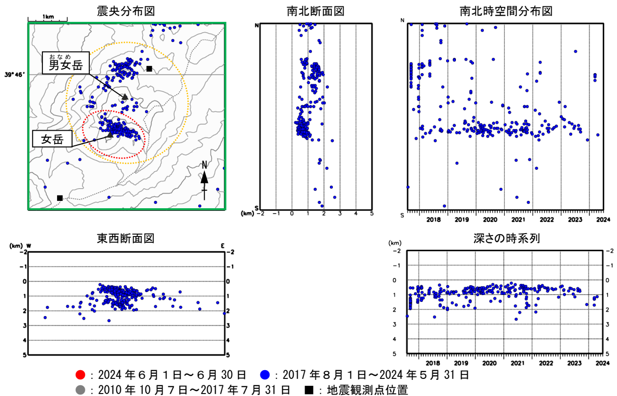
図4 秋田駒ヶ岳 地震活動（2010年10月7日～2024年6月）
