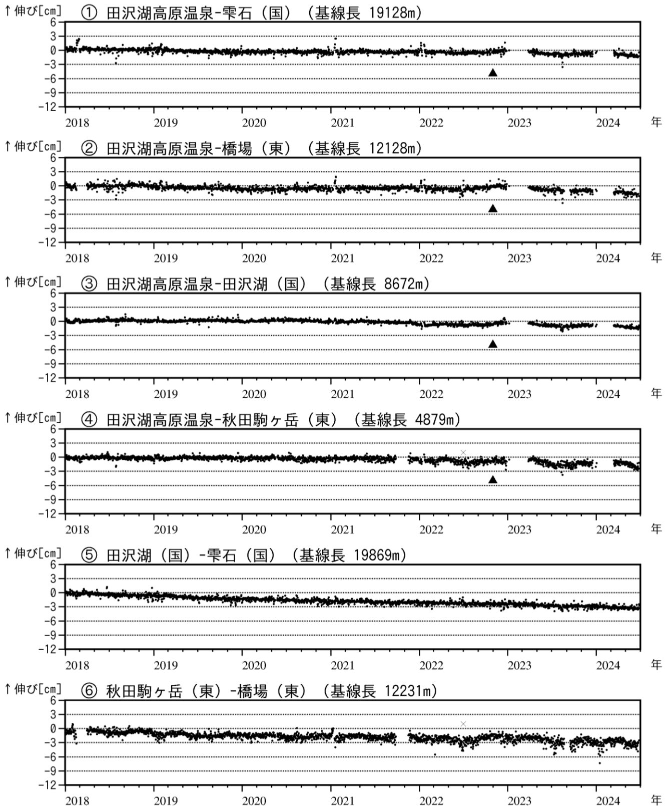
図5 秋田駒ヶ岳 GNSS 基線長変化図 (2018年1月~2024年6月)
