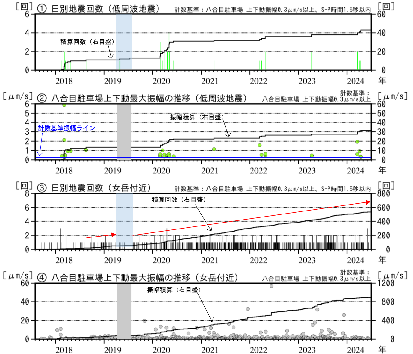
図3 秋田駒ヶ岳 低周波地震及び女岳付近の日別回数と最大振幅（2017年8月～2024年6月）
