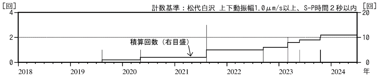
図2 岩木山 日別地震回数（2018年1月～2024年6月）
