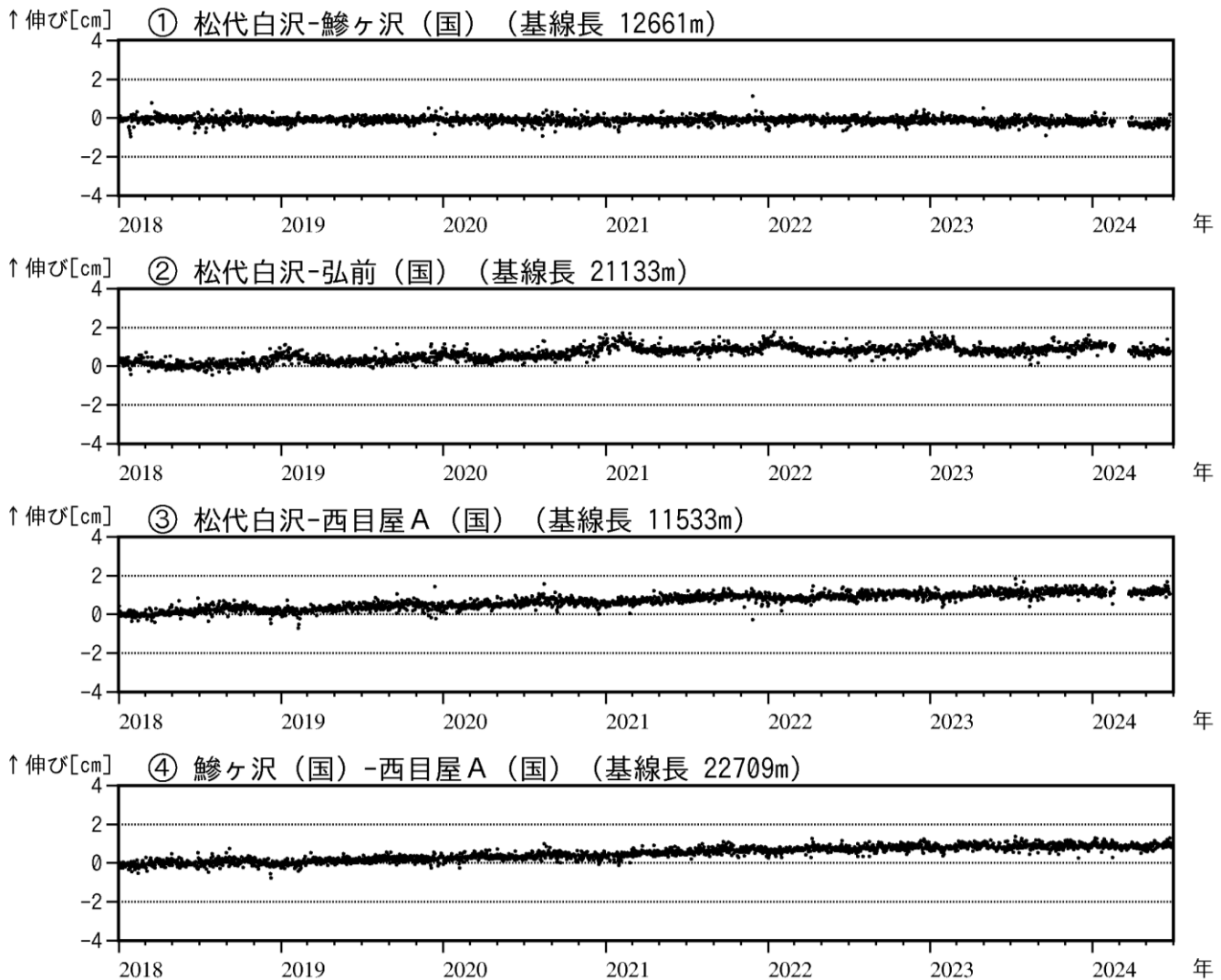
図3 岩木山 GNSS 基線長変化図（2018年1月～2024年6月）
