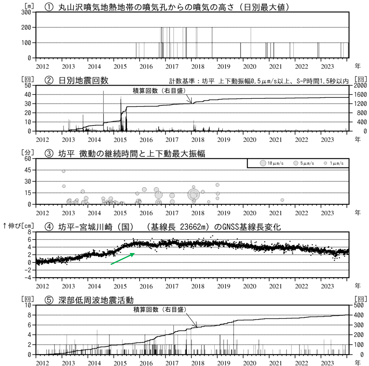
図2 蔵王山 火山活動経過図（2012年1月～2024年1月）
