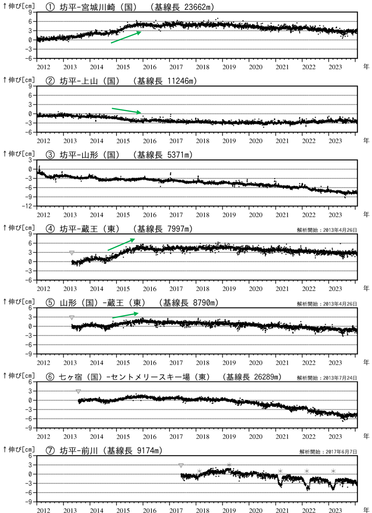
図3 蔵王山 GNSS 基線長変化図 (2012年1月～2024年1月)
