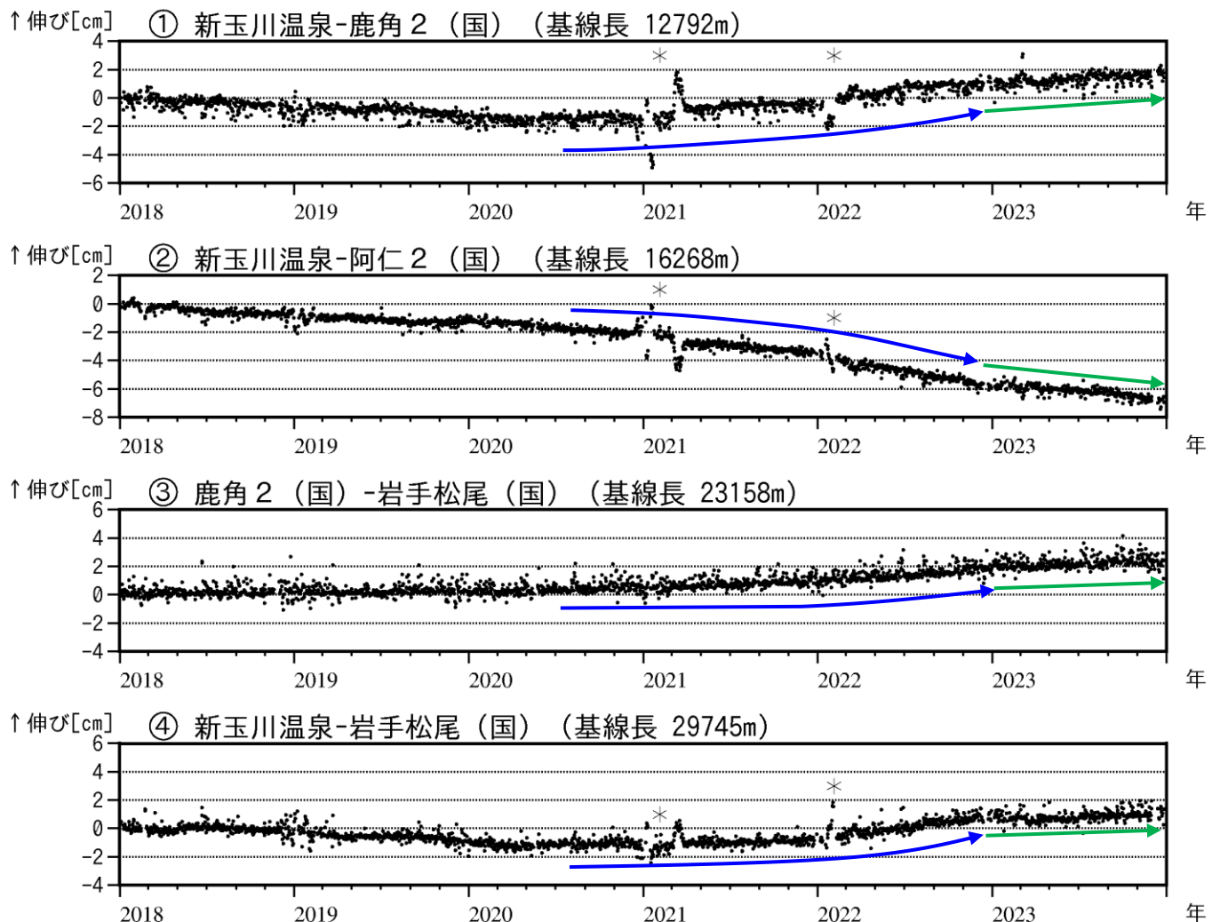
図4 秋田焼山 GNSS 基線長変化図（2018年1月～2023年12月）
