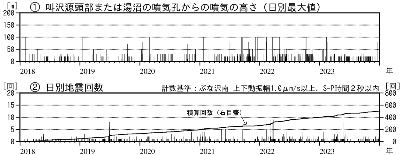
図3 秋田焼山 火山活動経過図（2018年1月～2023年12月）
