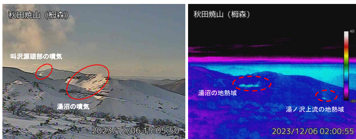
図2 秋田焼山 湯沼と湯ノ沢上流の状況と地表面温度分布（12月6日）
