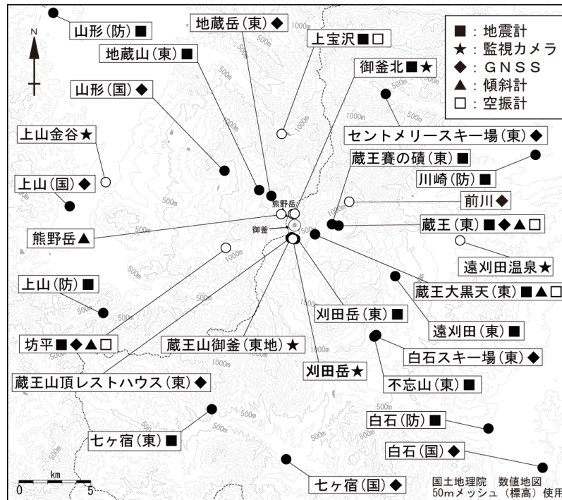
図7 蔵王山 観測点配置図
