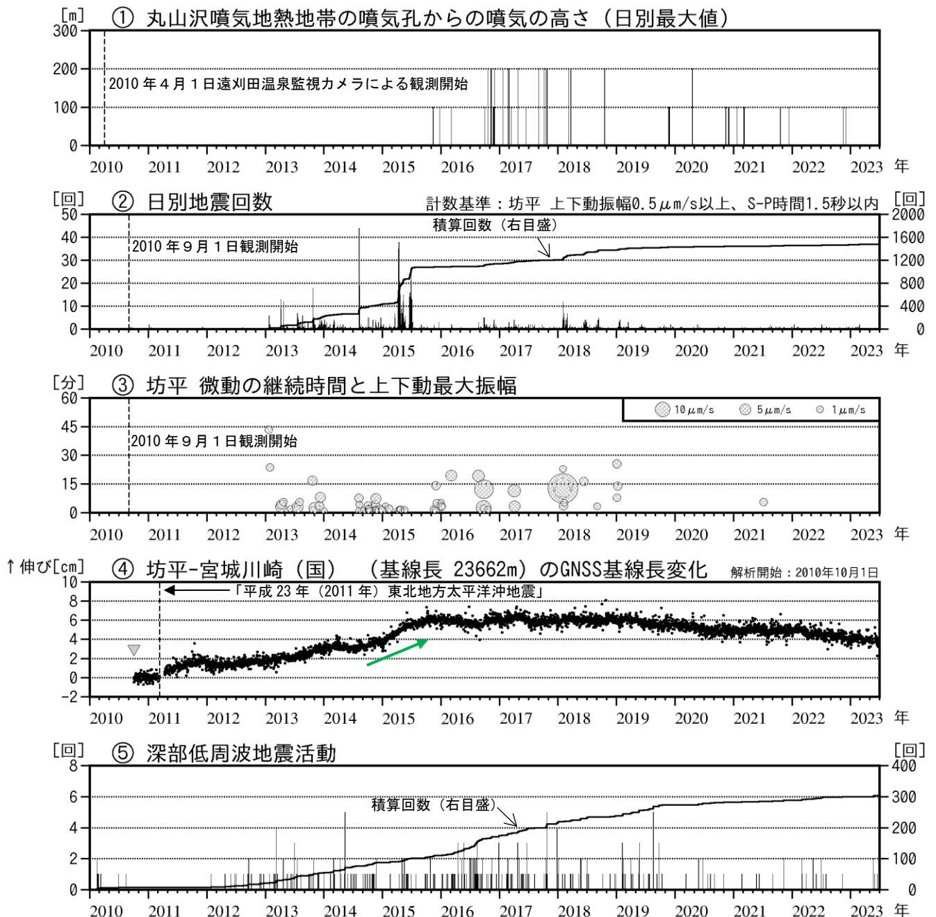
図5 蔵王山 火山活動経過図（2010年4月～2023年6月）
