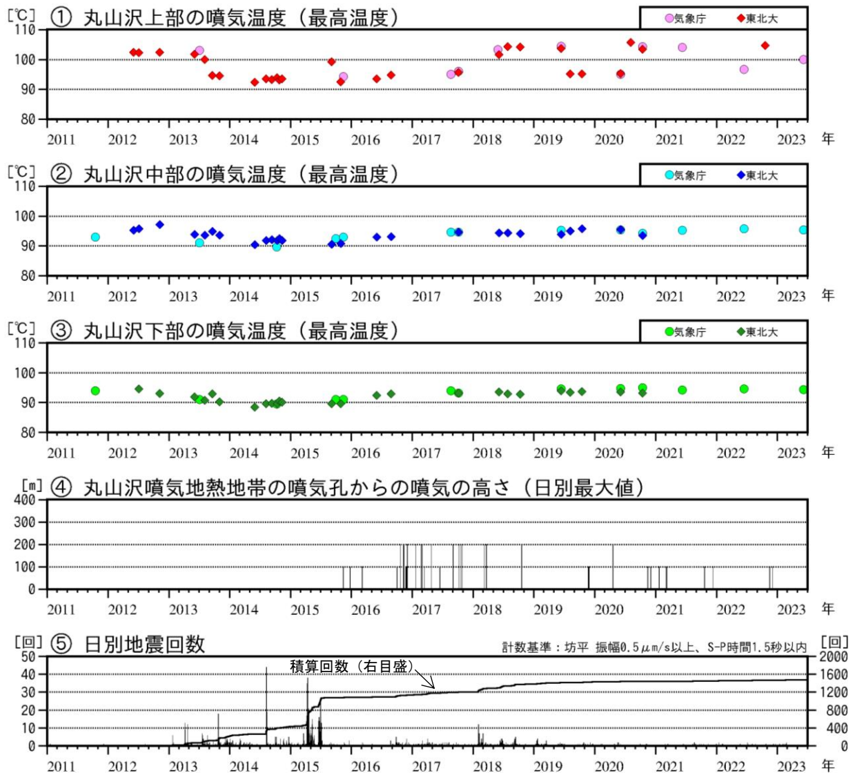
図4 蔵王山 丸山沢の噴気温度、噴気の高さ及び日別地震回数（2011年1月～2023年6月）
