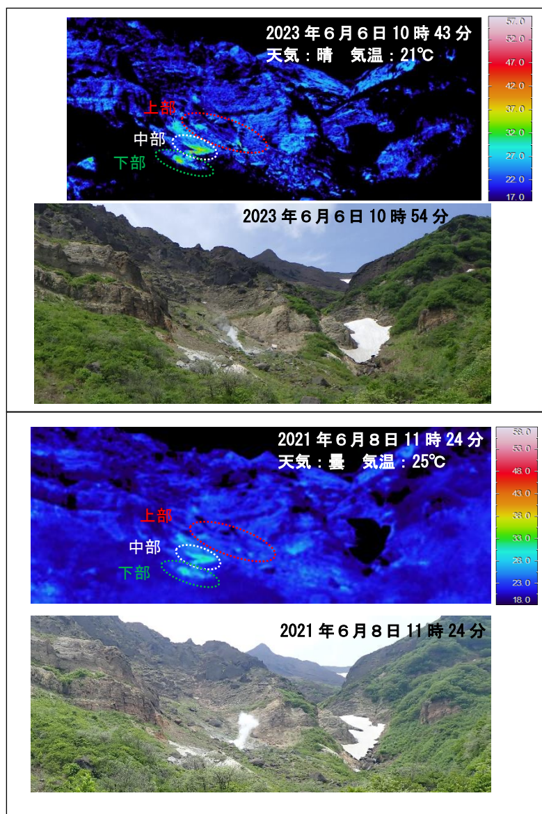
図3 蔵王山 東方向から撮影した丸山沢の状況（下段）と地表面温度分布（上段） ・地熱域以外で温度の高い部分は、岩等が日射により温められたことによるものと推定されます。
