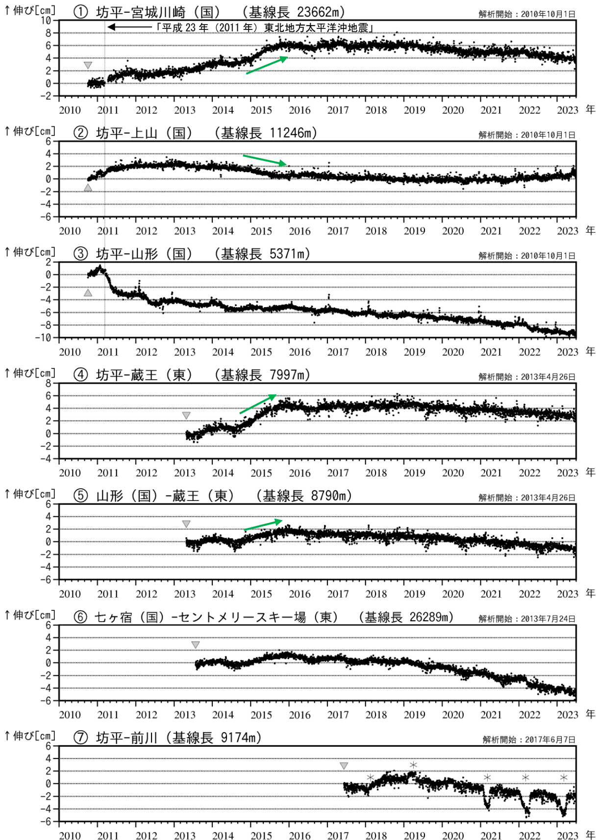
図6 蔵王山 GNSS 基線長変化図（2010年10月～2023年6月）
