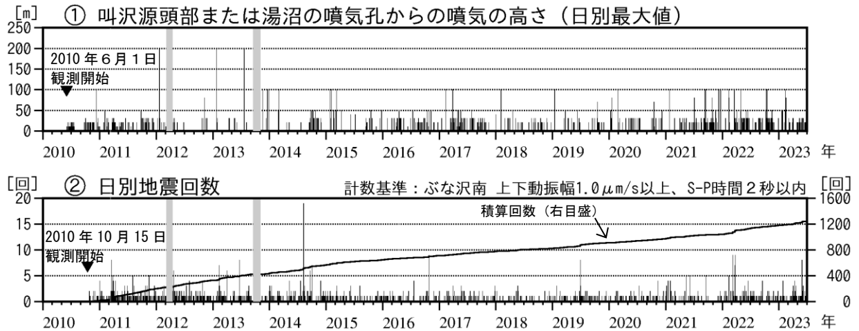
図3 秋田焼山 火山活動経過図（2010年6月～2023年6月）
