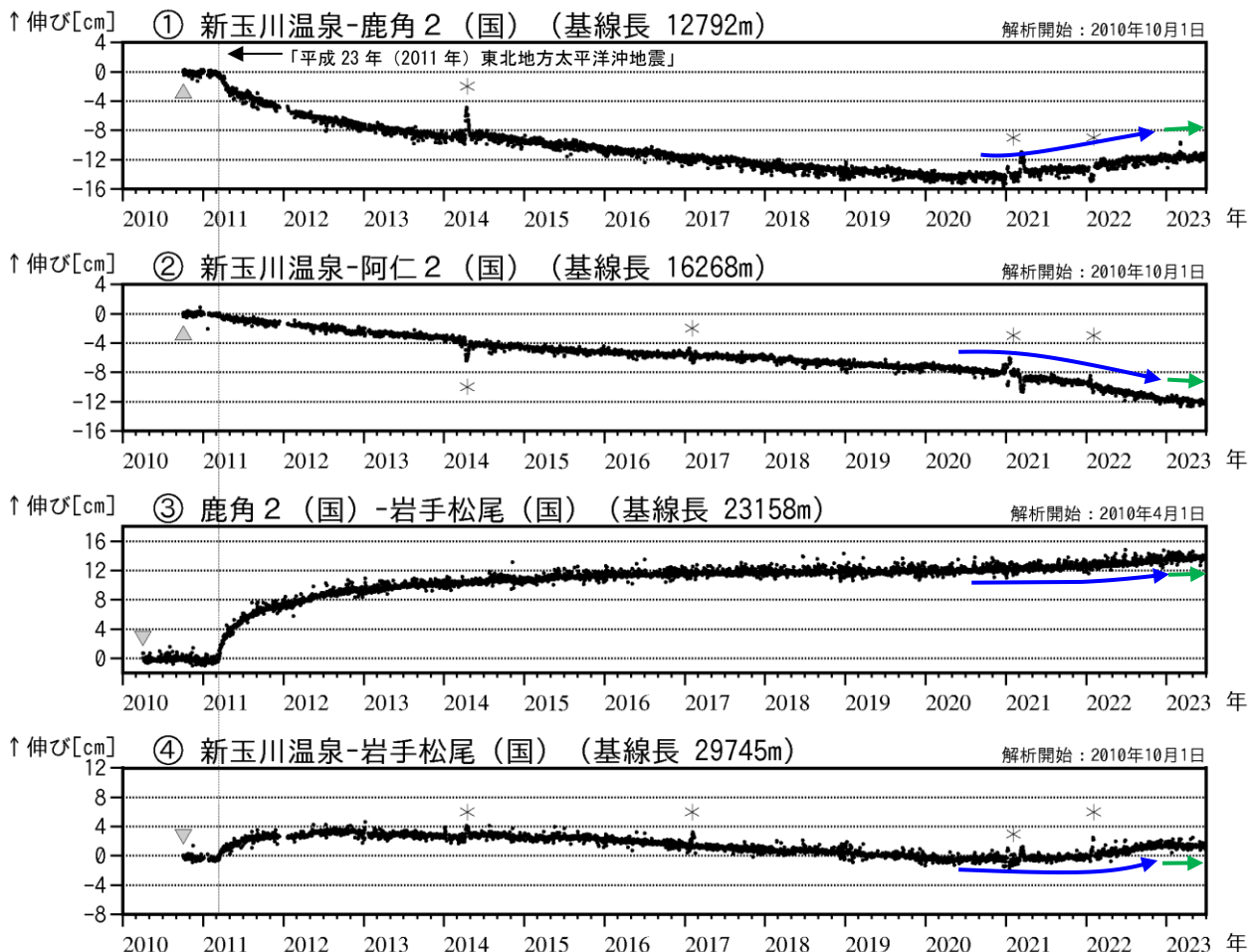
図4 秋田焼山 GNSS 基線長変化図（2010年4月～2023年6月）
