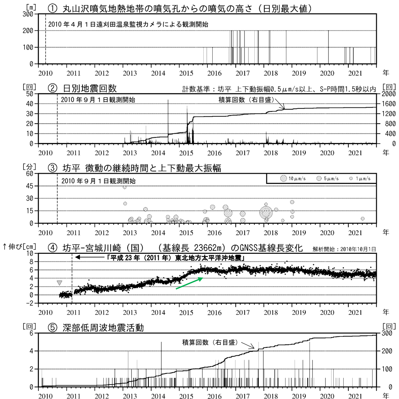
図2 蔵王山 火山活動経過図（2010年4月～2021年12月）
