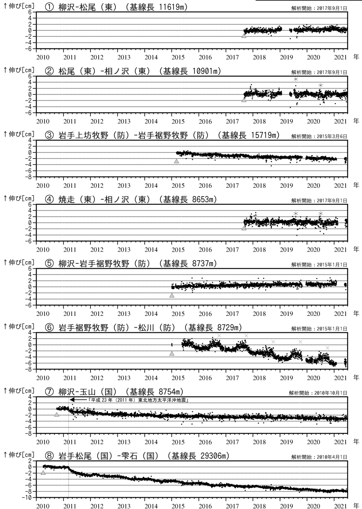
図6 岩手山 GNSS 基線長変化図 (2010 年 4 月～2021 年 6 月)
