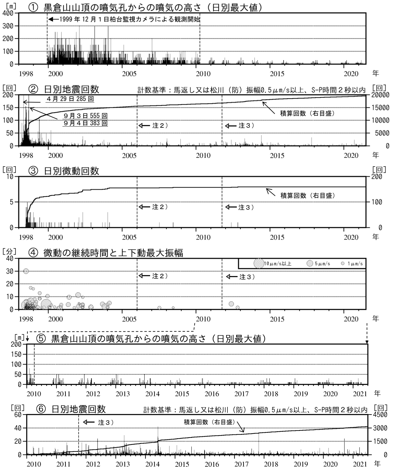
図5 岩手山 火山活動経過図（1998年1月～2021年6月）
