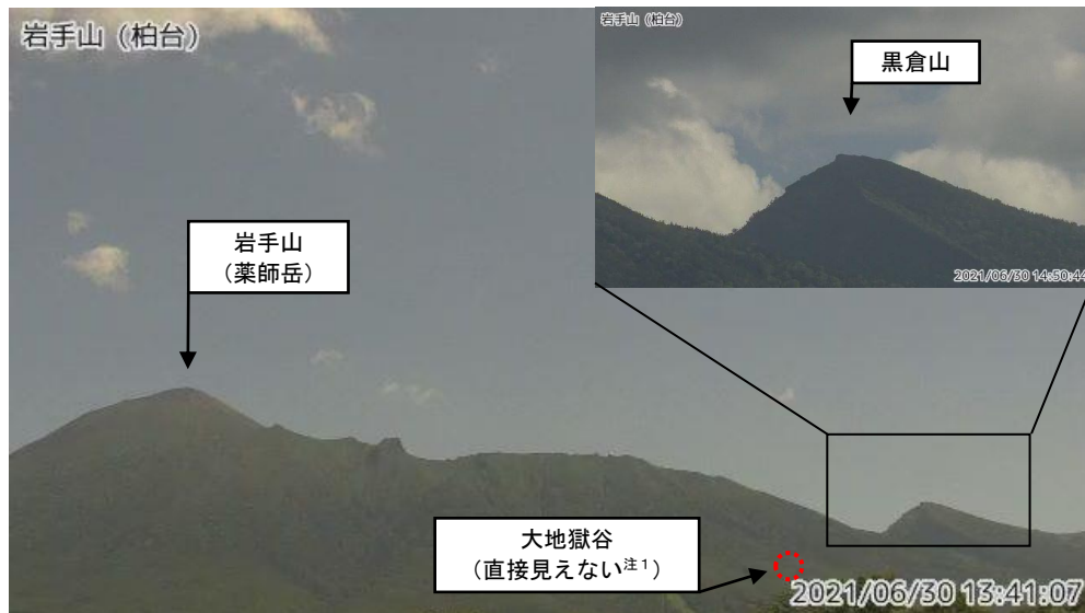
図1 岩手山 山頂部から黒倉山周辺の状況（6月30日）
