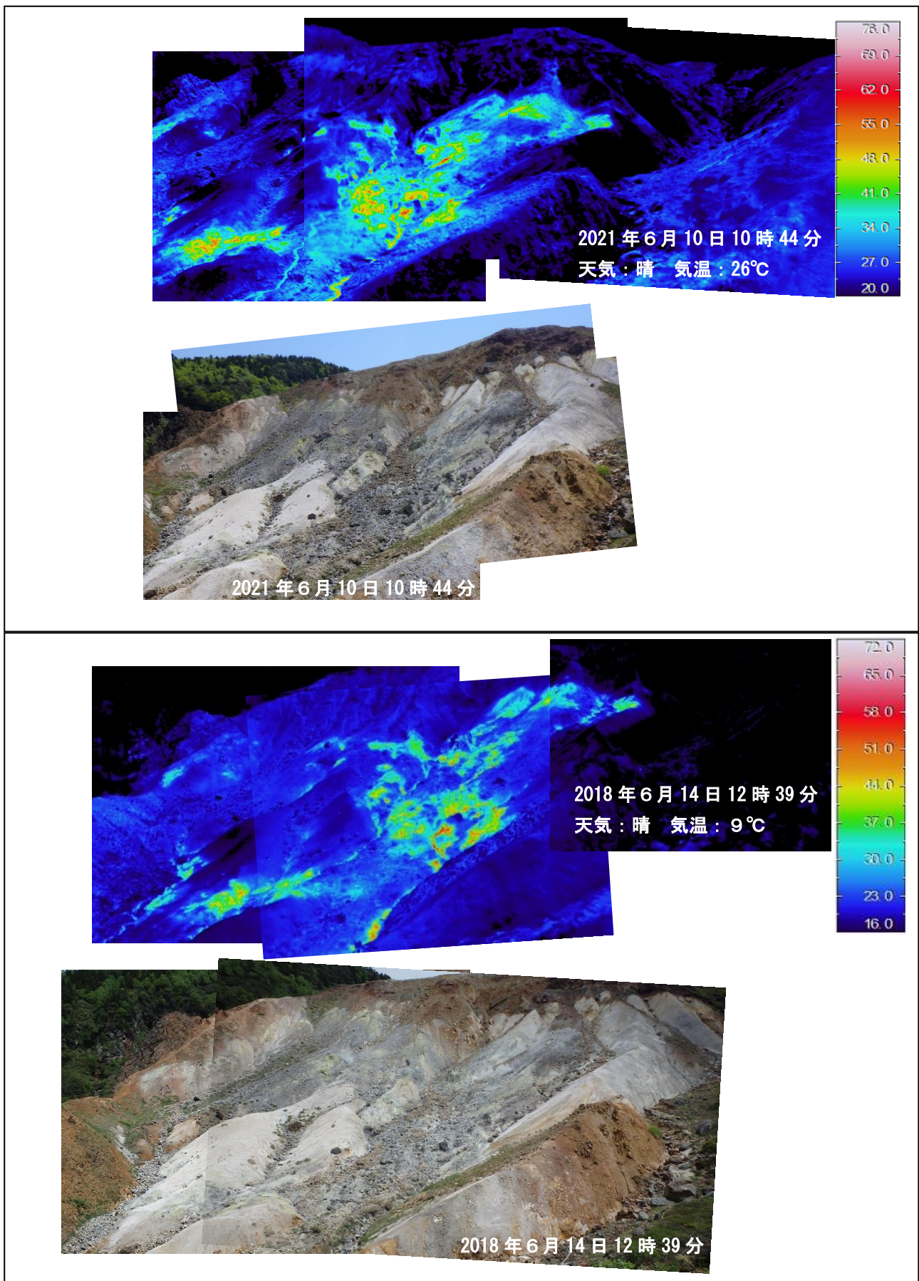
図4 岩手山 北西から撮影した大地獄谷の状況と地表面温度分布
