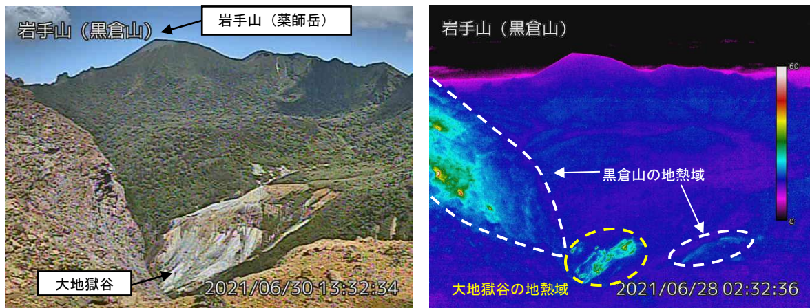
図2 岩手山 黒倉山監視カメラからの状況（6月30日）と地表面温度分布（6月28日）
