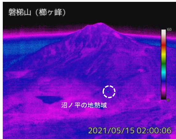
図2 磐梯山 沼ノ平周辺の状況（5月18日）と地表面温度分布（5月15日）
