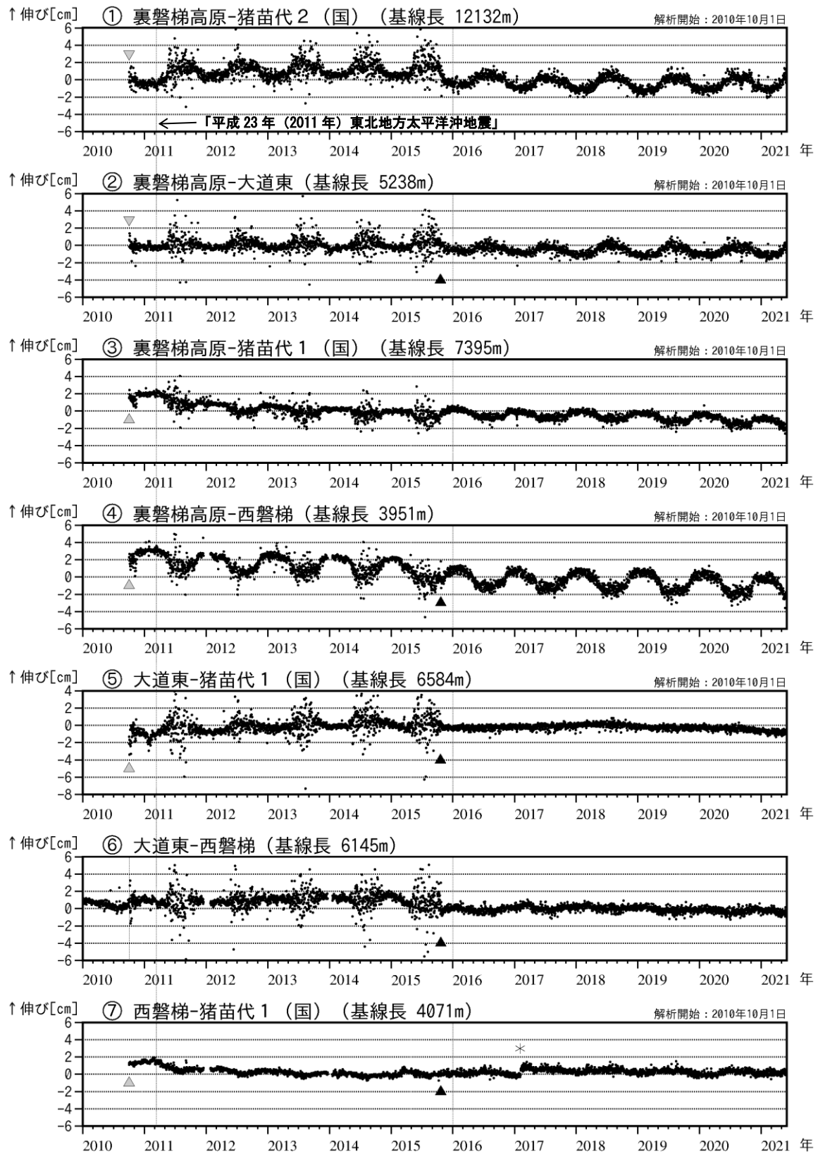
図4 磐梯山 GNSS 基線長変化図 (2010年1月～2021年5月)
