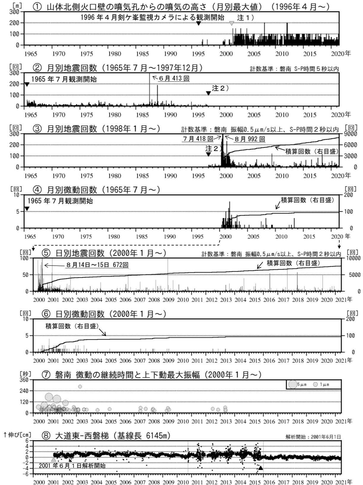
図3 磐梯山 火山活動経過図（1965年7月～2021年5月）
