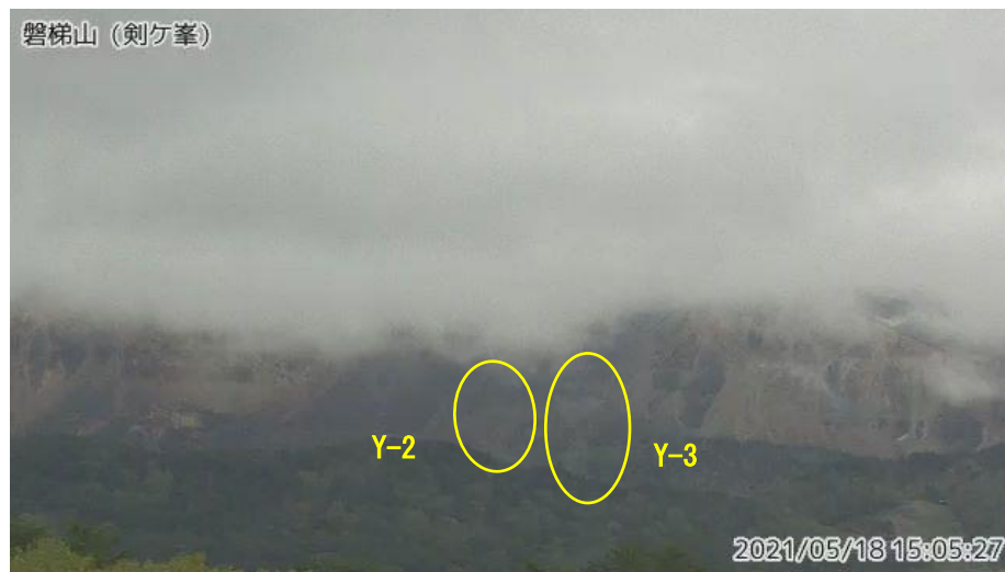
図1 磐梯山 山体北側火口壁の噴気の状態（5月18日）
