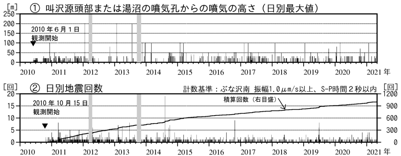
図3 秋田焼山 火山活動経過図（2010年6月～2021年4月）
