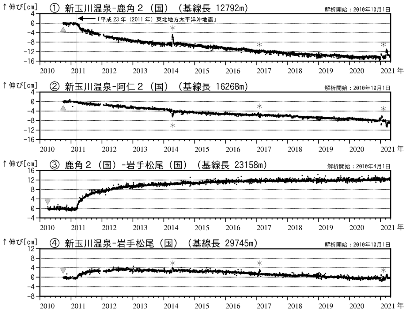
図4 秋田焼山 GNSS 基線長変化図（2010年4月～2021年4月）
