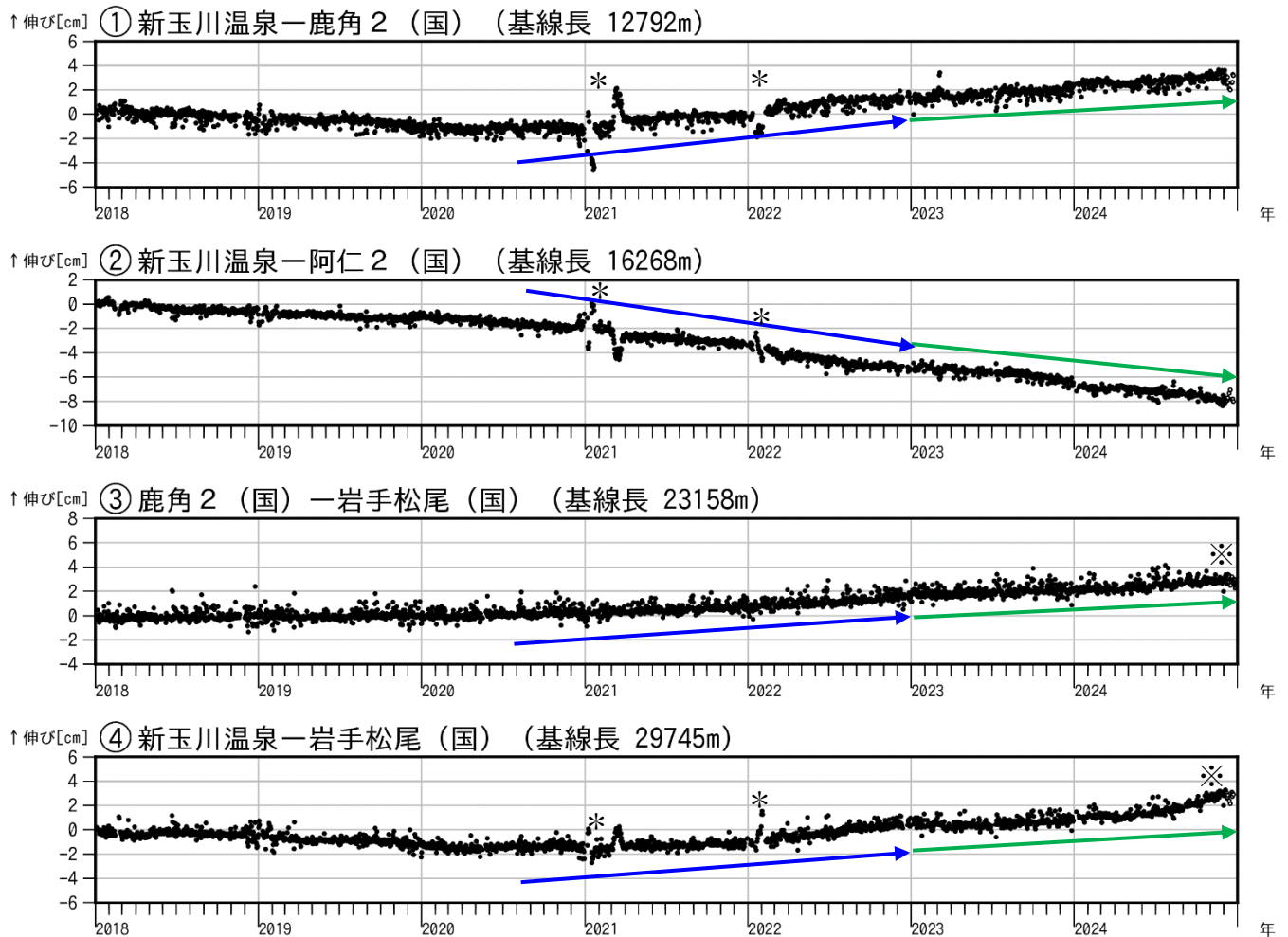
図10 秋田焼山 GNSS 基線長変化図（2018年1月～2024年12月）
