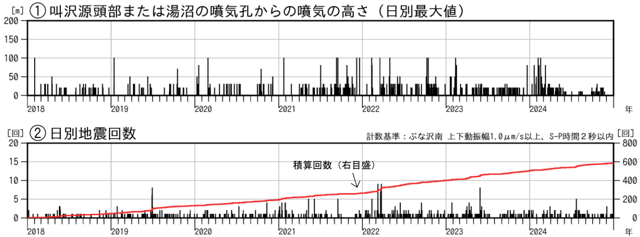
図9 秋田焼山 火山活動経過図（2018年1月～2024年12月）
