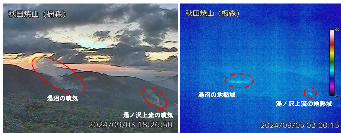
図2 秋田焼山 湯沼と湯ノ沢上流の状況と地表面温度分布（9月3日）
