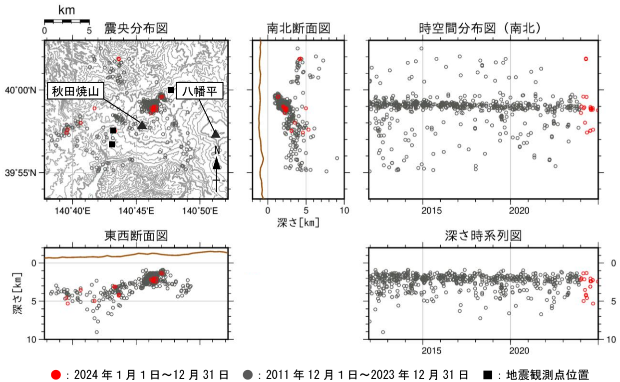
図8 秋田焼山 地震活動 (2011 年 12 月～2024 年 12 月)
