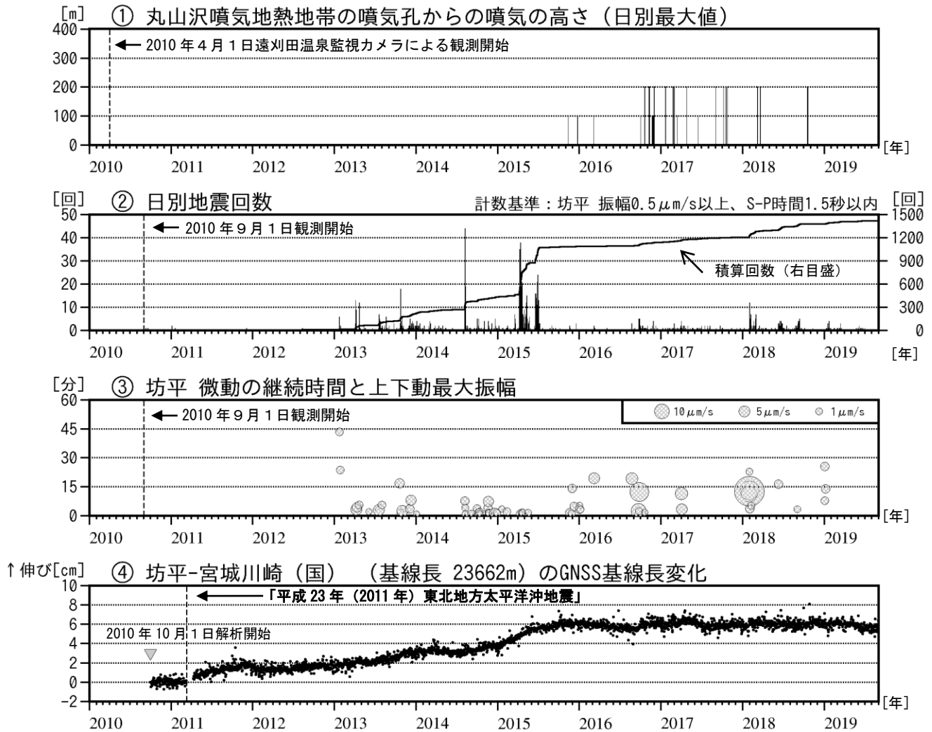
図2 蔵王山 火山活動経過図（2010年4月～2019年8月）
