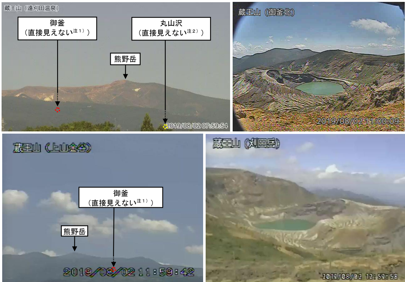
図1 蔵王山 山頂部の状況（8月2日）
