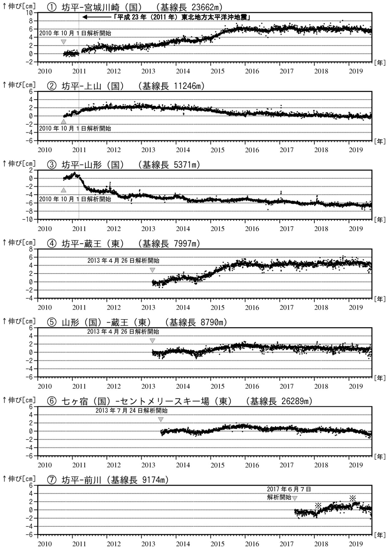
図 4 蔵王山 GNSS 基線長変化図 (2010 年 10 月～2019 年 8 月)
