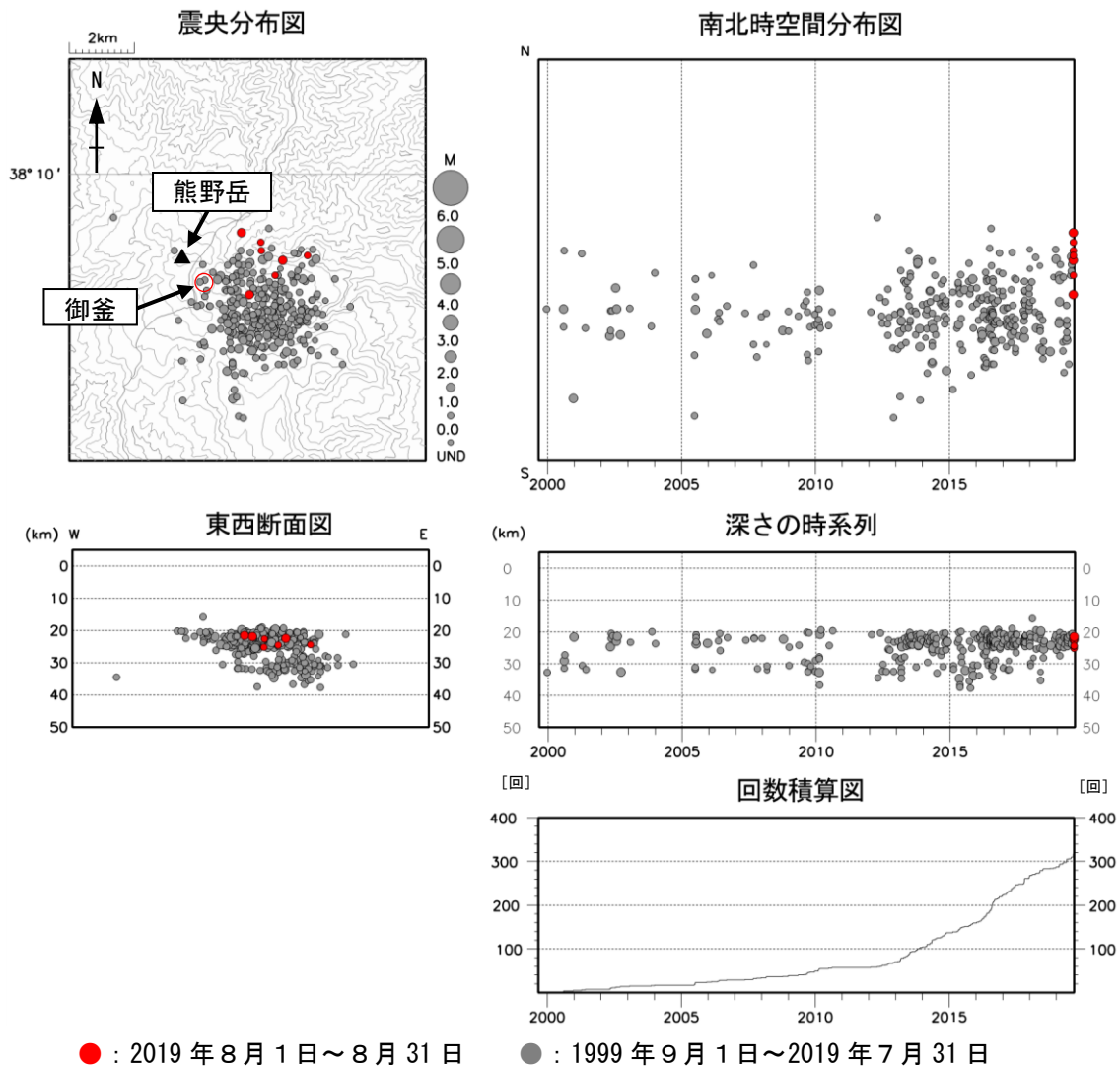
図 3 蔵王山 広域地震観測網による深部低周波地震活動（1999 年 9 月～2019 年 8 月）
