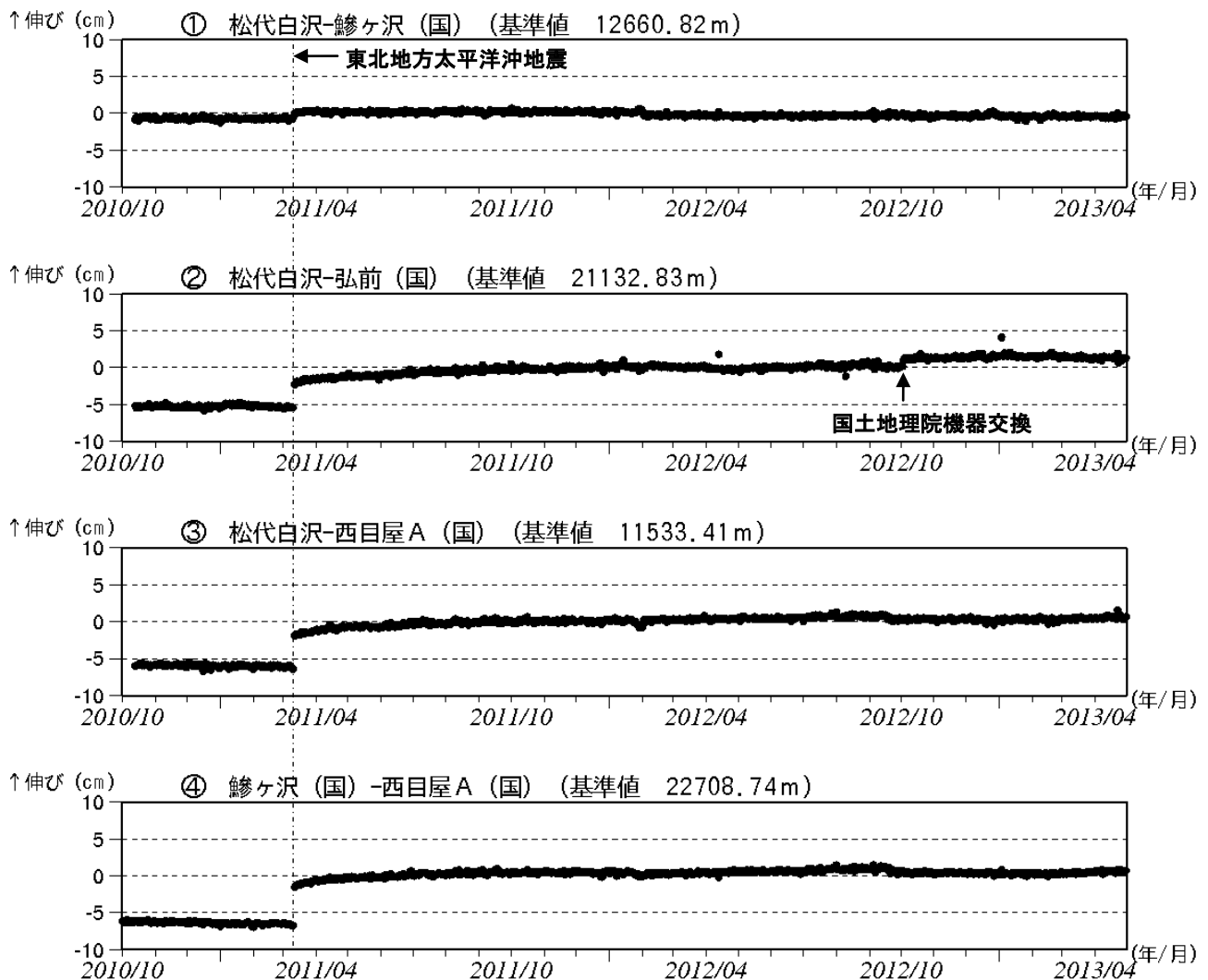
図3※ 岩木山 GPS 基線長変化図（2010年10月～2013年4月）
