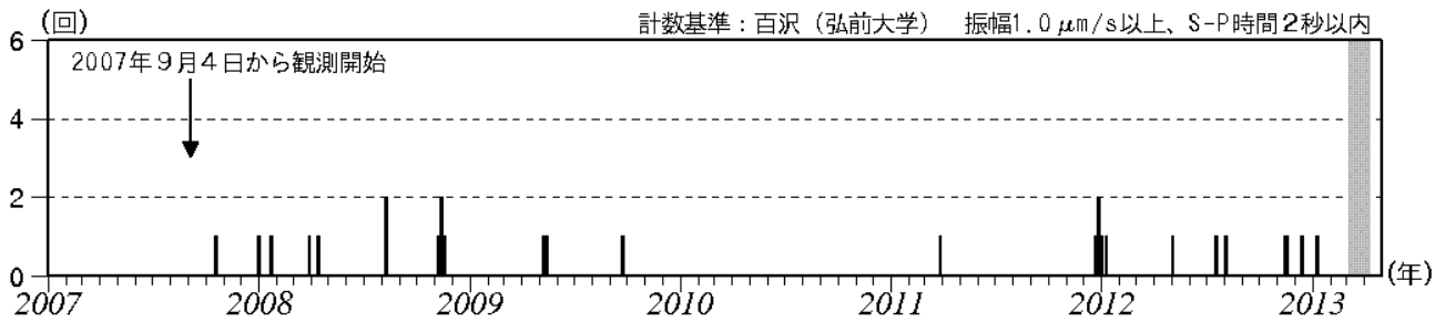
図2※ 岩木山 日別地震回数（2007年9月～2013年4月）
