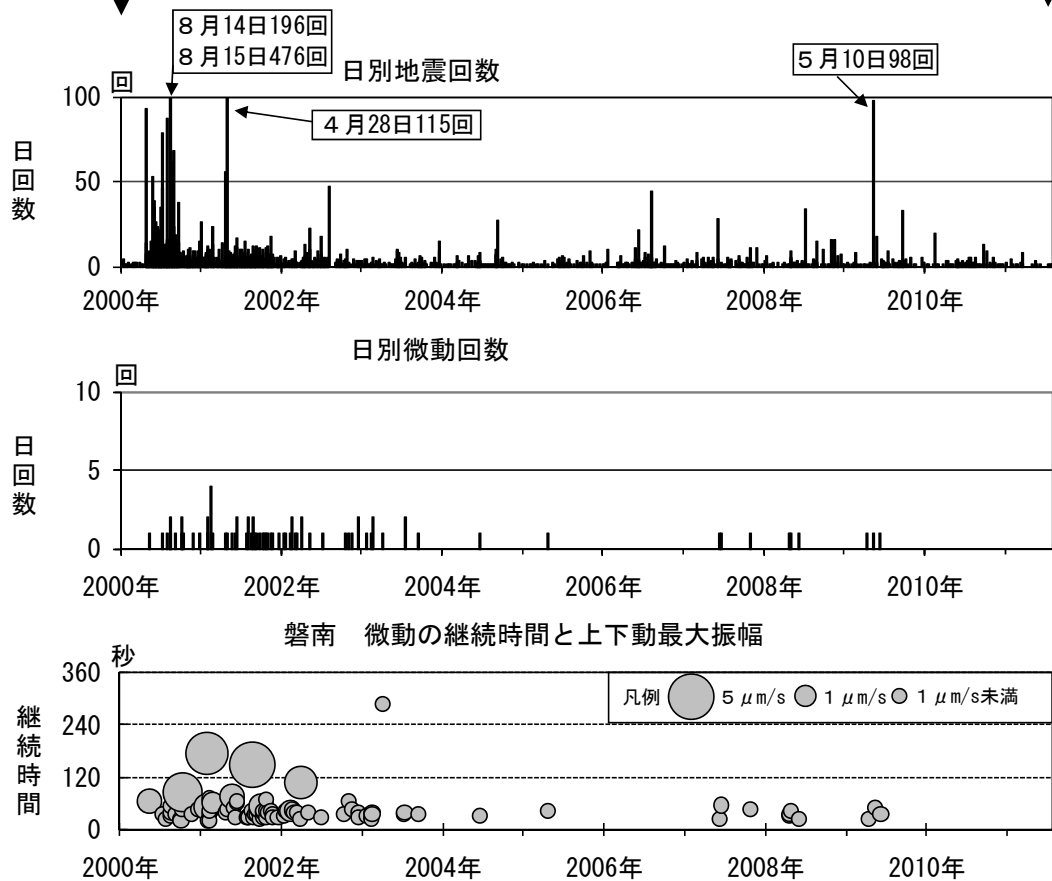
図5 磐梯山 最近の地震と微動の活動経過図（2000年1月～2011年7月）
