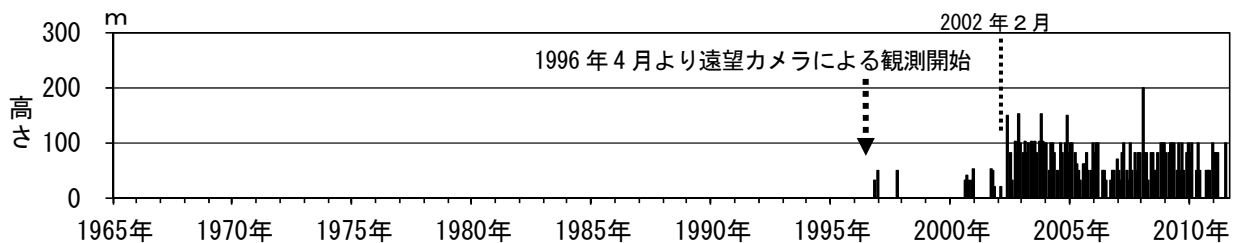
図3 磐梯山 月最大噴気高（1996年4月～2011年7月） 2002年2月以前は定時(09時、15時)及び随時観測による高さです。 2002年2月以後は全ての時間で観測したデータによる高さです。
