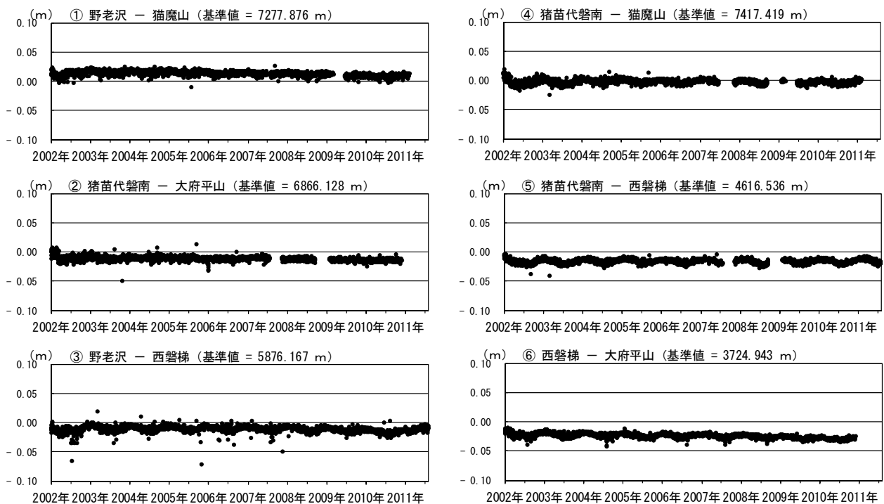
図 7 磐梯山 GPS 基線長変化図 (2002 年 1 月～2011 年 7 月)
