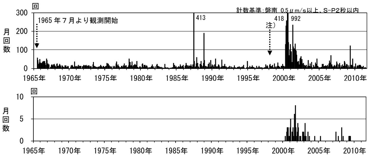
図4 磐梯山 上段：月別地震回数(1965年7月～2011年7月)
