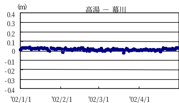
G P S 基線長変化図
