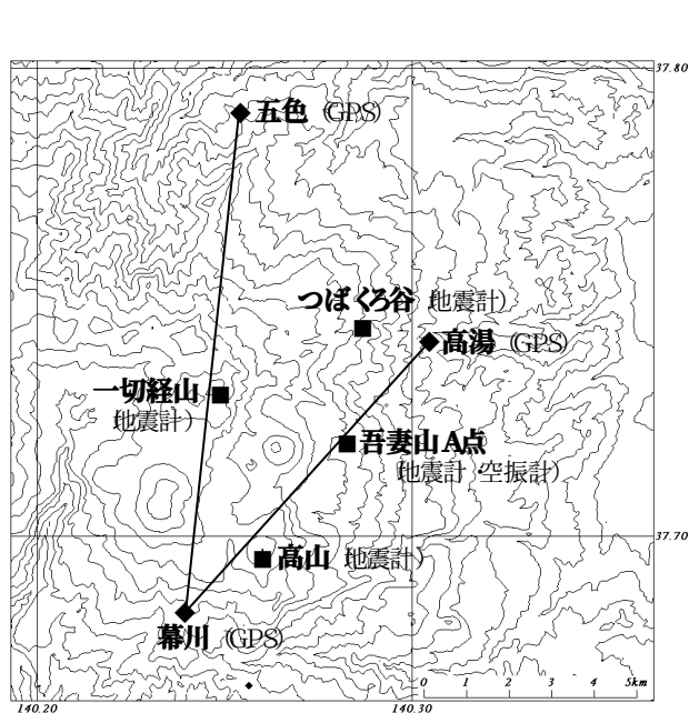
吾妻山観測点配置図
