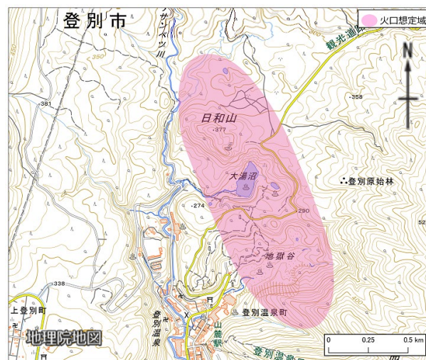
図8 倶多楽 火口想定域
