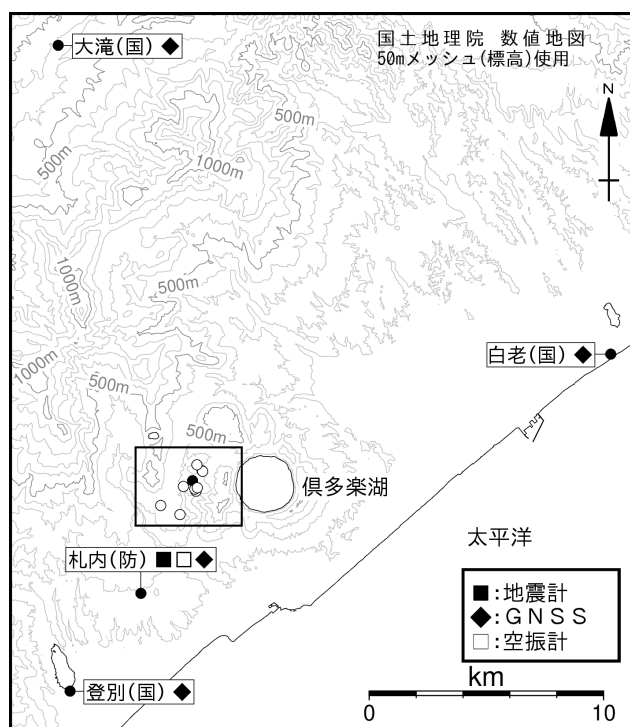
図9 倶多楽 観測点配置図
