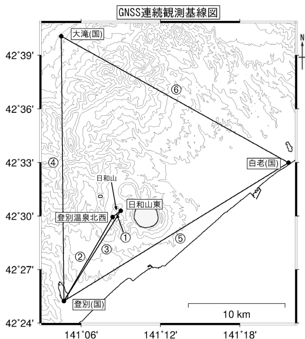
図7 倶多楽 GNSS連続観測の観測点配置図
