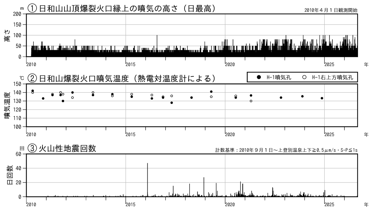
図2 倶多楽 火山活動経過図（2010年1月～2026年9月）
