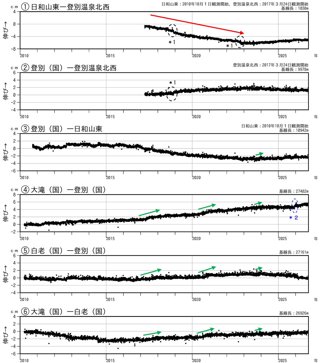
図6 倶多楽 GNSS連続観測による基線長変化（2010年4月～2026年9月）
