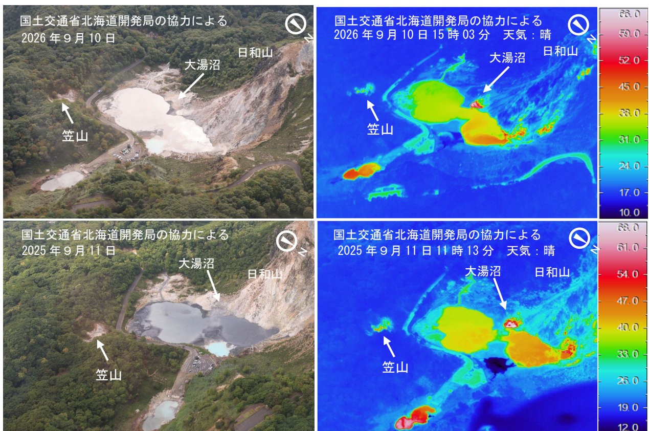
図4 倶多楽 赤外熱映像装置による日和山・大湯沼・笠山周辺の地表面温度分布 上：北東側上空（図3の①）から撮影 下：東側上空（図3の②）から撮影 ・過去の観測（2025年9月）と比較して、日和山や大湯沼周辺、笠山の地表面温度分布に特段の変化は認められませんでした。
