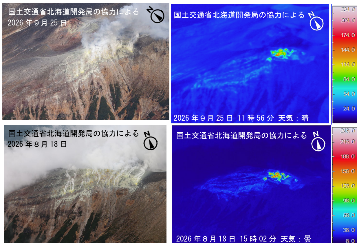
図7 十勝岳 赤外熱映像装置による振子沢噴気孔群の地表面温度分布 上：南西側上空（図5の②）から撮影 下：南側上空（図5の③）から撮影 ・振子沢噴気孔群において引き続き地表面温度が高い状態であることを確認しました。
