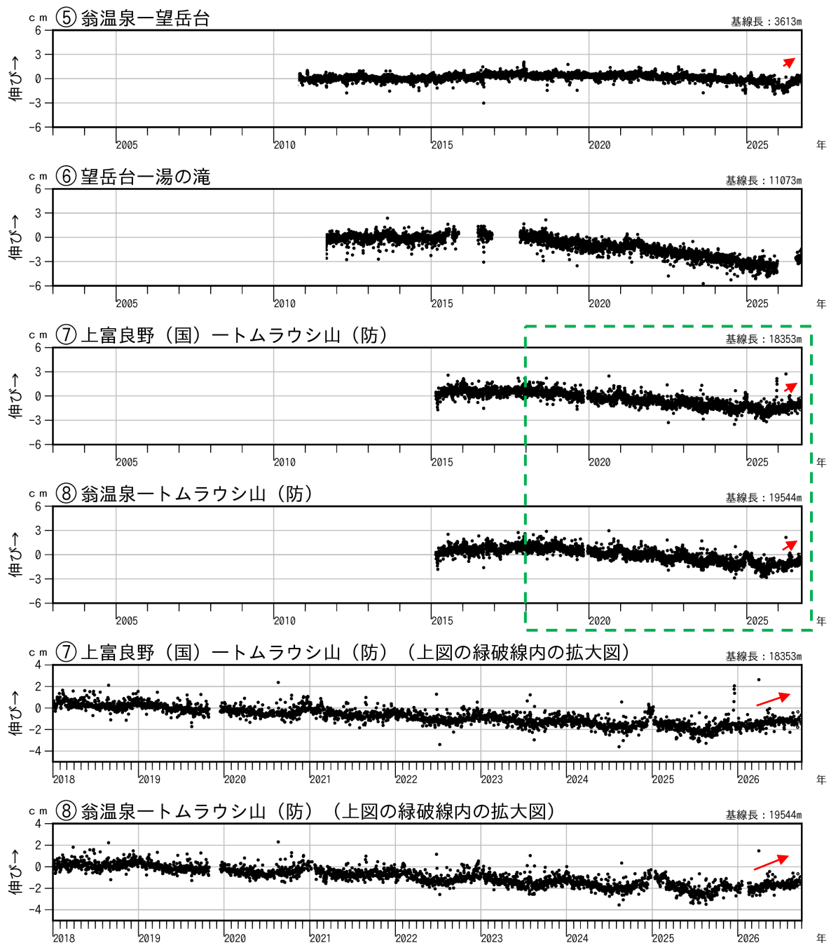
図12-2 十勝岳 GNSS連続観測による基線長変化（2003年5月～2026年9月）
