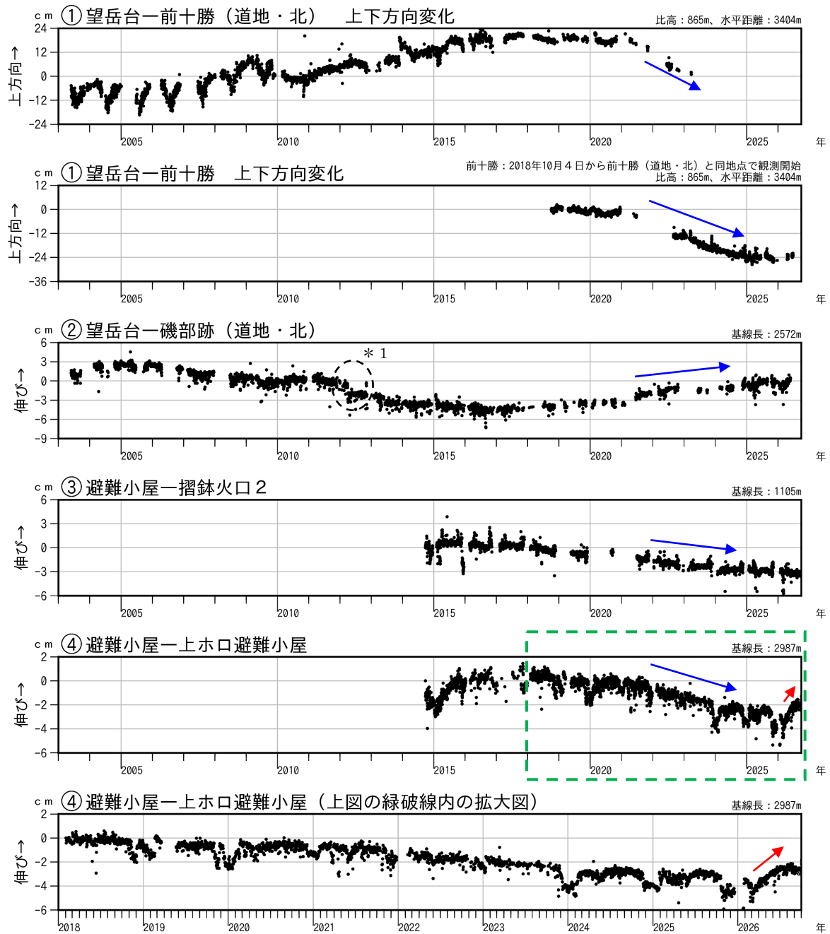
図12-1 十勝岳 GNSS連続観測による上下方向変化及び基線長変化（2003年5月～2026年9月）
