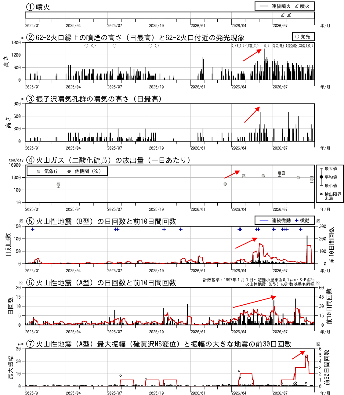
図3 十勝岳 火山活動経過図（2025年1月～2026年9月）
