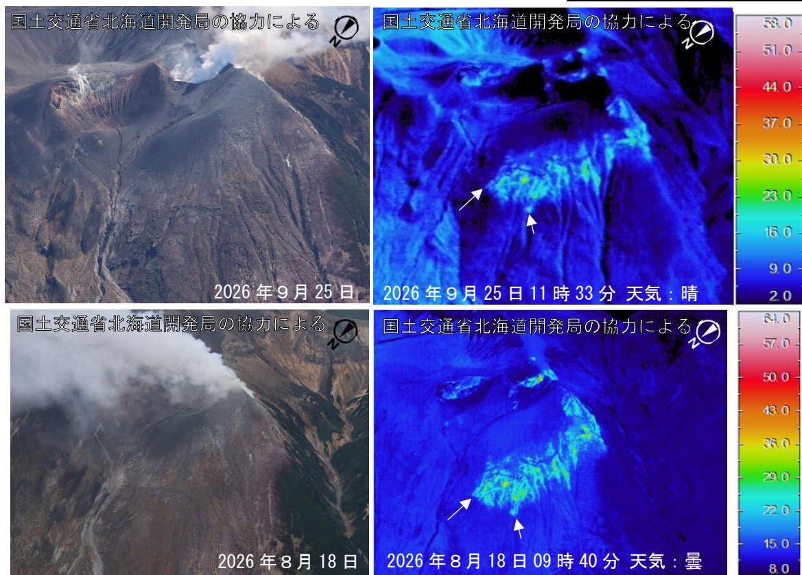
図8 十勝岳 赤外熱映像装置による前十勝北西側斜面の地表面温度分布
