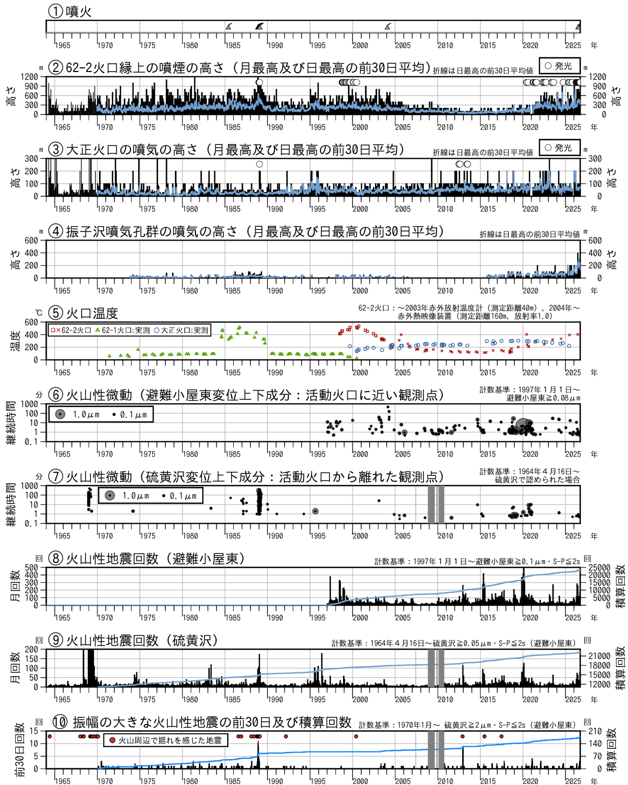
図1 十勝岳 火山活動経過図（1964年1月～2026年9月）
