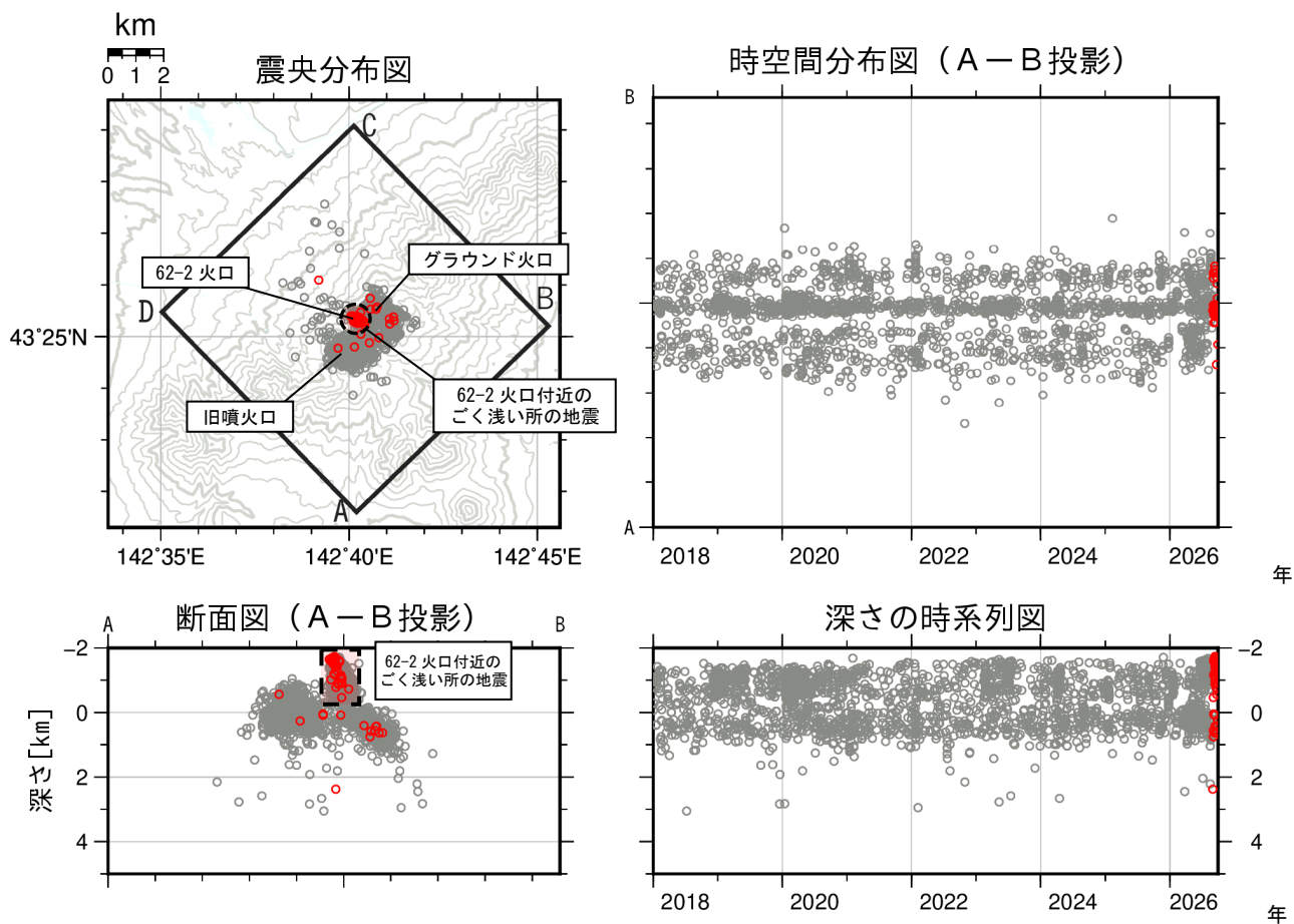
図10 十勝岳 火山性地震の震源分布（2018年1月～2026年9月）
