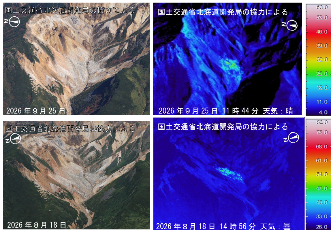
図9 十勝岳 赤外熱映像装置による旧噴火口の地表面温度分布
