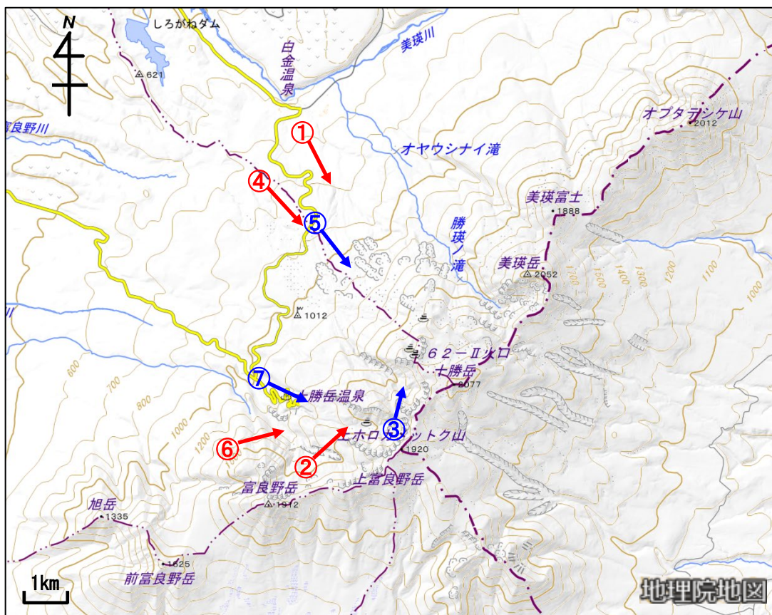
図5 十勝岳 写真及び赤外熱画像の撮影方向（矢印）
