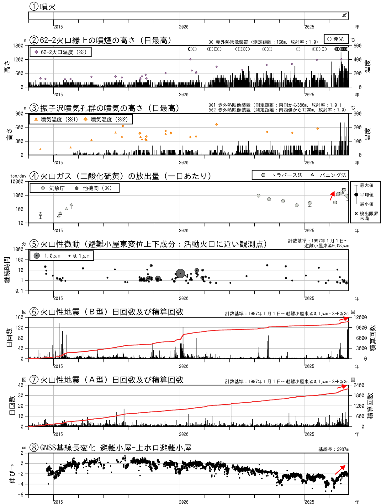
図2 十勝岳 火山活動経過図（2014年1月～2026年9月）
