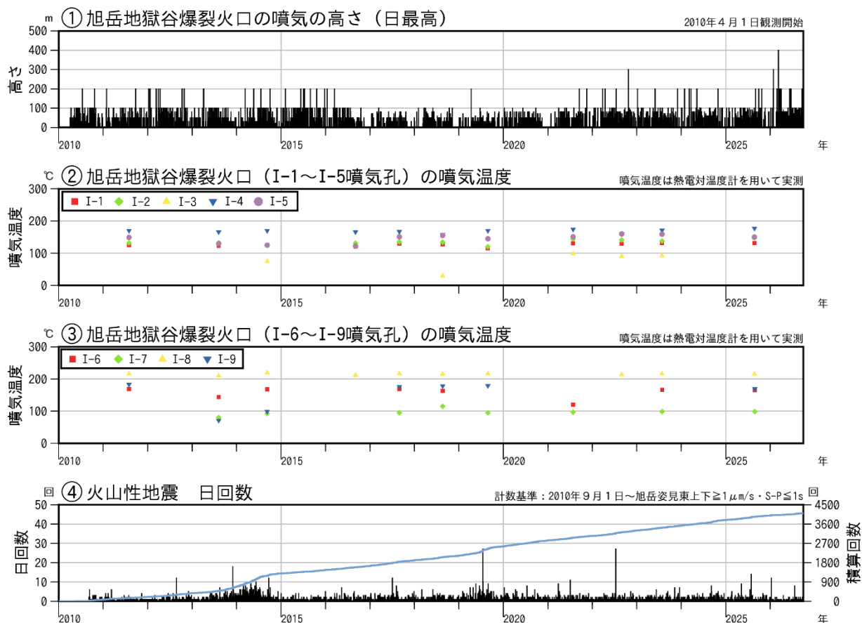
図2 大雪山 火山活動経過図（2010年4月～2026年9月）
