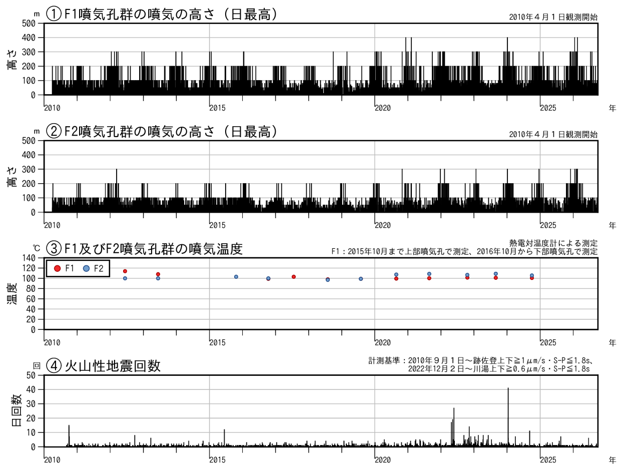
図1 アトサヌプリ 火山活動経過図（2010年4月～2026年9月）
