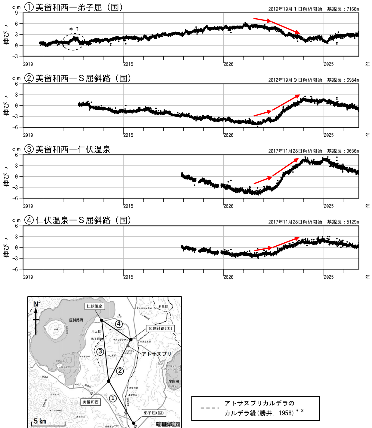
図4 アトサヌプリ GNSS連続観測による基線長変化(2010年10月～2026年9月)及び観測点配置図 冬季に凍上や積雪の影響によると考えられる変動がみられる基線があります。
