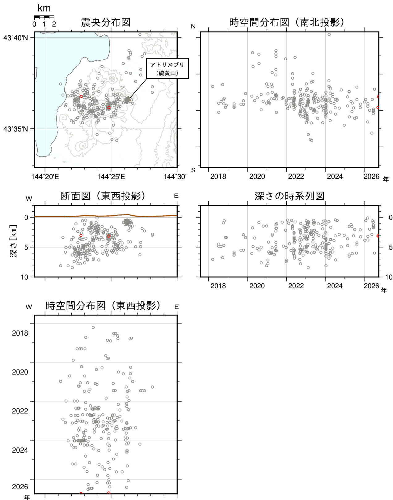
図3 アトサヌプリ 火山性地震の震源分布（2017年8月～2026年9月）
