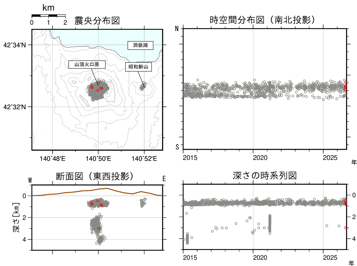
図3 有珠山 火山性地震の震源分布（2015年1月～2026年8月） ○：2015年1月～2026年7月の震源 ○：2026年8月の震源
