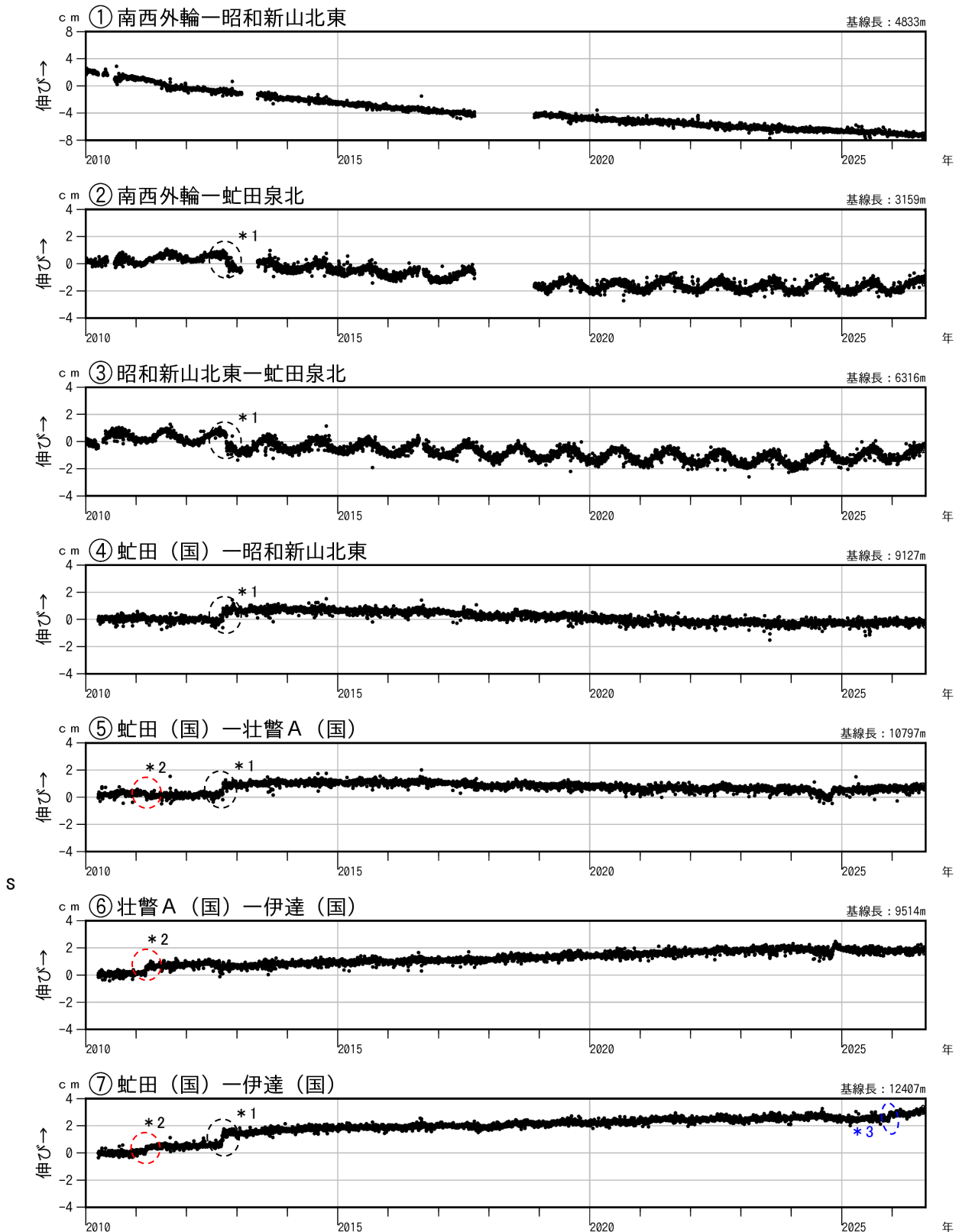
図4 有珠山 GNSS連続観測による基線長変化（2010年1月～2026年8月）
