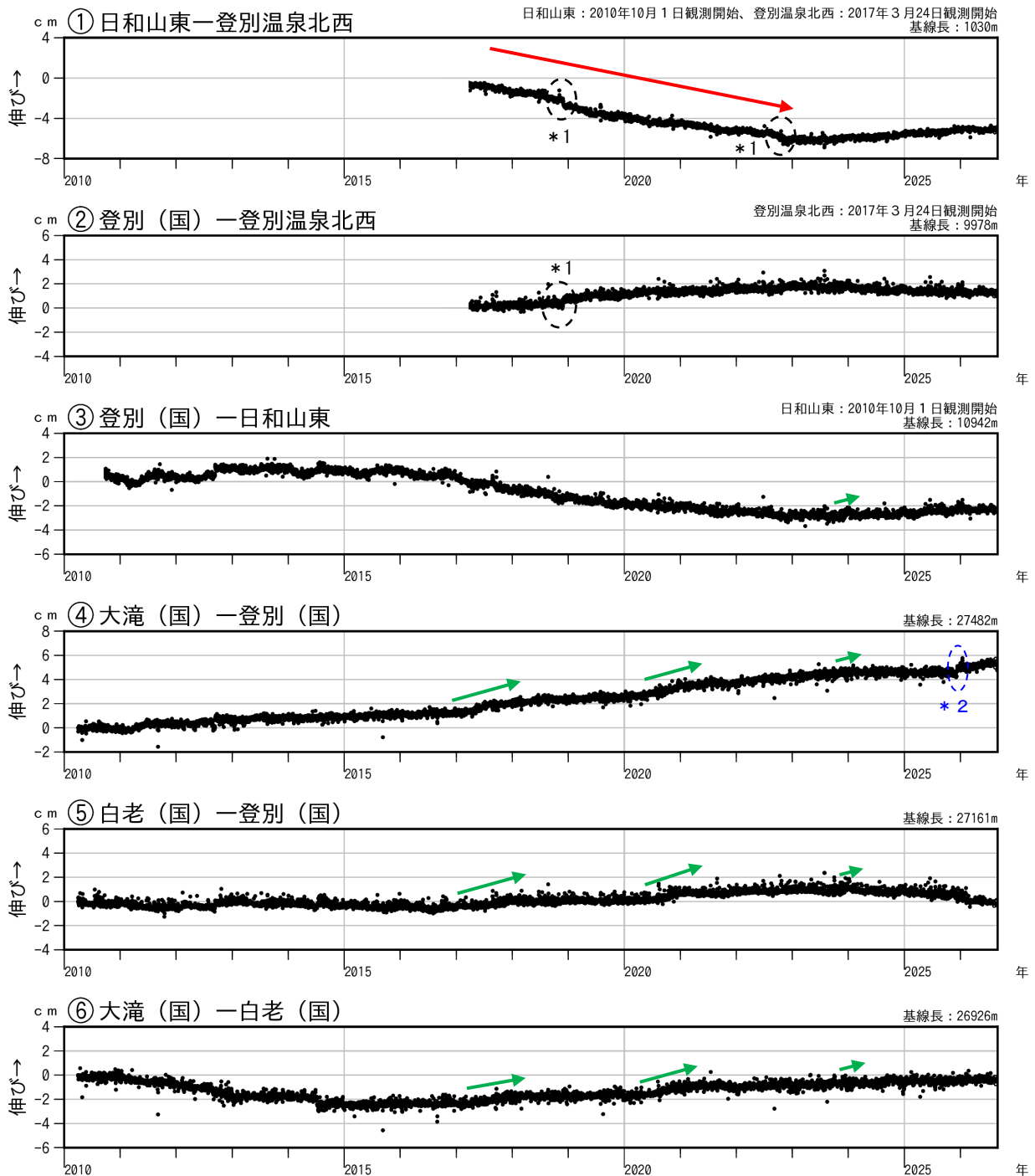
図3 倶多楽 GNSS連続観測による基線長変化（2010年4月～2026年8月）
