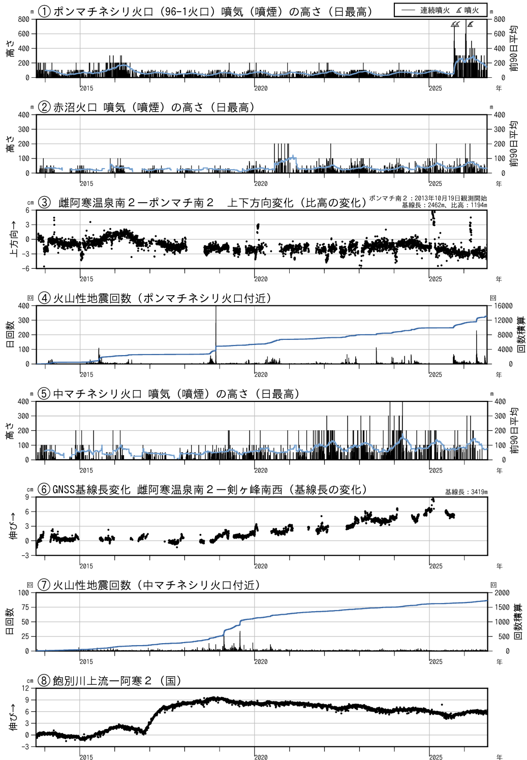
図5 雌阿寒岳 火口別の活動経過図（2013年10月～2026年8月）
