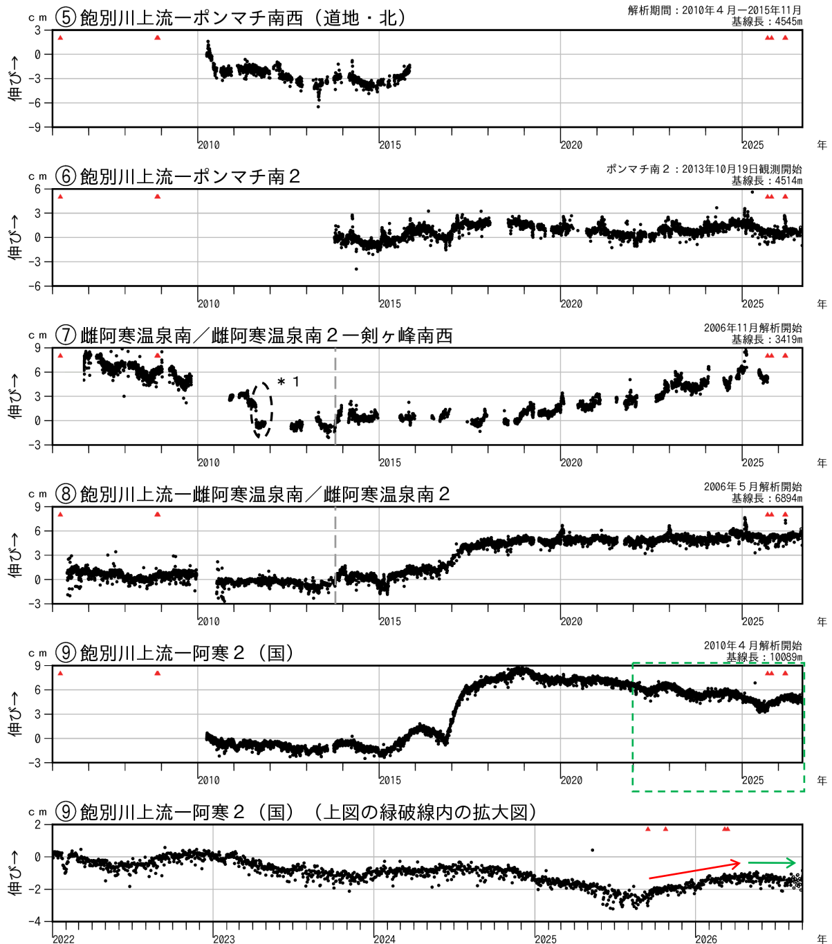
図7-2 雌阿寒岳 GNSS連続観測による基線長の変化（2006年4月～2026年8月）
