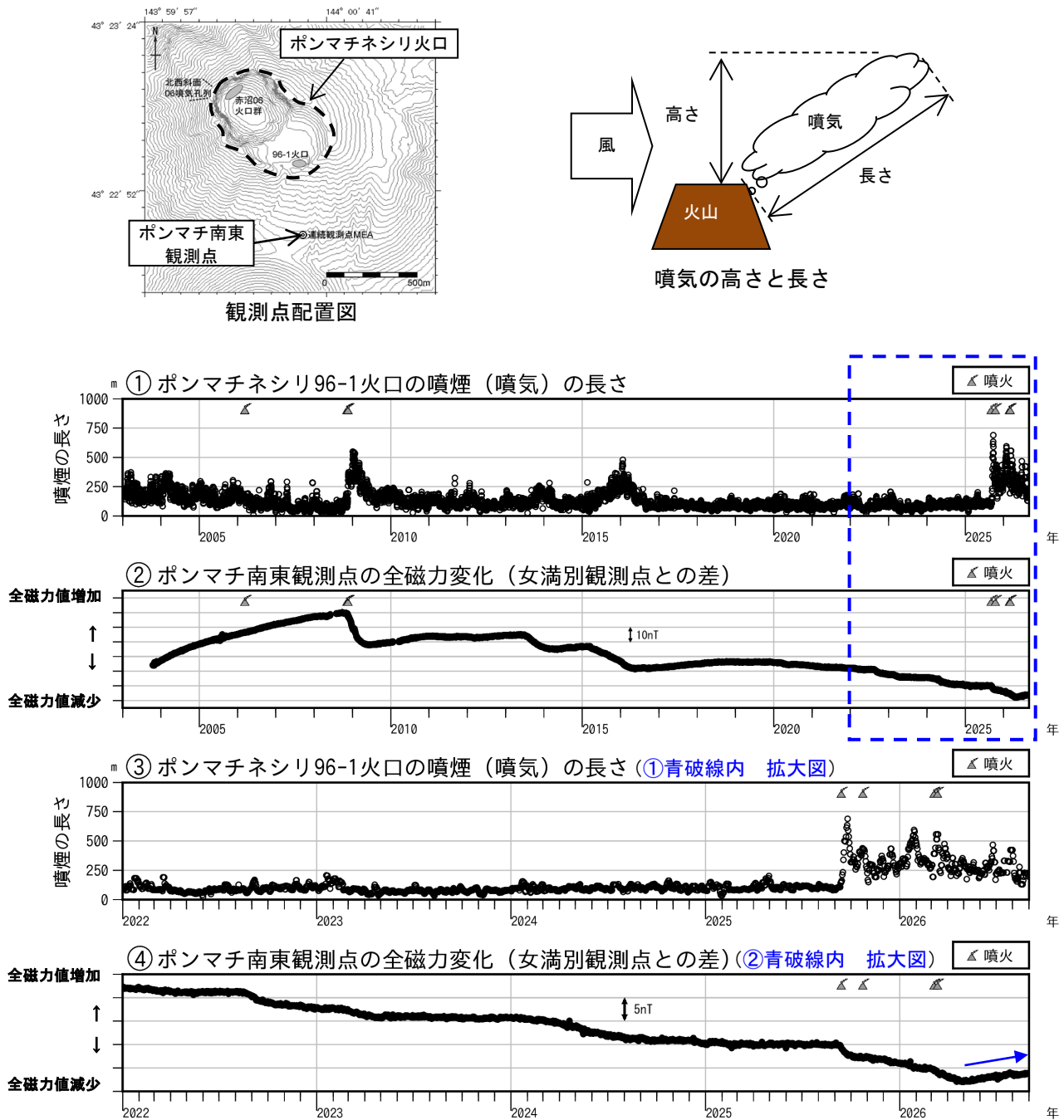
図6 雌阿寒岳 ポンマチネシリ96-1火口の噴気（噴煙）の長さ、全磁力値の経過及び全磁力観測点配置図（2003年～2026年8月）
