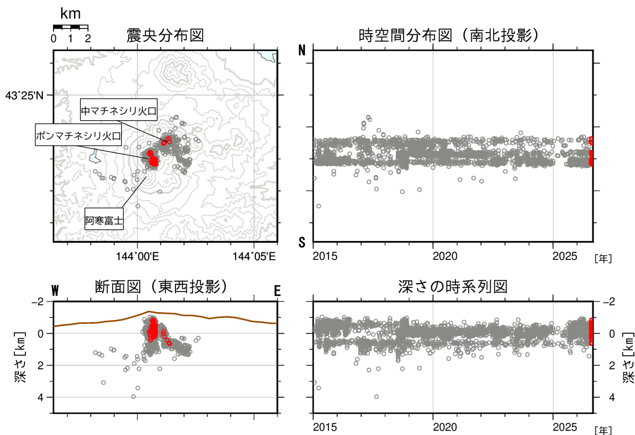
図4 雌阿寒岳 火山性地震の震源分布（2015年1月～2026年8月） ○：2015年1月～2026年7月の震源 ○：2026年8月の震源
