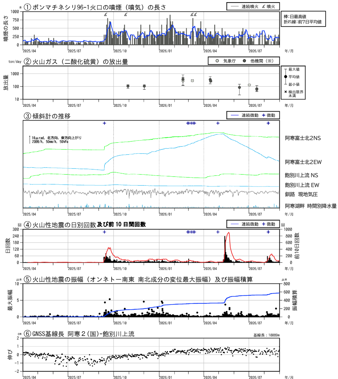
図2 雌阿寒岳 短期の火山活動経過図（2025年4月～2026年8月）
