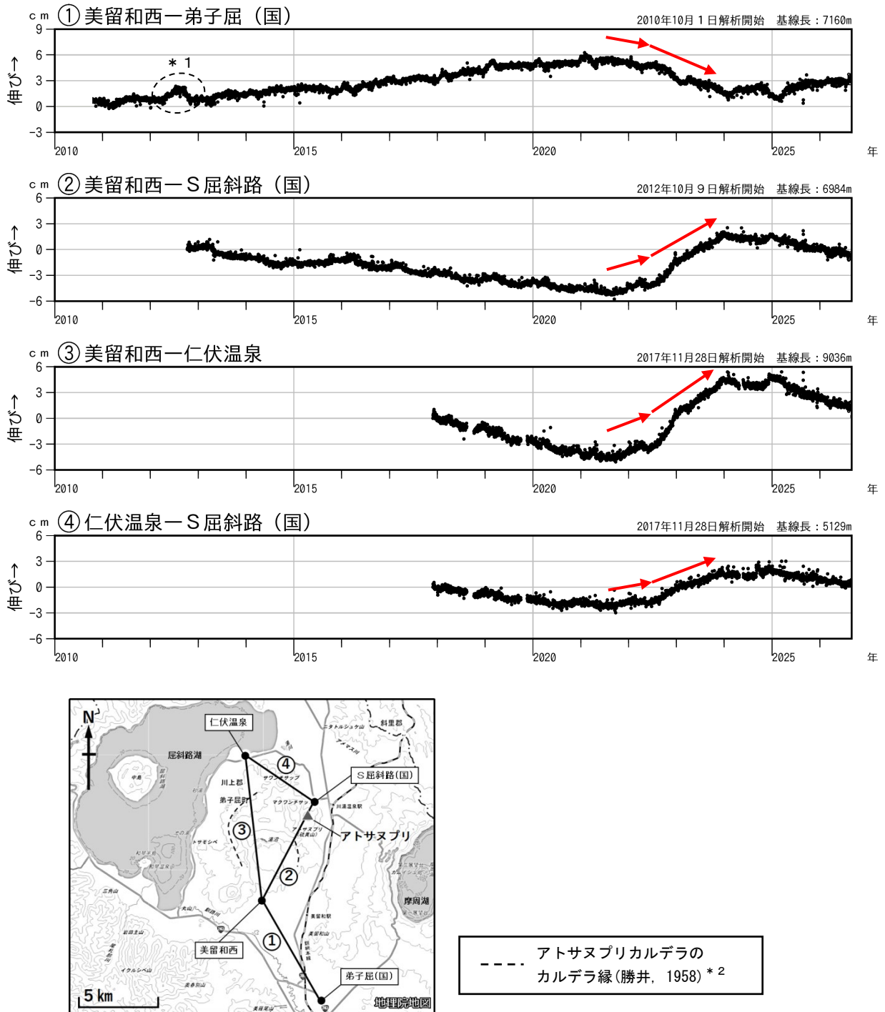
図4 アトサヌプリ GNSS連続観測による基線長変化（2010年10月～2026年8月）及び観測点配置図 冬季に凍上や積雪の影響によると考えられる変動がみられる基線があります。
