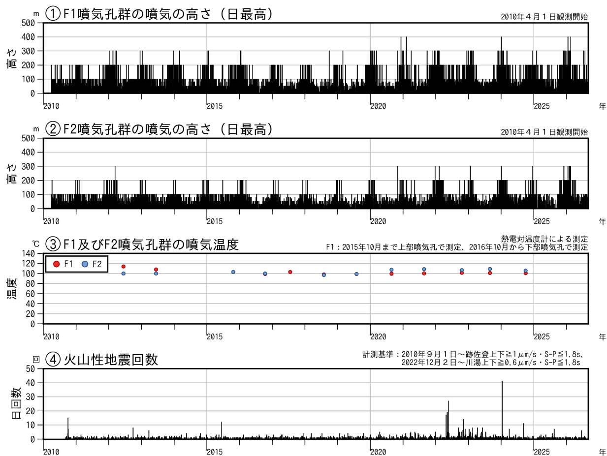
図1 アトサヌプリ 火山活動経過図（2010年4月～2026年8月）
