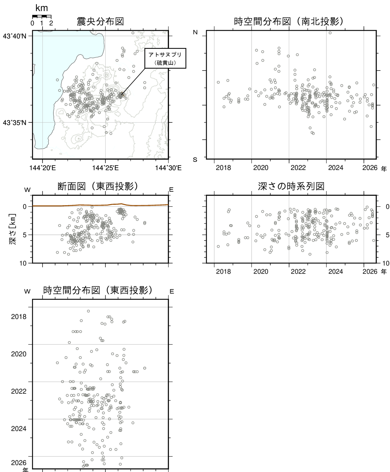
図3 アトサヌプリ 火山性地震の震源分布（2017年8月～2026年8月）
