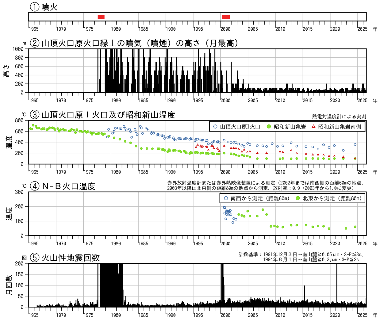
図1 有珠山 火山活動経過図（1965年1月～2026年7月）
