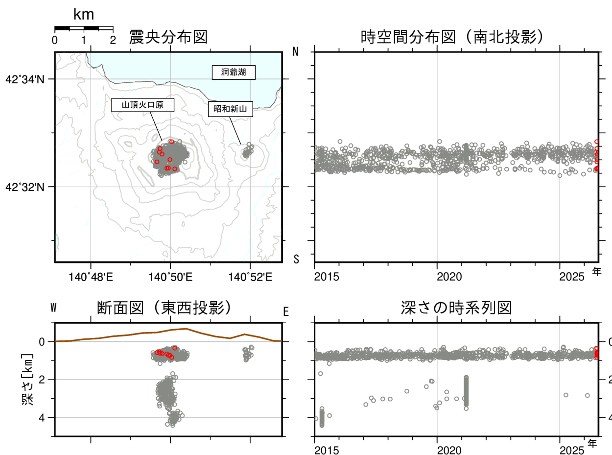
図3 有珠山 火山性地震の震源分布（2015年1月～2026年7月） ○：2015年1月～2026年6月の震源 ●：2026年7月の震源
