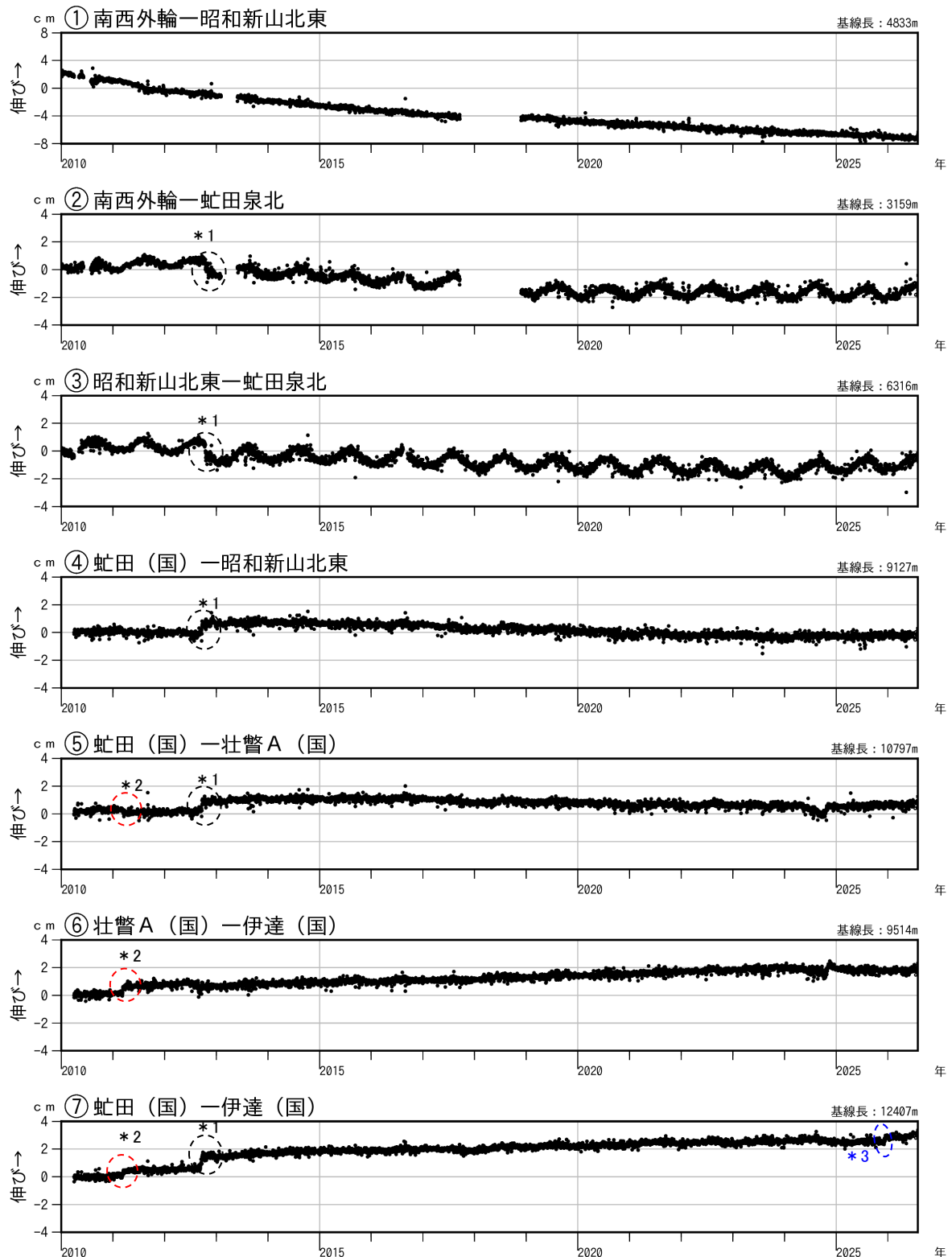
図4 有珠山 GNSS連続観測による基線長変化（2010年1月～2026年7月）
