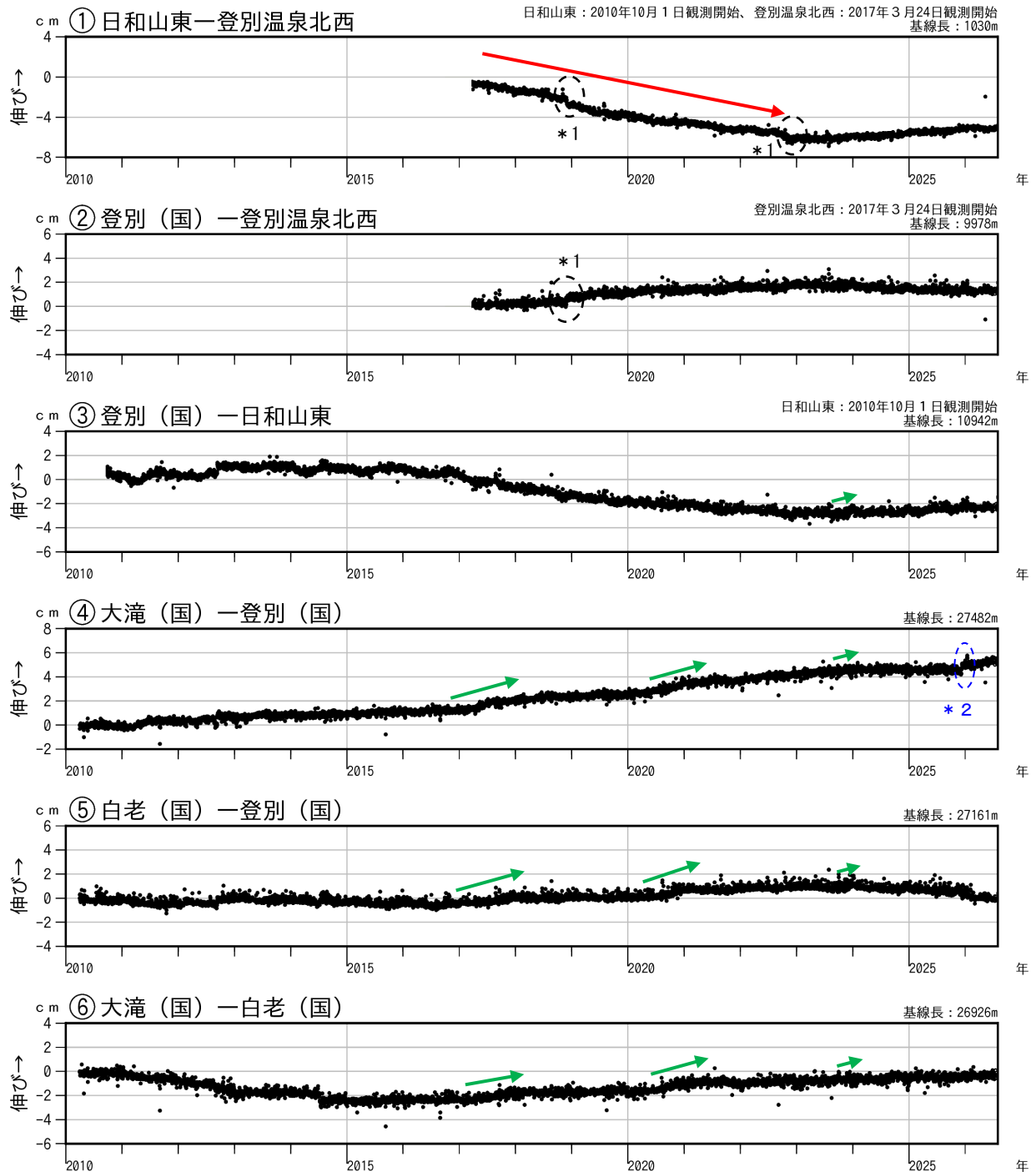
図3 倶多楽 GNSS連続観測による基線長変化（2010年4月～2026年7月）
