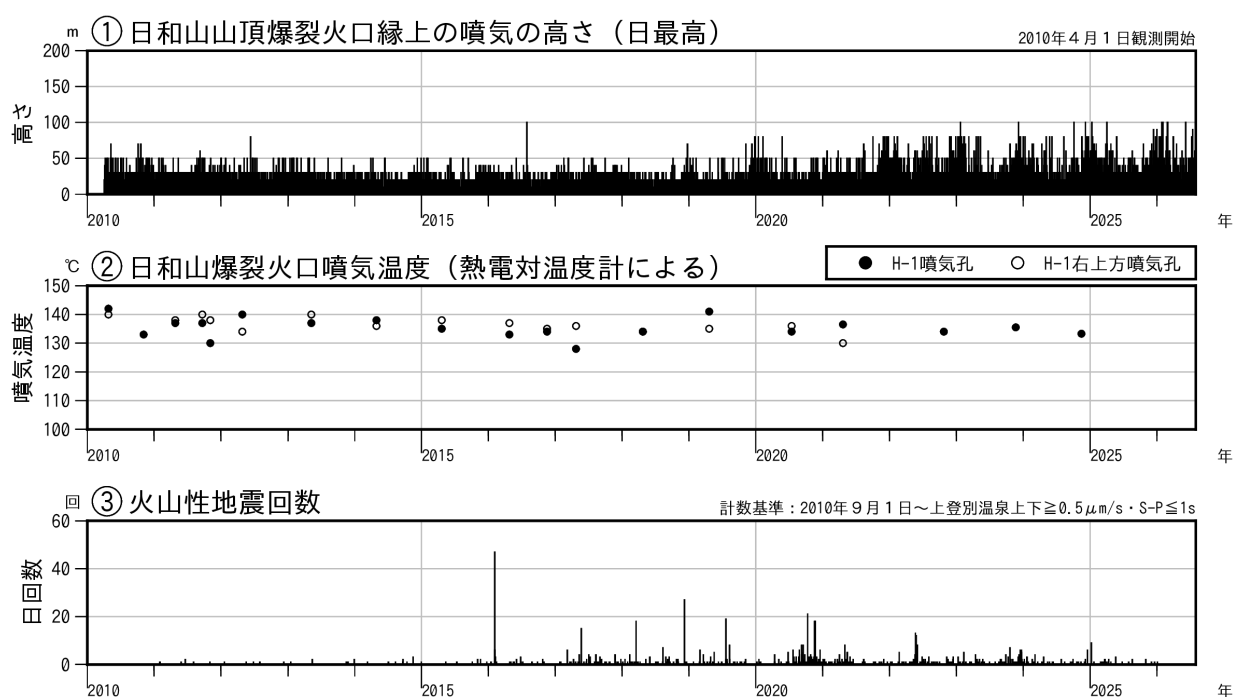
図2 倶多楽 火山活動経過図（2010年1月～2026年7月）
