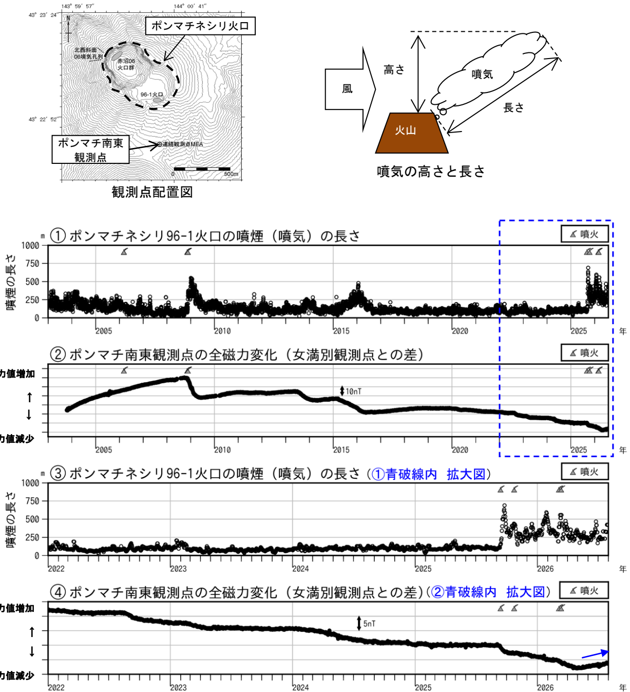
図6 雌阿寒岳 ポンマチネシリ96-1火口の噴気（噴煙）の長さ、全磁力値の経過及び全磁力観測点配置図（2003年～2026年7月）
