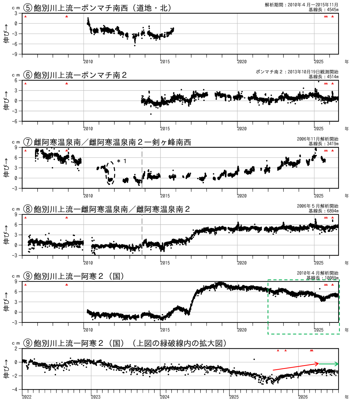
図7-2 雌阿寒岳 GNSS連続観測による基線長の変化（2006年4月～2026年7月）
