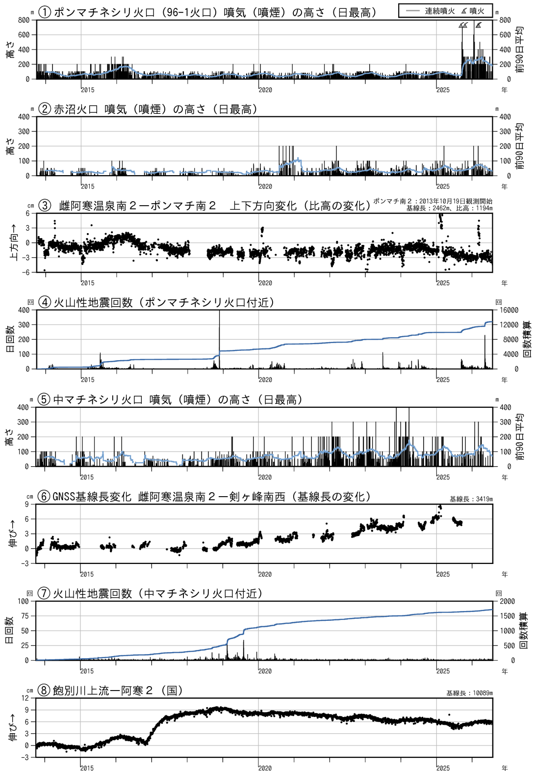
図5 雌阿寒岳 火口別の活動経過図（2013年10月～2026年7月）
