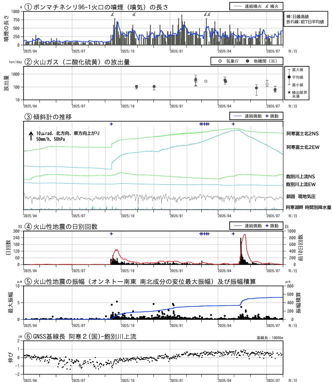
図2 雌阿寒岳 短期の火山活動経過図（2025年4月～2026年7月）
