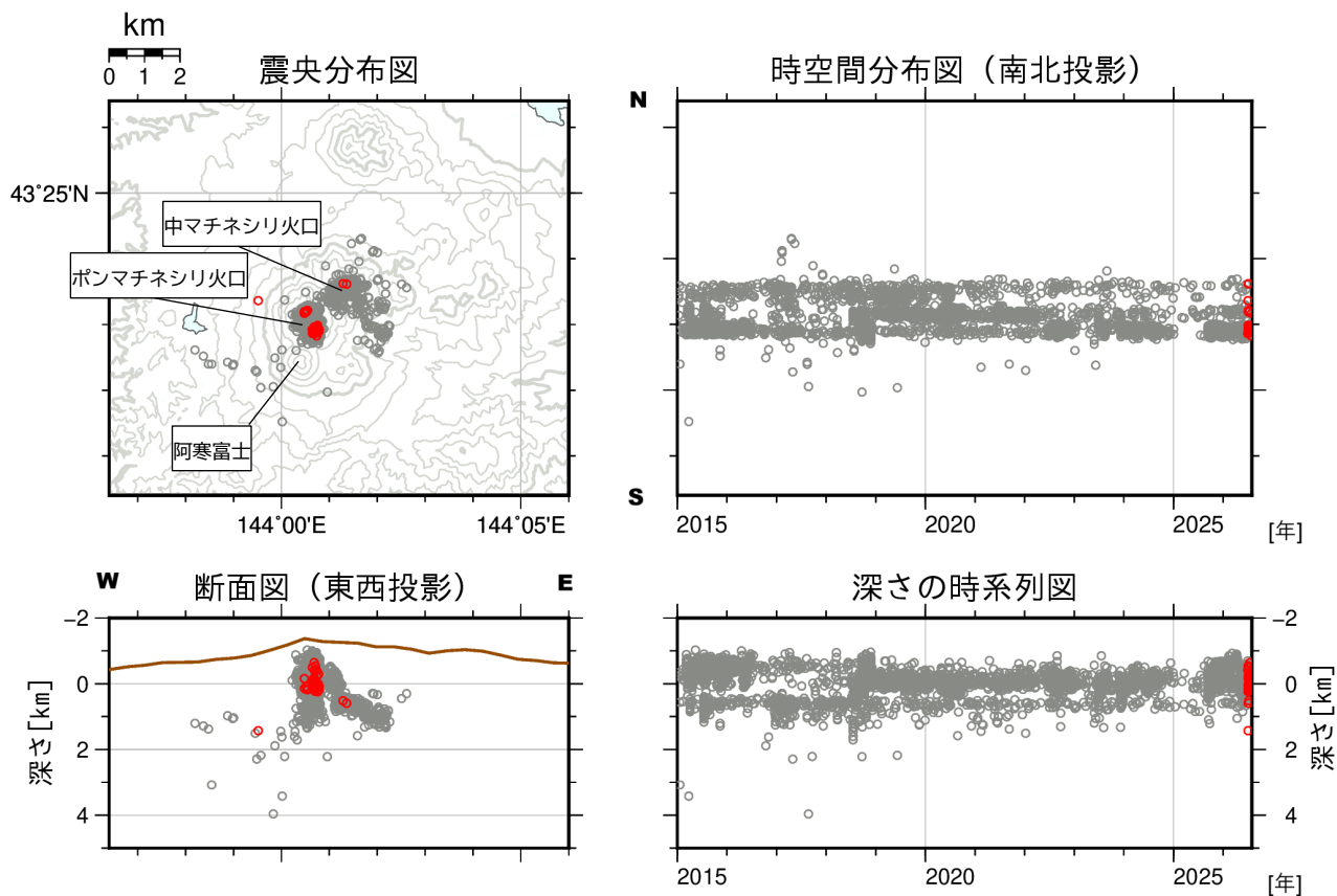
図4 雌阿寒岳 火山性地震の震源分布（2015年1月～2026年7月） ○：2015年1月～2026年6月の震源 ○：2026年7月の震源
