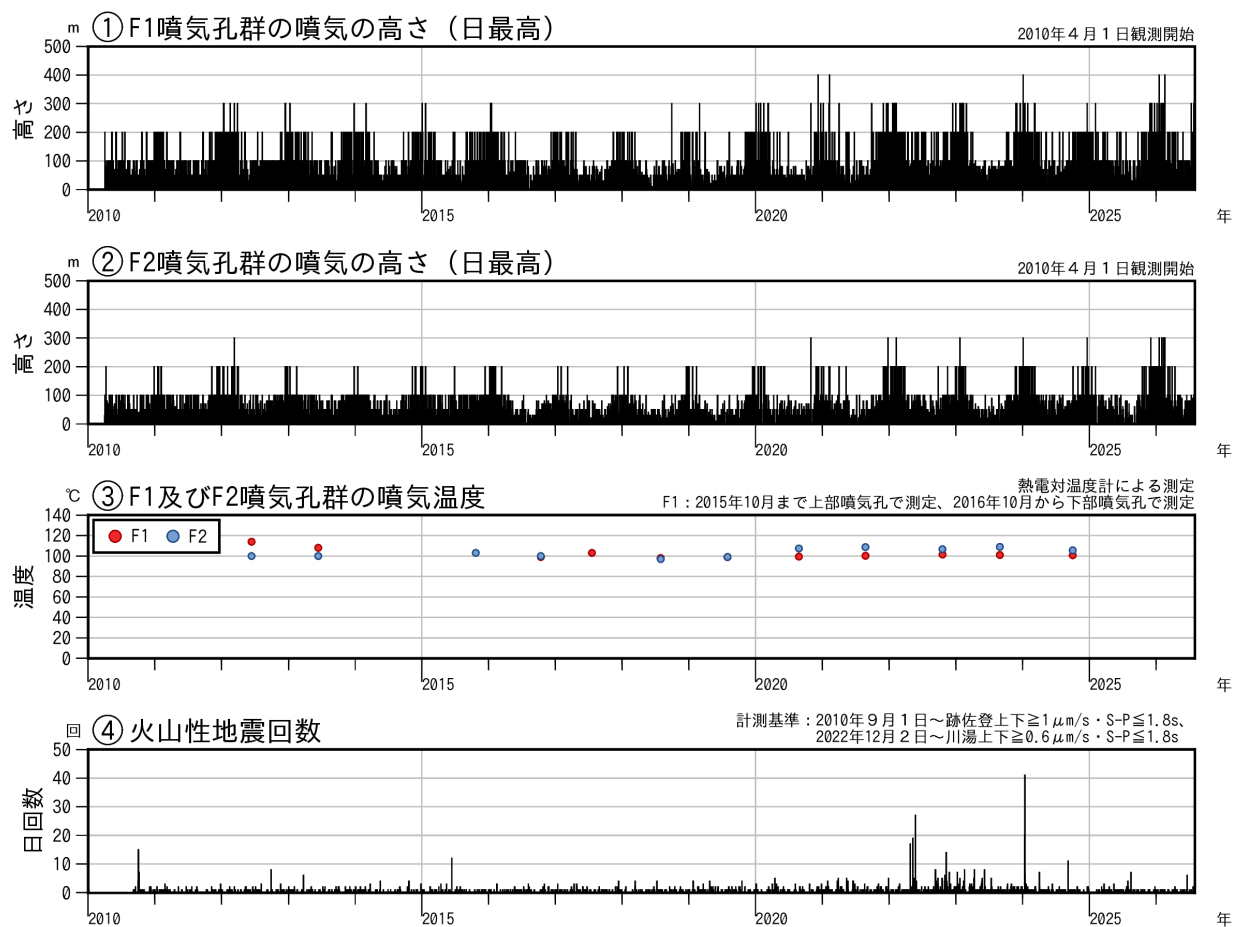
図1 アトサヌプリ 火山活動経過図（2010年4月～2026年7月）
