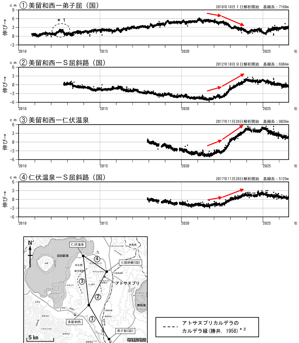
図4 アトサヌプリ GNSS連続観測による基線長変化（2010年10月～2026年7月）及び観測点配置図 冬季に凍上や積雪の影響によると考えられる変動がみられる基線があります。
