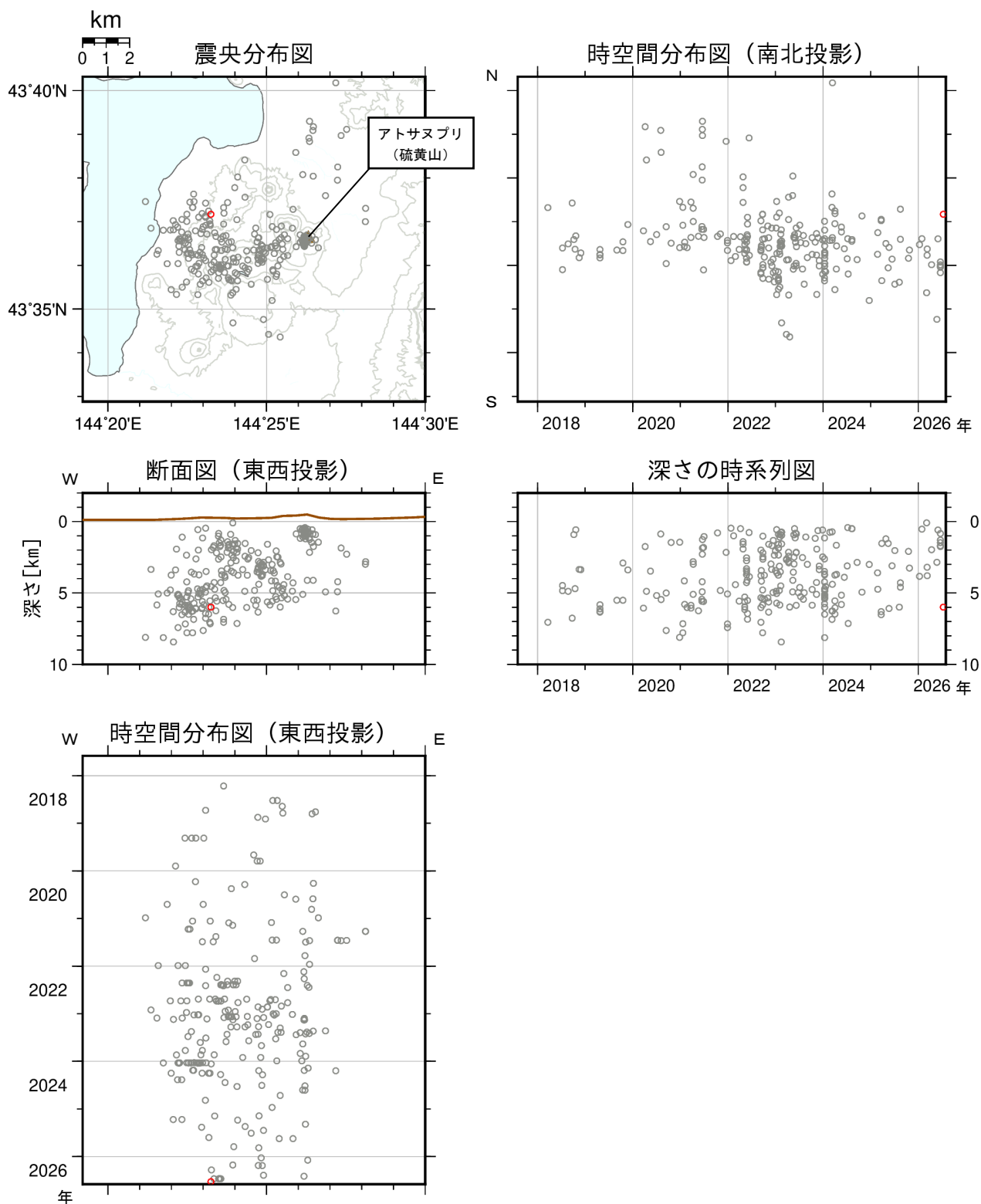
図3 アトサヌプリ 火山性地震の震源分布（2017年8月～2026年7月） ○：2017年8月～2026年6月の震源 ●：2026年7月の震源
