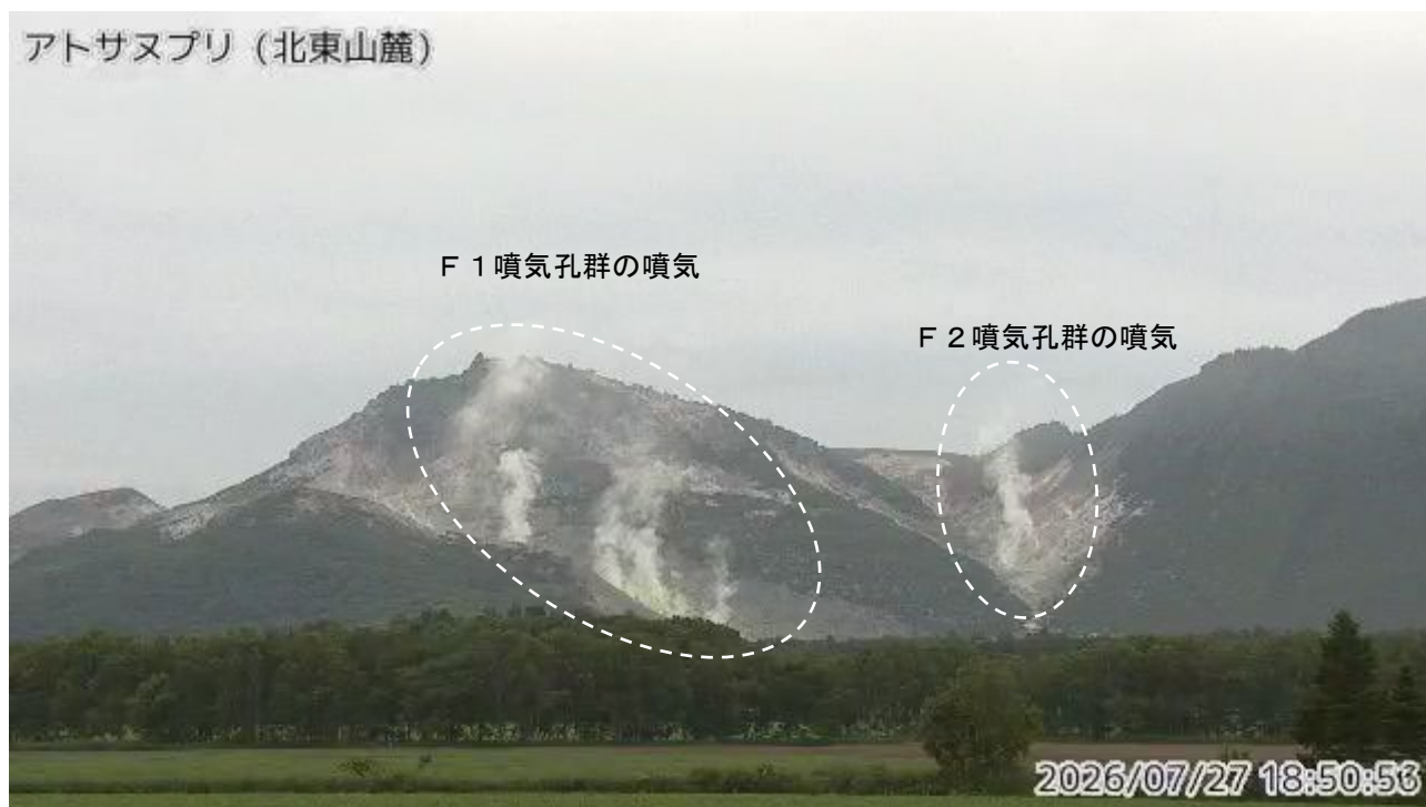
図2 アトサヌプリ 北東側から見たF 1及びF 2噴気孔群の状況（北東山麓監視カメラによる）
