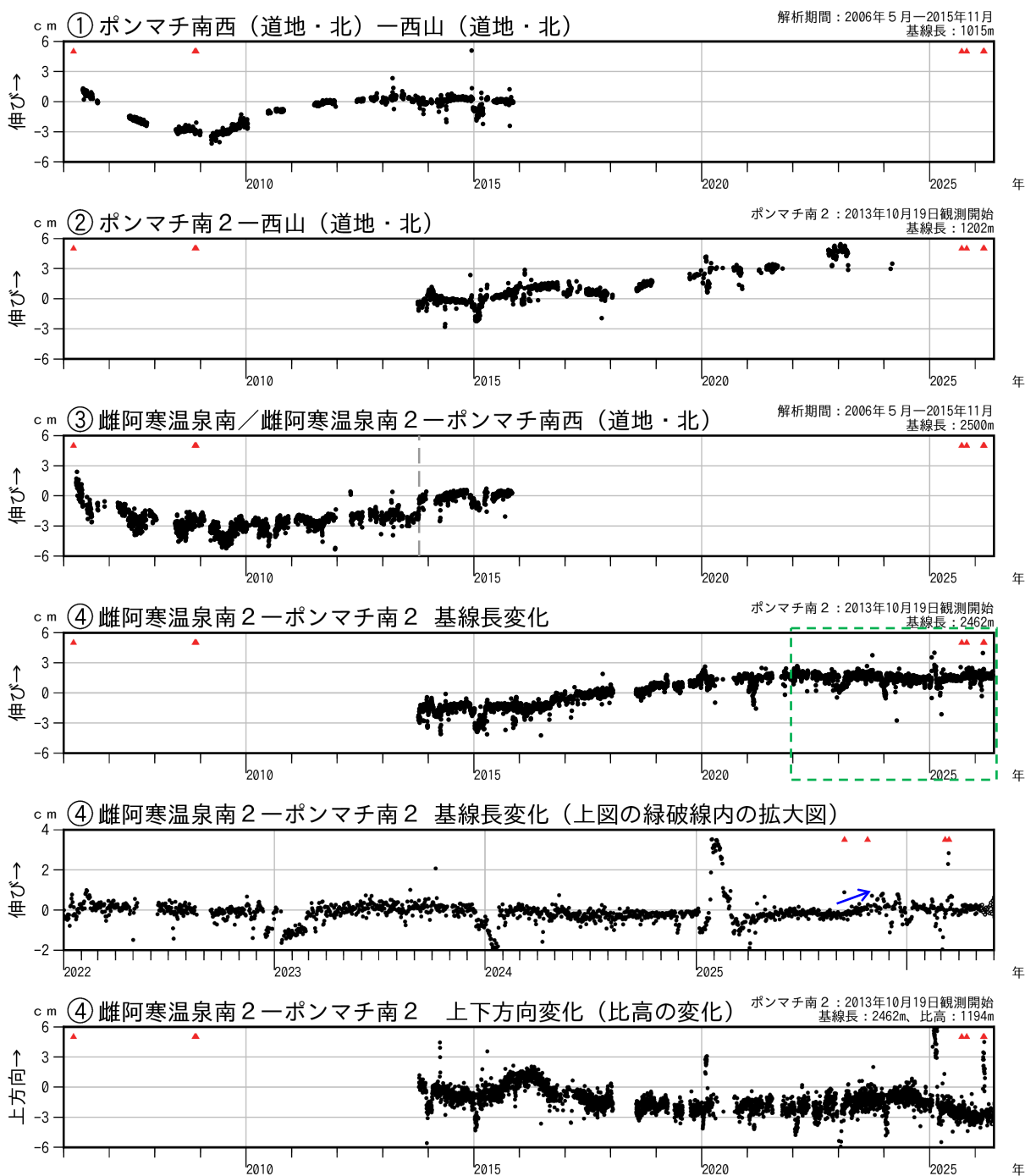
図10-1 雌阿寒岳 GNSS連続観測による基線長及び比高の変化（2006年4月～2026年5月） ・グラフ①～④はGNSS連続観測の基線図（図12）の基線①～④に対応しています。 ・▲はごく小規模な噴火の発生を、空白部分は欠測をそれぞれ示します。 ・ポンマチ南西（道地・北）とポンマチ南2はそれぞれ別の場所に設置された観測点ですが、基線②は①、基線④（基線長）は③と類似した推移を観測していると考えられます。 ・基線③の破線（2013年10月19日）前後で雌阿寒温泉南から近傍の雌阿寒温泉南2に観測点を移設しています。 ・グラフ④は基線④の基線長と比高を別個に描画しています。比高は雌阿寒温泉南2からみたポンマチ南2の上下方向の動きを表しています。 ・冬季に凍上や積雪の影響によると考えられる変動がみられる基線があります。 ・基線④（基線長）では、2025年9月中旬から11月頃にかけてごくわずかな伸長（青矢印）が認められましたが、その後、特段の変化は認められません。
