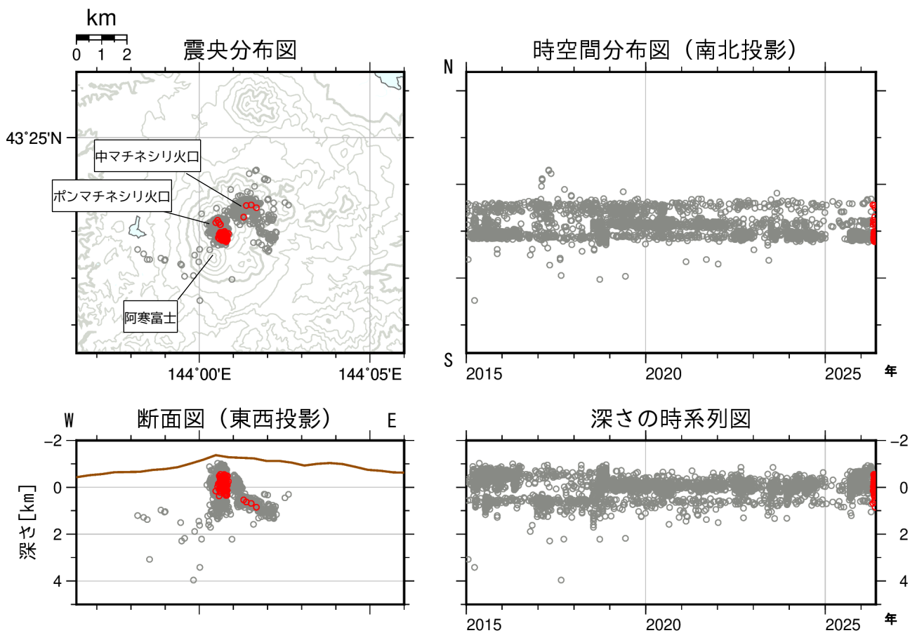
図7 雌阿寒岳 火山性地震の震源分布（2015年1月～2026年5月） ○：2015年1月～2026年4月の震源 ○：2026年5月の震源
