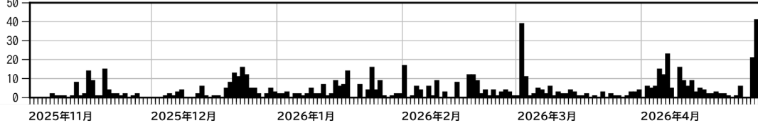
図4 樽前山 傾斜変動の推移及び火山性地震の発生状況（2025年11月～2026年4月）
