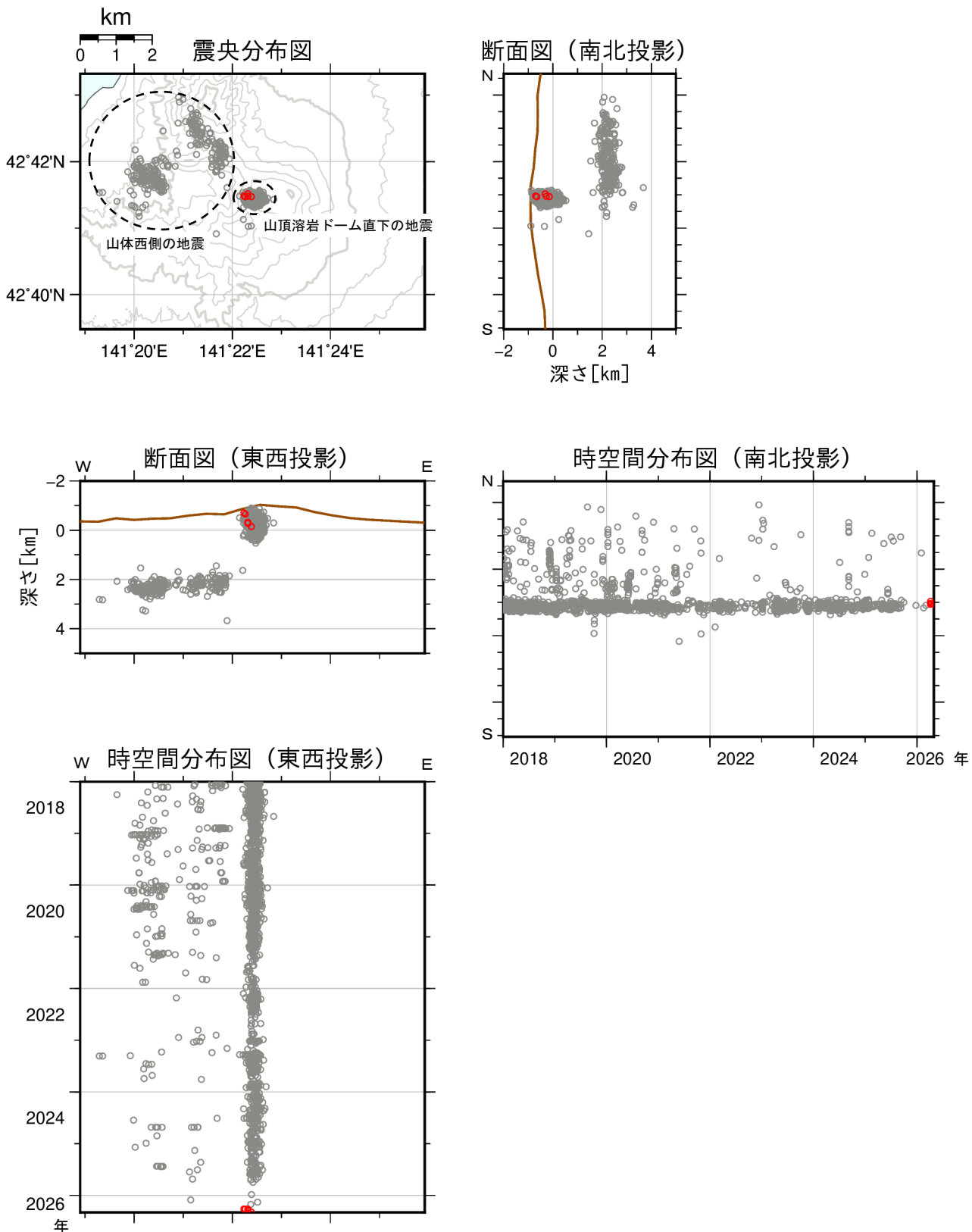
図3 樽前山 火山性地震の震源分布（2018年1月～2026年4月） ○：2018年1月～2026年3月の震源 ○：2026年4月の震源 2025年10月頃以降、一部観測点の欠測のため、震源の求まった数が減少しています。
