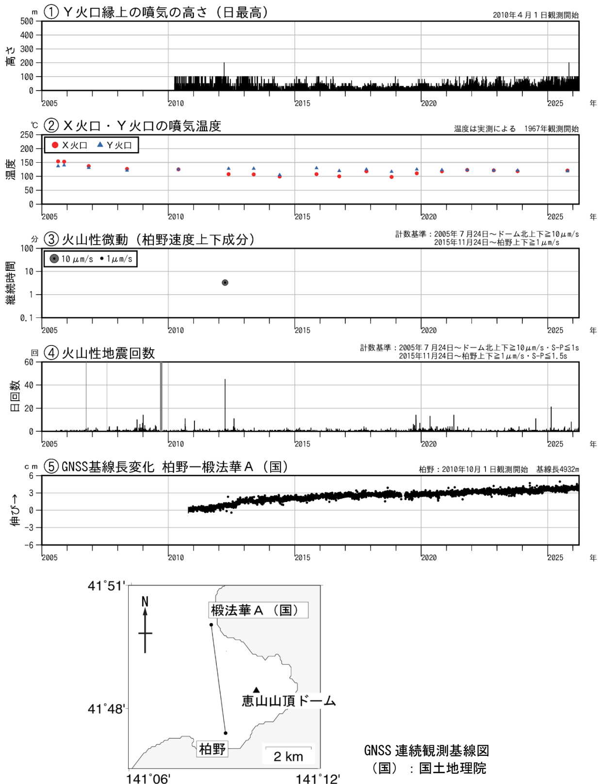
図2 恵山 火山活動経過図（2005年7月～2026年3月）
