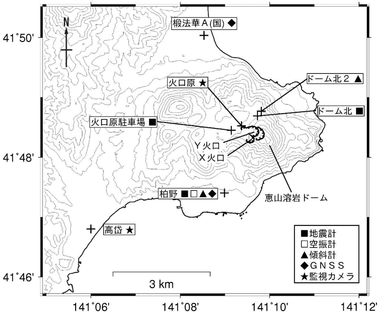
図3 恵山 観測点配置図
