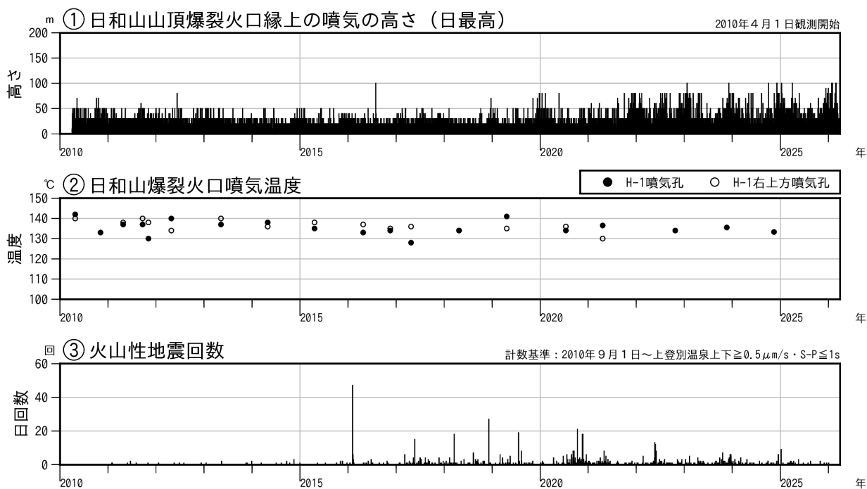
図2 倶多楽 火山活動経過図（2010年1月～2026年3月）
