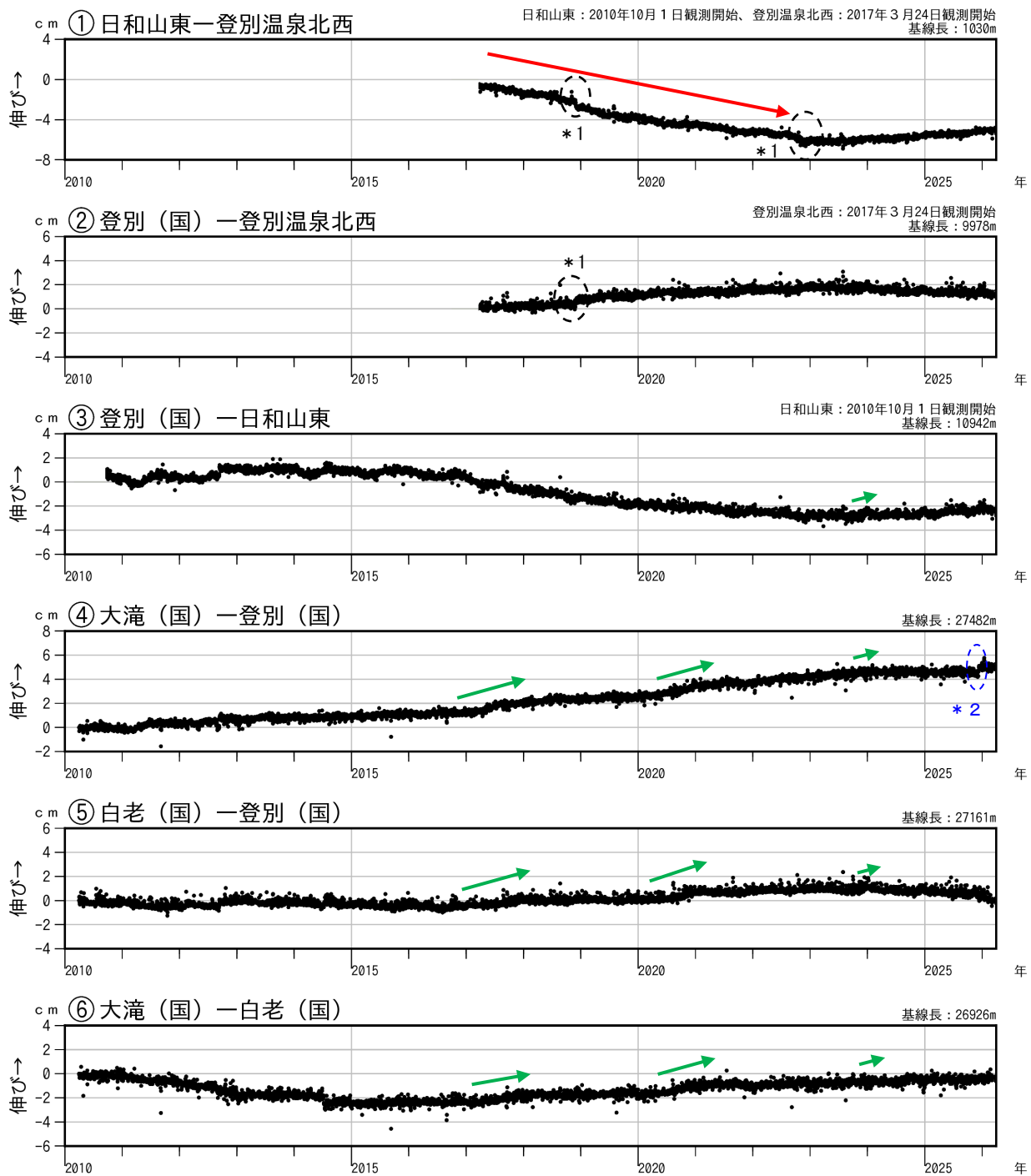
図3 倶多楽 GNSS連続観測による基線長変化（2010年4月～2026年3月）
