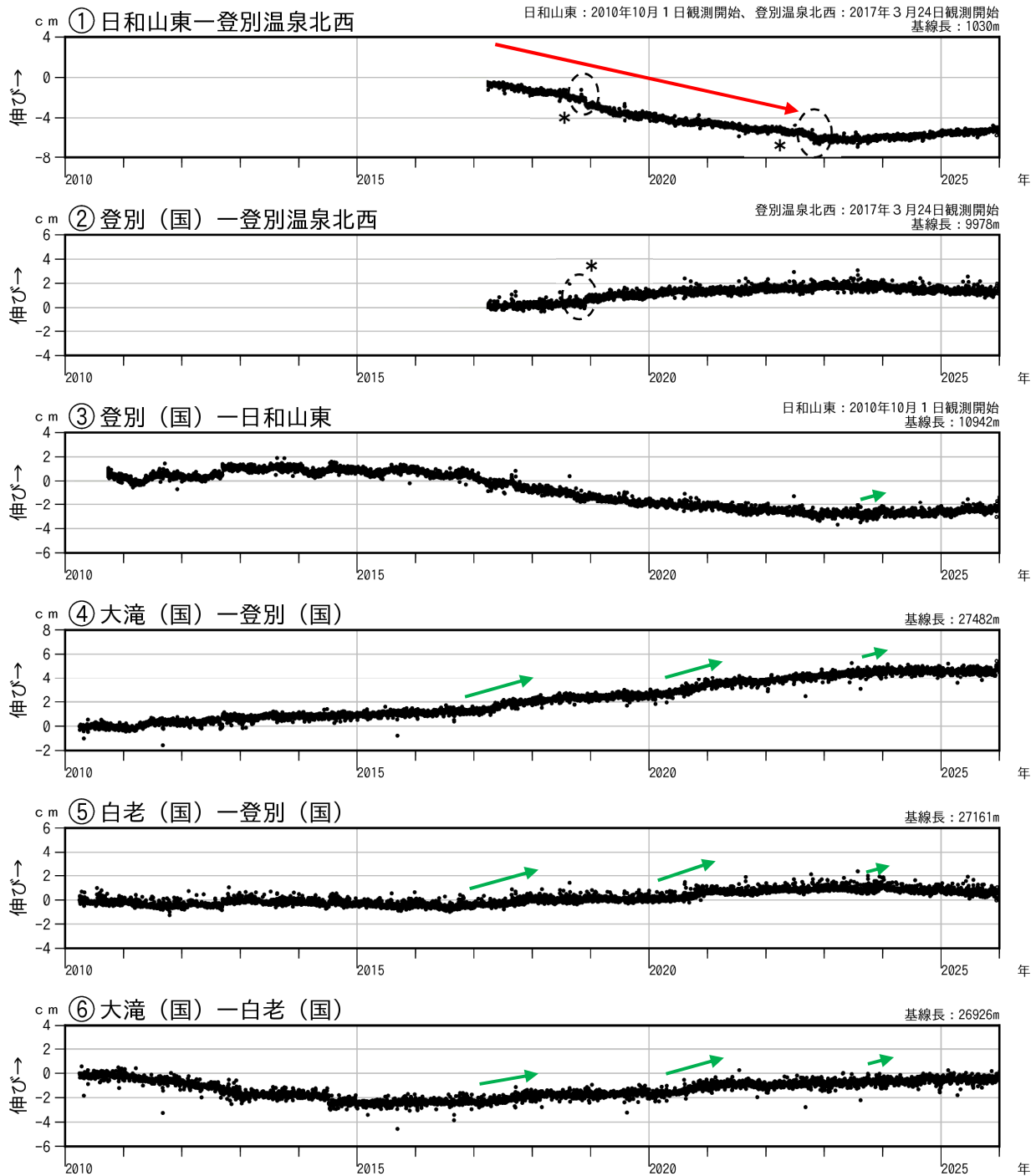
図3 倶多楽 GNSS連続観測による基線長変化（2010年4月～2025年12月）
