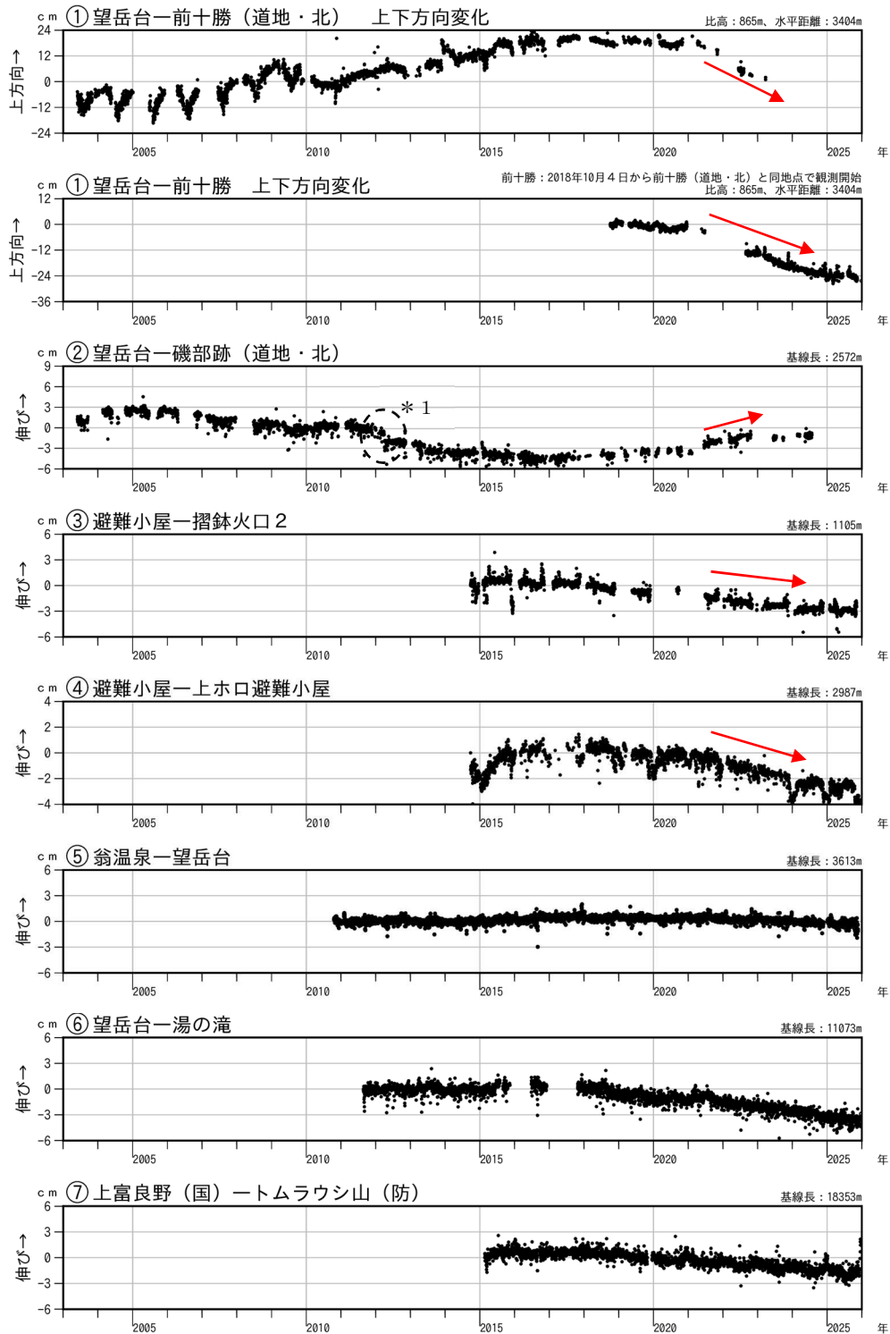
図6 十勝岳 GNSS連続観測による上下方向変化及び基線長変化（2003年5月～2025年12月）
