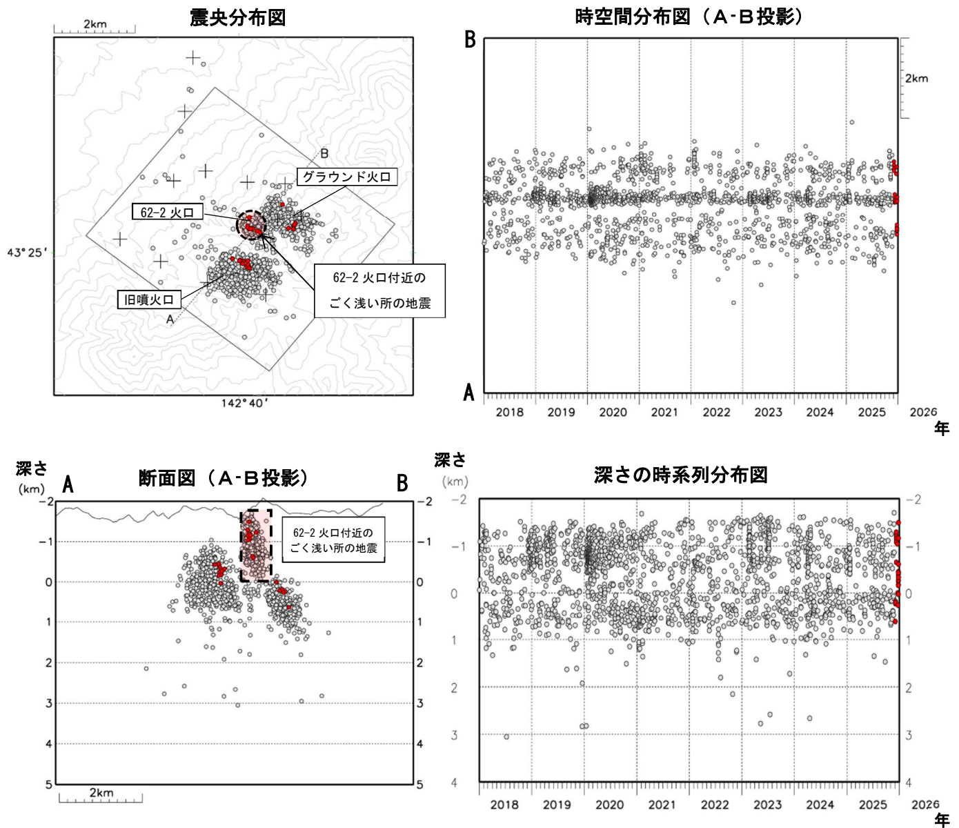
図5 十勝岳 火山性地震の震源分布（2018年1月～2025年12月）
