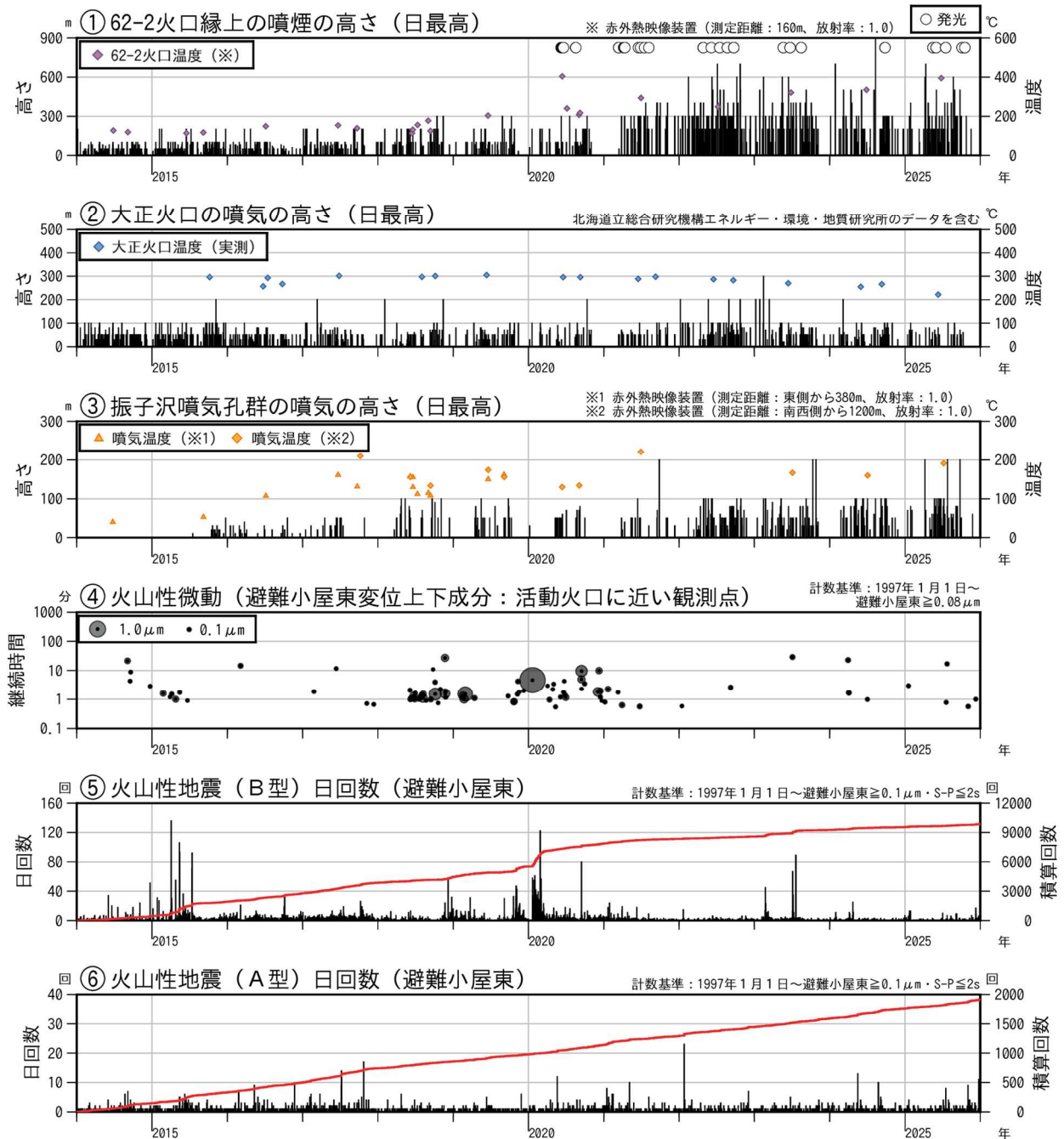
図2 十勝岳 火山活動経過図（2014年1月～2025年12月）
