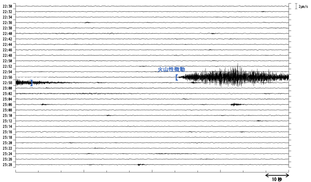
図4 十勝岳 避難小屋東の速度波形上下成分（9日22時30分～23時30分）
