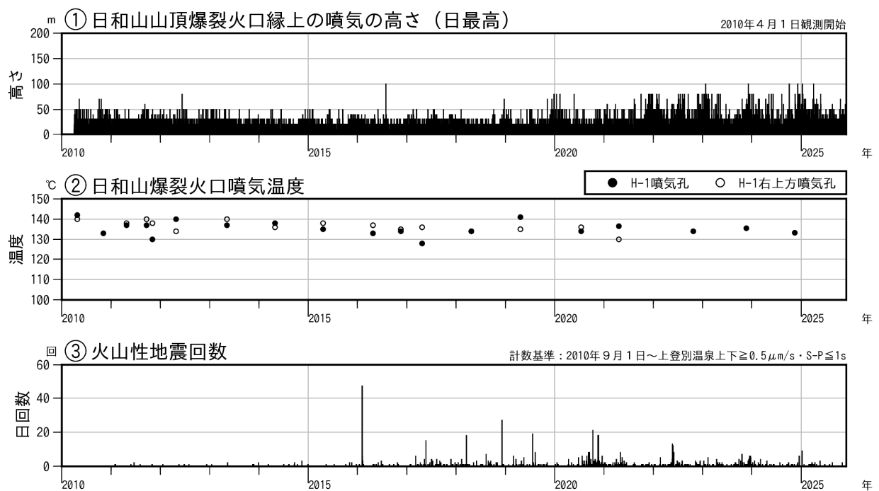
図2 倶多楽 火山活動経過図（2010年1月～2025年11月）
