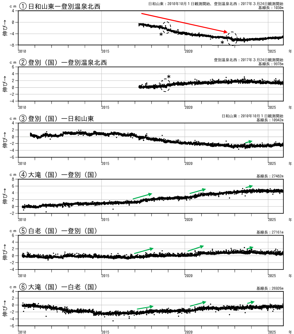
図3 倶多楽 GNSS連続観測による基線長変化（2010年4月～2025年11月）
