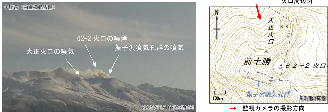
図3 十勝岳 北西側から見た火口周辺の状況（白金模範牧場監視カメラによる）及び火口周辺図
