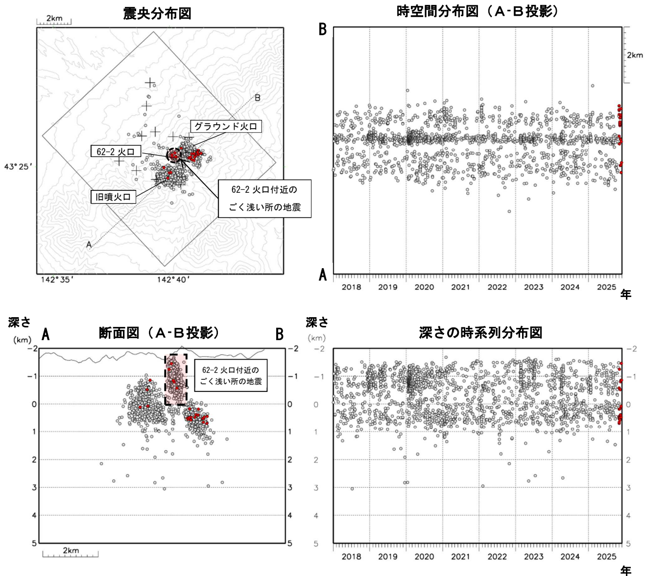
図5 十勝岳 火山性地震の震源分布（2018年1月～2025年11月）
