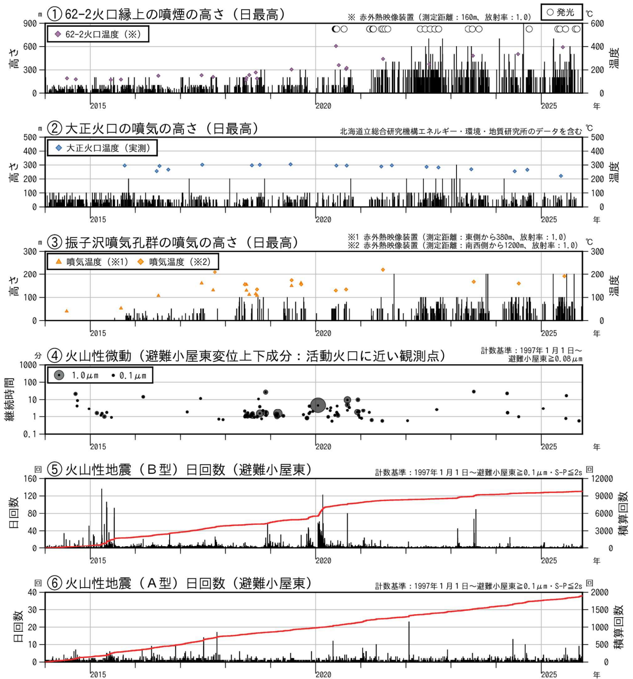
図2 十勝岳 火山活動経過図（2014年1月～2025年11月）
