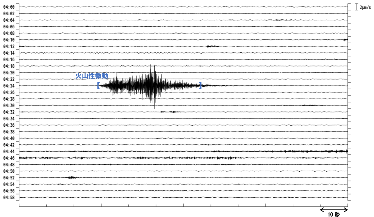
図4 十勝岳 避難小屋東の速度波形上下成分（3日04時00分～05時00分）
