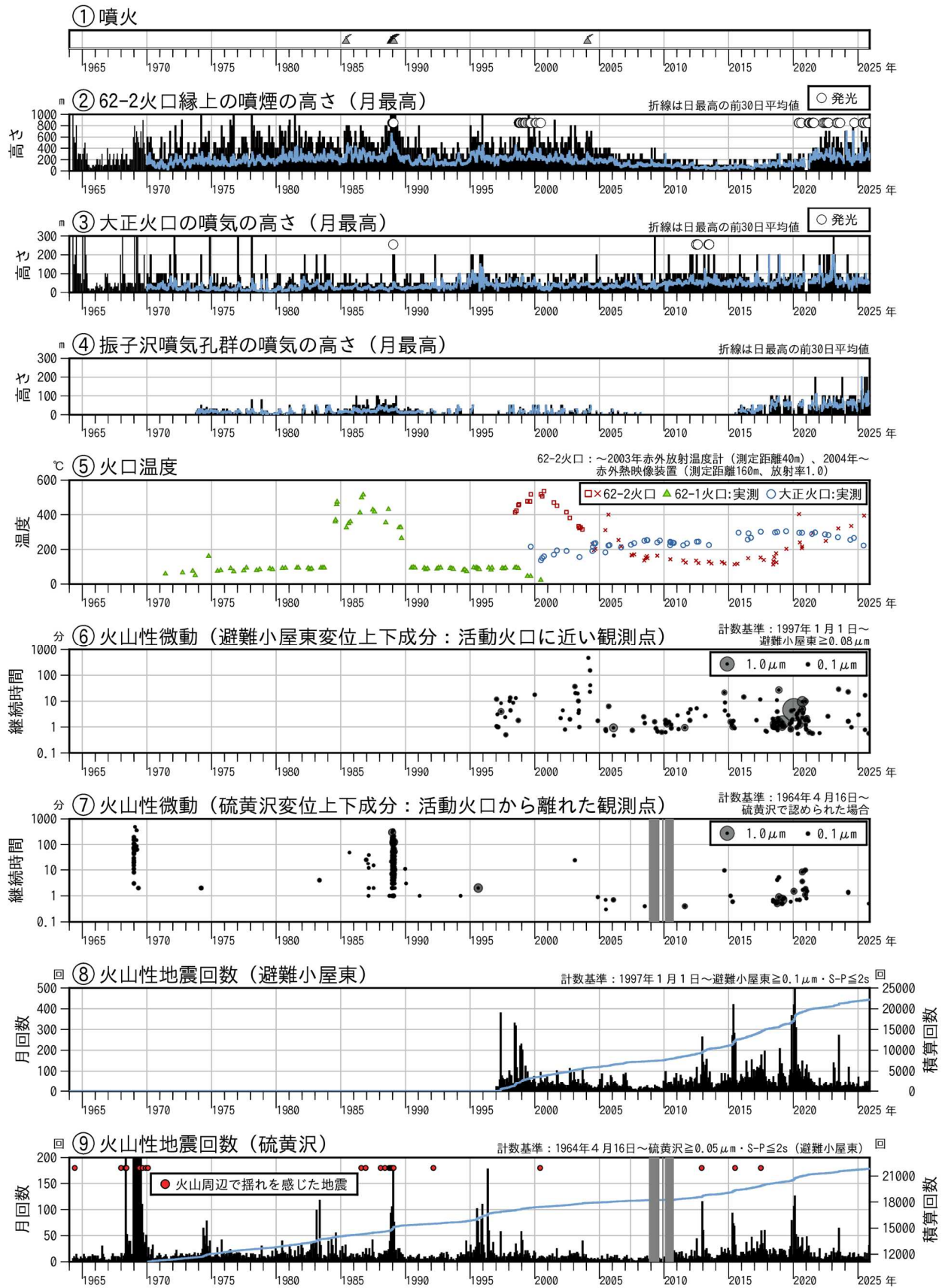
図1 十勝岳 火山活動経過図（1964年1月～2025年11月）
