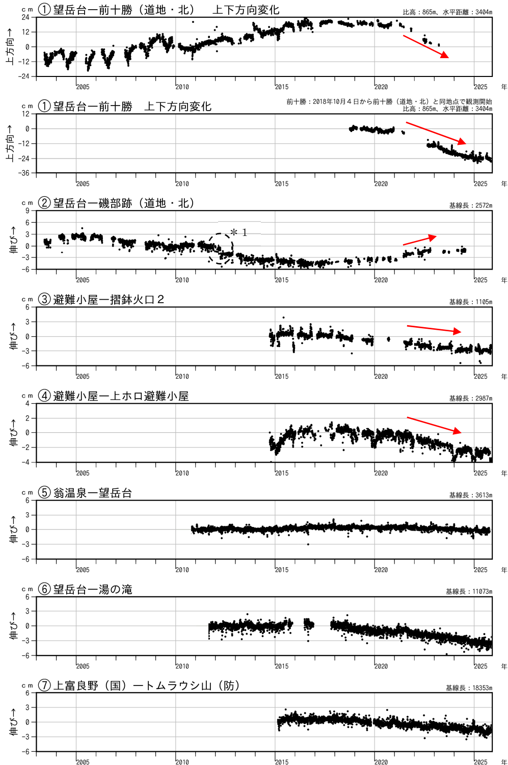
図6 十勝岳 GNSS連続観測による上下方向変化及び基線長変化（2003年5月～2025年11月）
