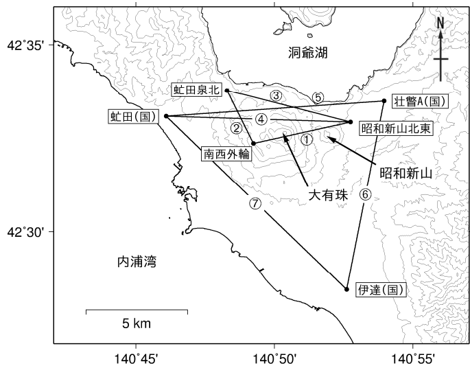
図7 有珠山 GNSS連続観測における観測点配置図
