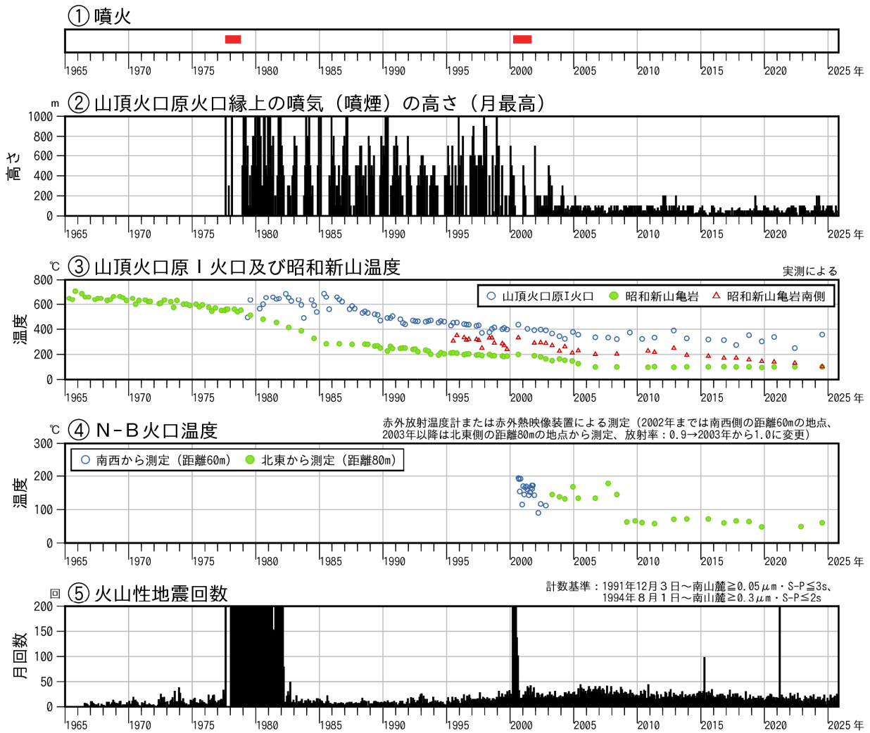
図1 有珠山 火山活動経過図（1965年1月～2025年10月）
