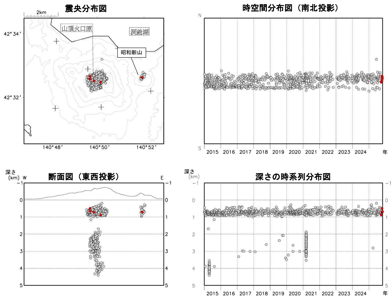
図5 有珠山 火山性地震の震源分布（2015年1月～2025年10月）
