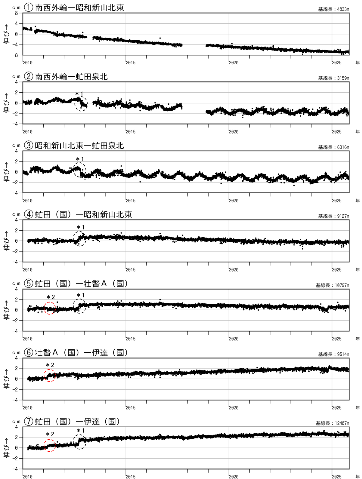
図6 有珠山 GNSS連続観測による基線長変化（2010年1月～2025年10月）
