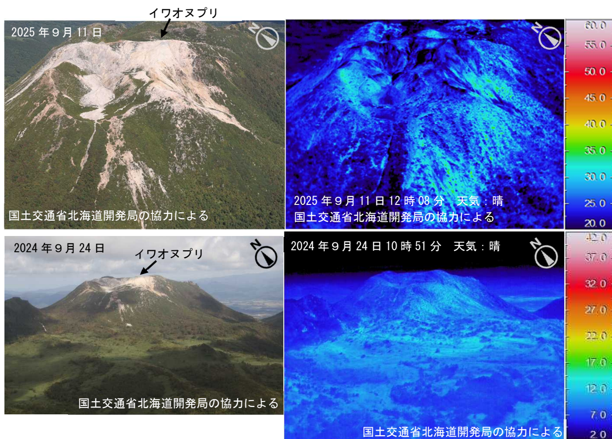
図3 ニセコ 赤外熱映像装置によるイワオヌプリ山頂部の地表面温度分布
