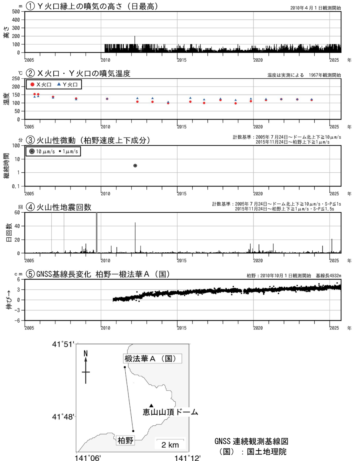
図 2 恵山 火山活動経過図（2005 年 7 月～2025 年 9 月） ④の灰色部分は機器障害による欠測期間を示します。 ⑤のグラフは上図の基線に対応しています。 ⑤のグラフの空白部分は欠測を示します。
