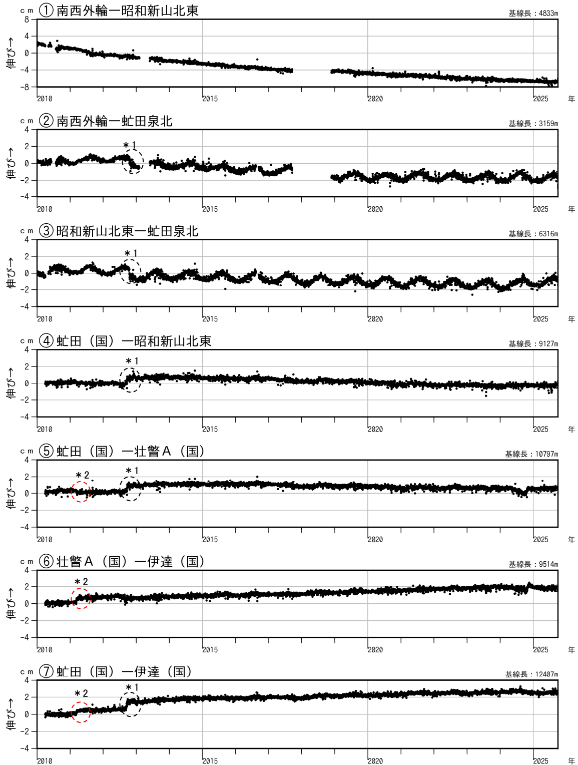
図7 有珠山 GNSS連続観測による基線長変化（2010年1月～2025年9月）
