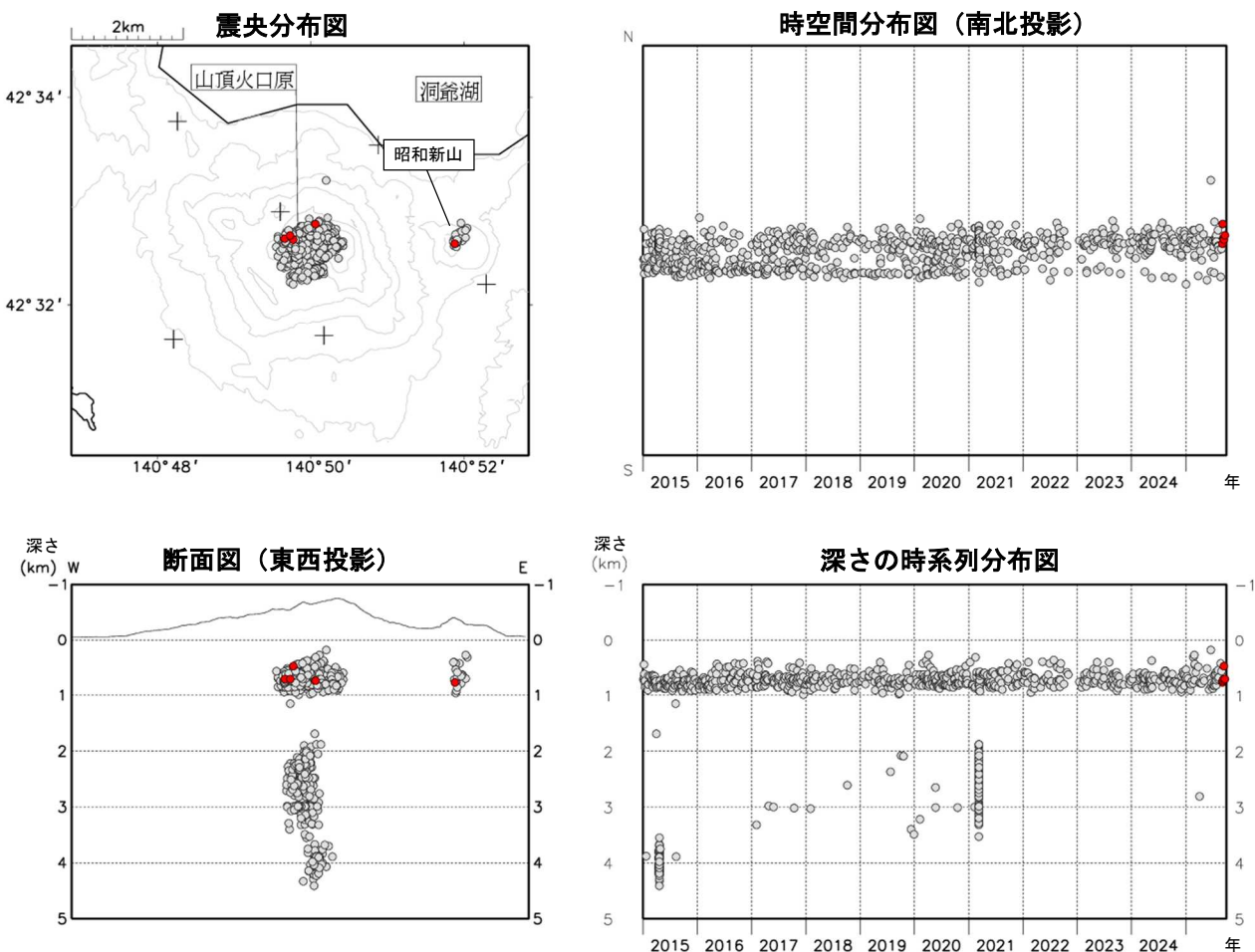
図6 有珠山 火山性地震の震源分布（2015年1月～2025年9月）
