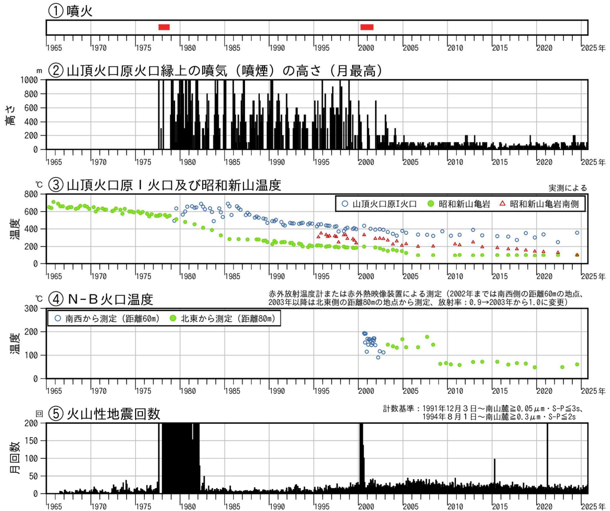
図1 有珠山 火山活動経過図（1965年1月～2025年9月）
