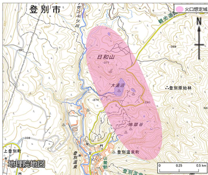
図8 倶多楽 火口想定域
