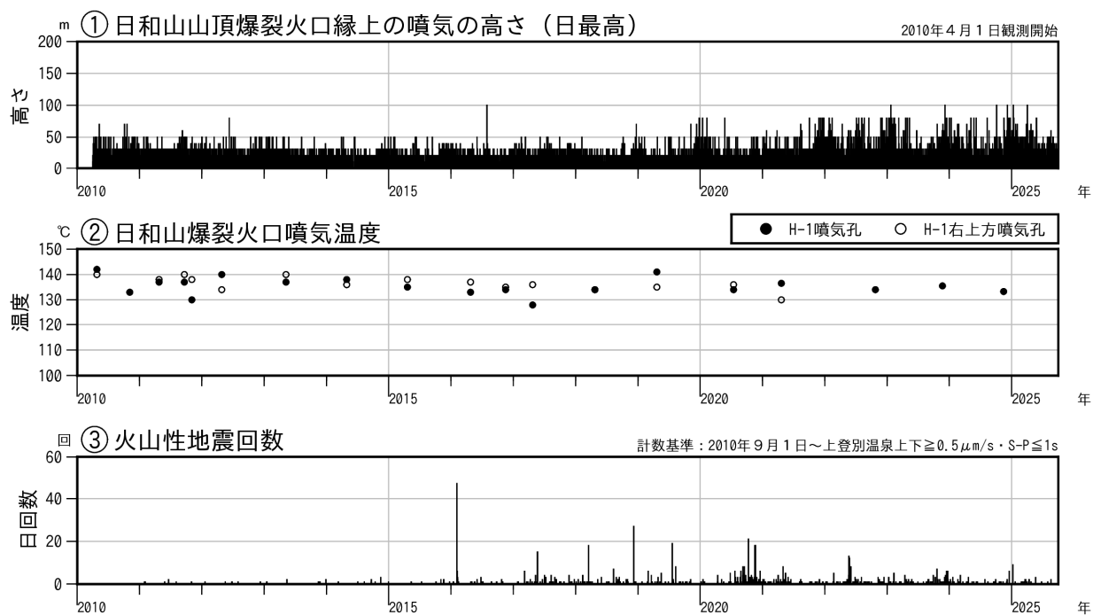
図2 倶多楽 火山活動経過図（2010年1月～2025年9月）
