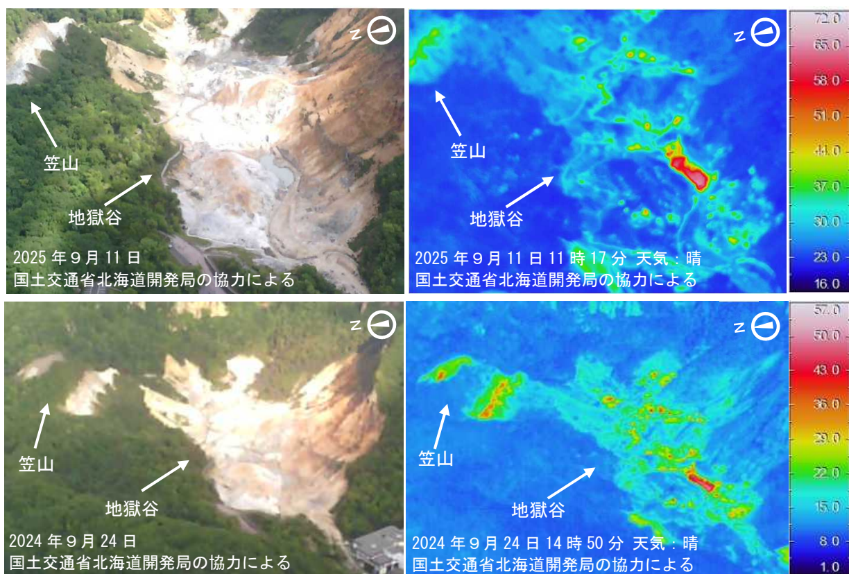
図5 倶多楽 赤外熱映像装置による地獄谷の地表面温度分布
