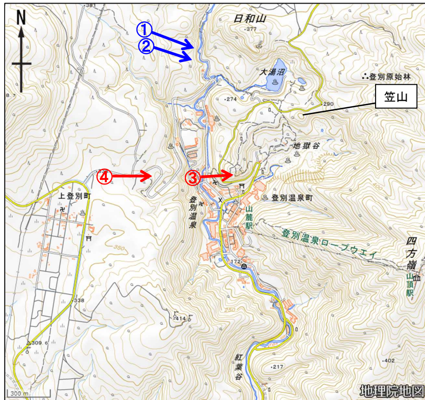
図3 赤外熱映像及び写真の撮影位置（丸数字）及び撮影方向（矢印） 青色は図4、赤色は図5に対応
