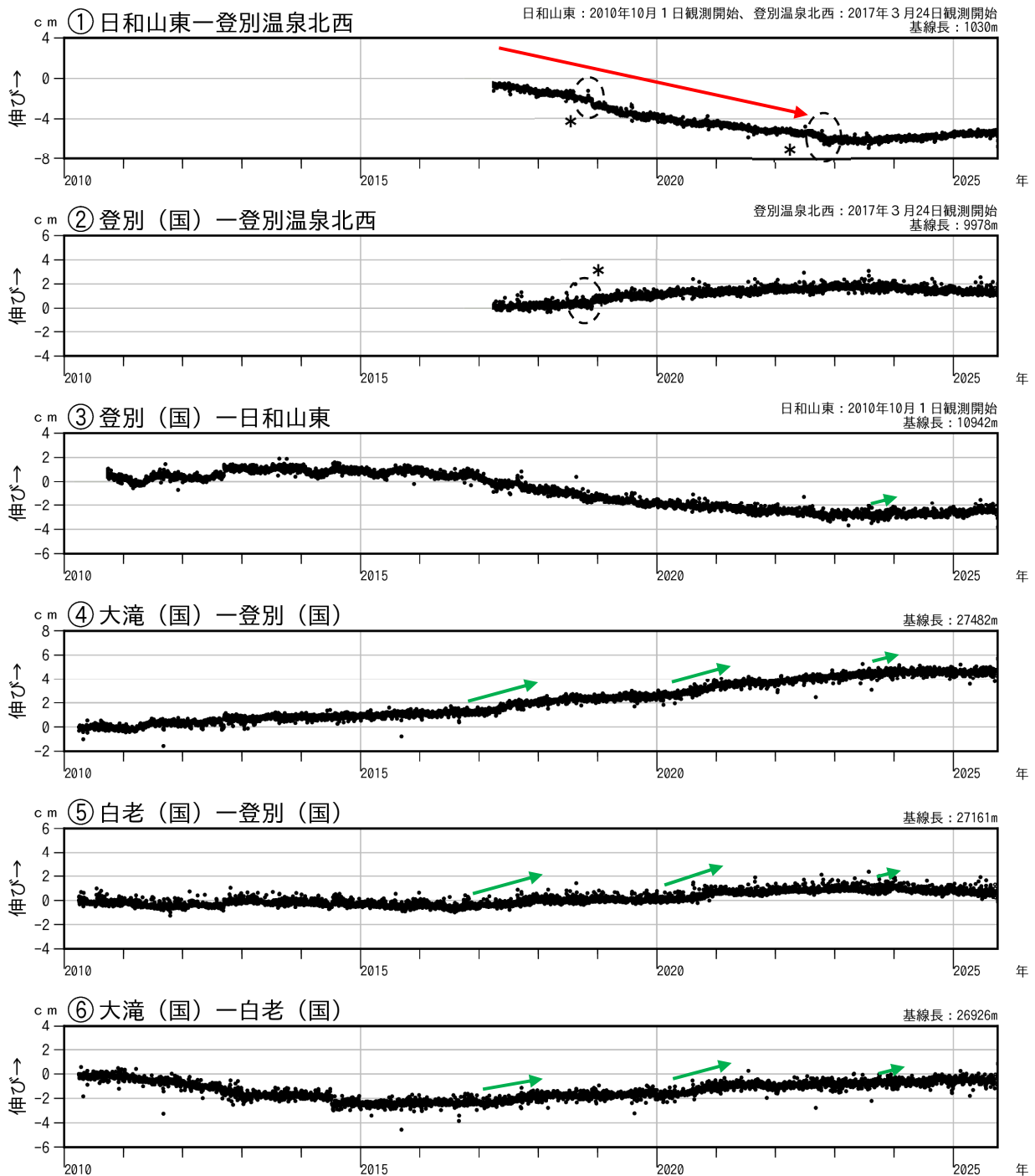
図6 倶多楽 GNSS連続観測による基線長変化（2010年4月～2025年9月）
