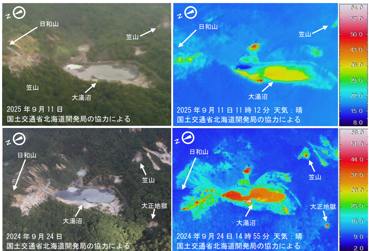
図4 倶多楽 赤外熱映像装置による日和山・大湯沼・笠山周辺の地表面温度分布 上：西側上空（図3の①）から撮影 下：西側上空（図3の②）から撮影 ・過去の観測（2024年9月）と比較して、日和山や大湯沼周辺、笠山の地表面温度分布に特段の変化は認められませんでした。
